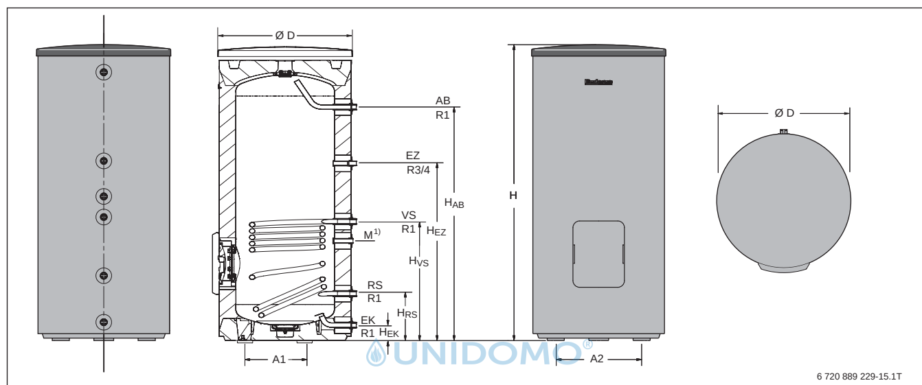
Bild 16 Abmessungen der stehenden Warmwasserspeicher Logalux ESU160 ... ESU300 (Maße in mm)
