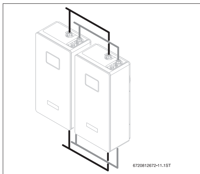
Bild 57 Beispiel: FS80/3 E mit Verrohrungsset
