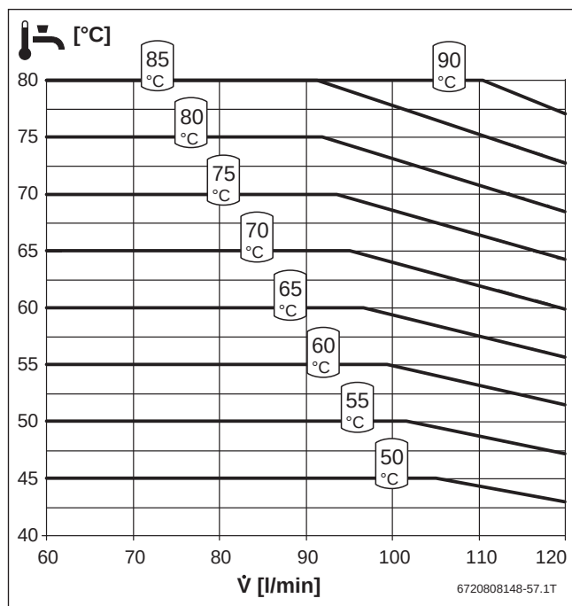
Bild 54 Temperaturverhalten Kaskade FS120/3 E
