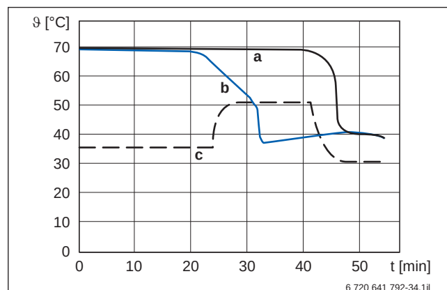
Bild 25 Vergleich des Temperaturverlaufes im Speicher oben
