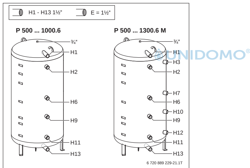
Bild 30 Aufbau und Anschlüsse Pufferspeicher Logalux P...6 (M)
