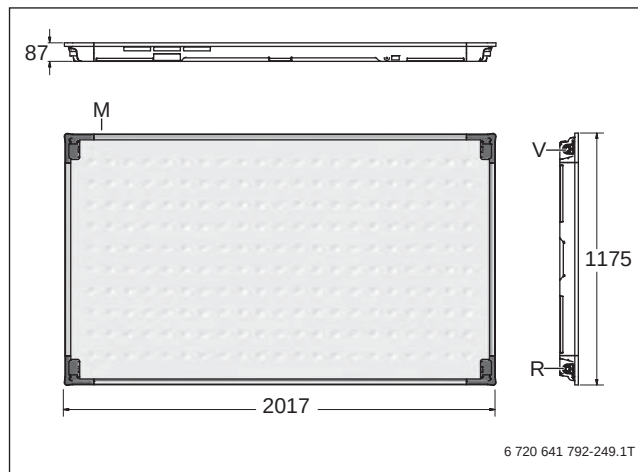
Bild 6 Abmessungen Logasol SKN4.0-w (waagerecht); Maße in mm
