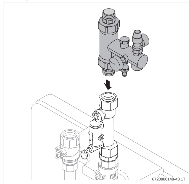
Bild 81 Sicherheitsgruppe montieren
