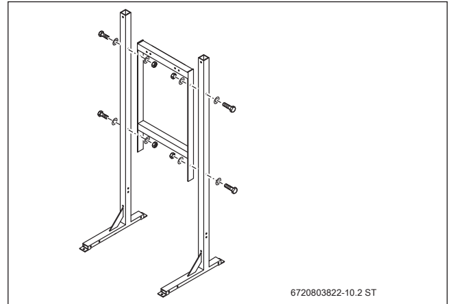
Bild 72 Montageständer
