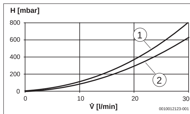
Bild 181 Druckverlust Sekundärseite
