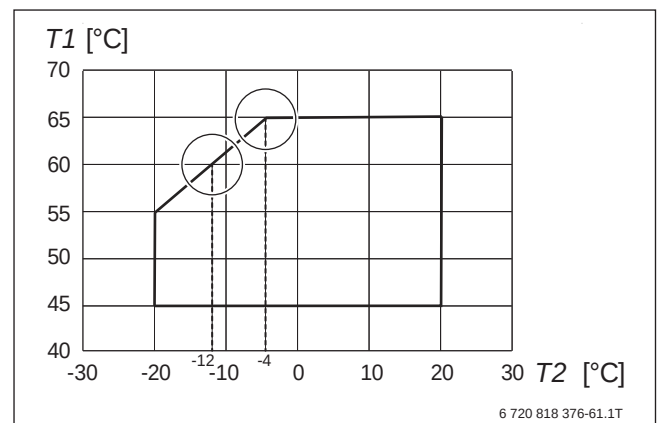
Bild 163 Ein- und Ausschaltemperatur WLW196i..IR/AR
