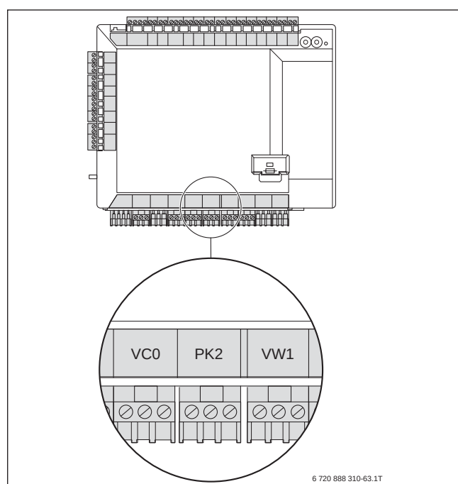
Bild 3 Anschluss Wechselkontakt
