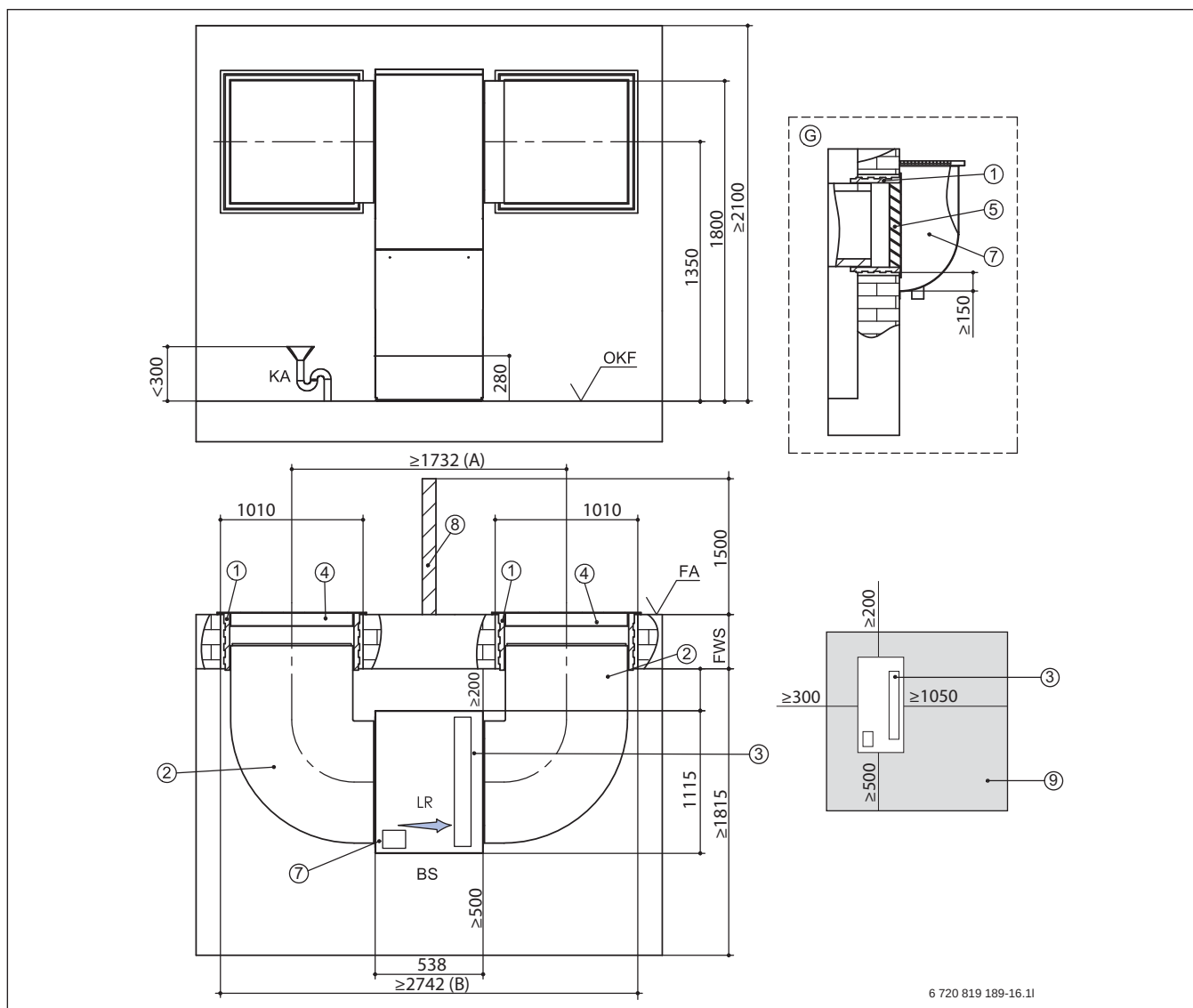
Bild 24 Kanalpläne für Luftkanalsystem für WLW196i-11 IR und WLW196i-14 IR (Maße in mm)
