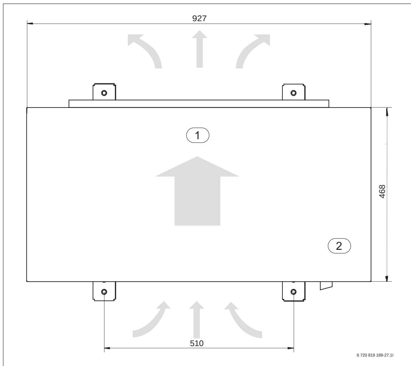
Bild 56 Abmessungen IDUWP6 und IDUWP8, Draufsicht (Maße in mm)
