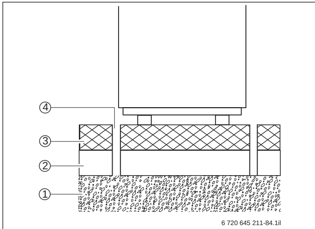
Bild 14 Estrich aussparen
