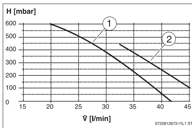
Bild 183 Restförderhöhe Primärseite
