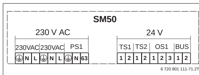
Bild 148 Anschlussklemmen des Solarmoduls SM50
