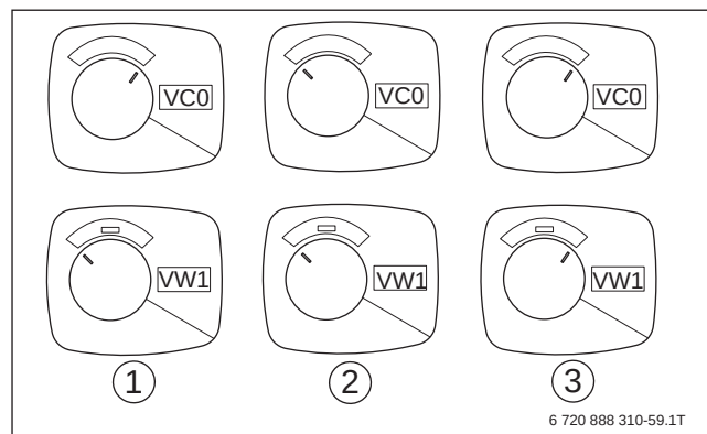
Bild 197 Einstellungen Stellmotoren (Hydraulikbox)
