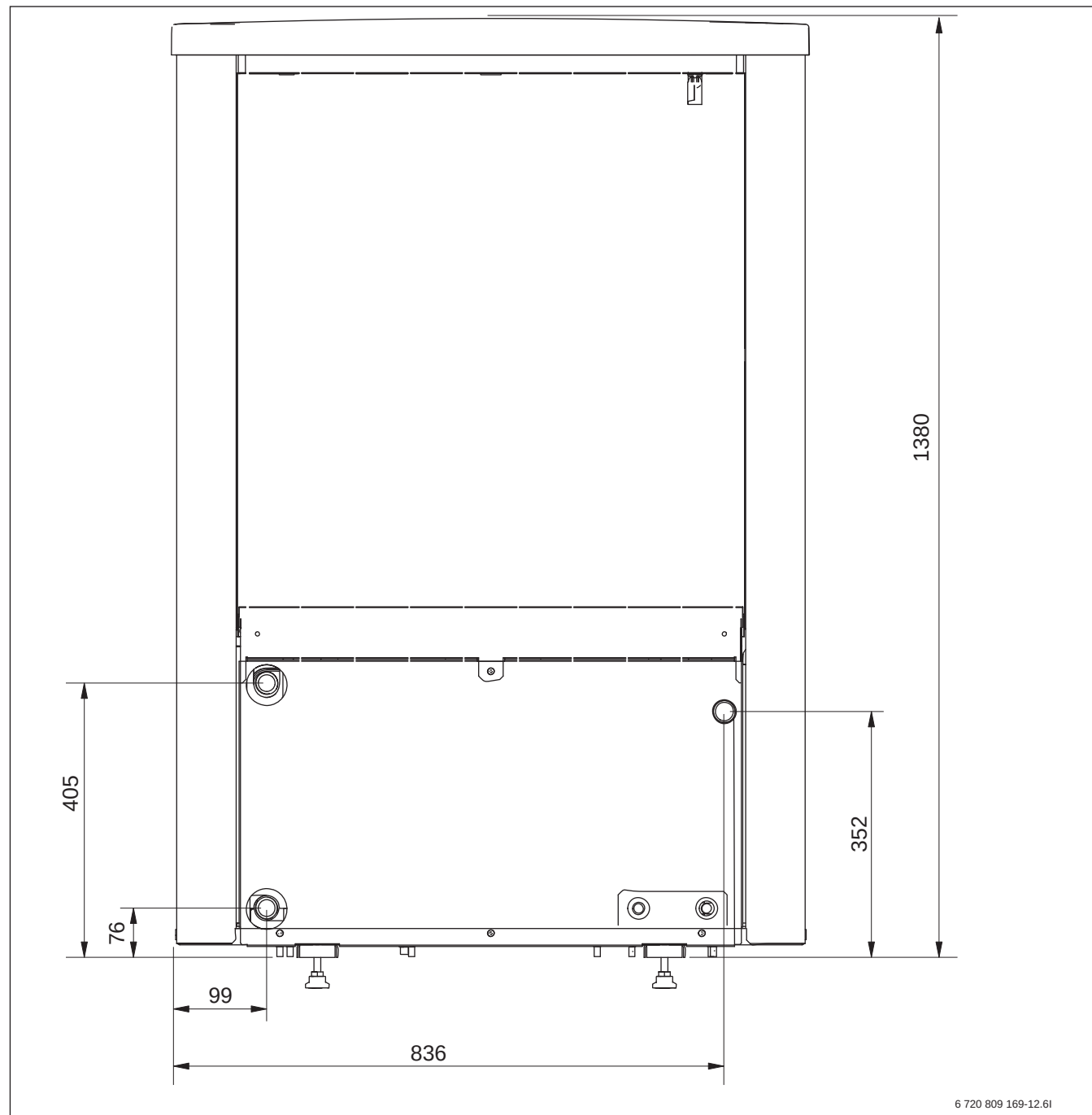
Bild 61 Abmessungen der Außeneinheit ODU4.2i ... ODU8.2i, Rückseite
