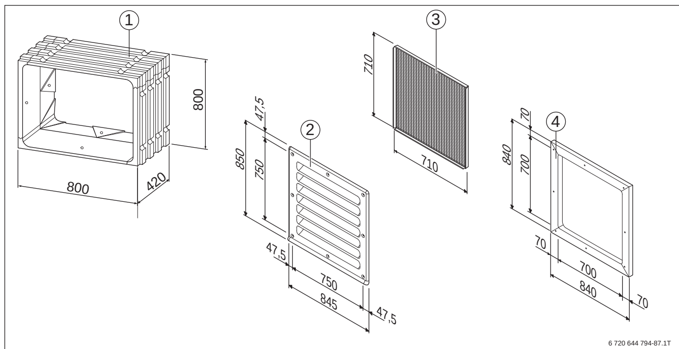
Bild 16 Wanddurchführung, Wetter-/Regenschutzgitter, Maschendrahtgitter und Verblendraahmen des Systems Luftkanal (Maße in mm)
