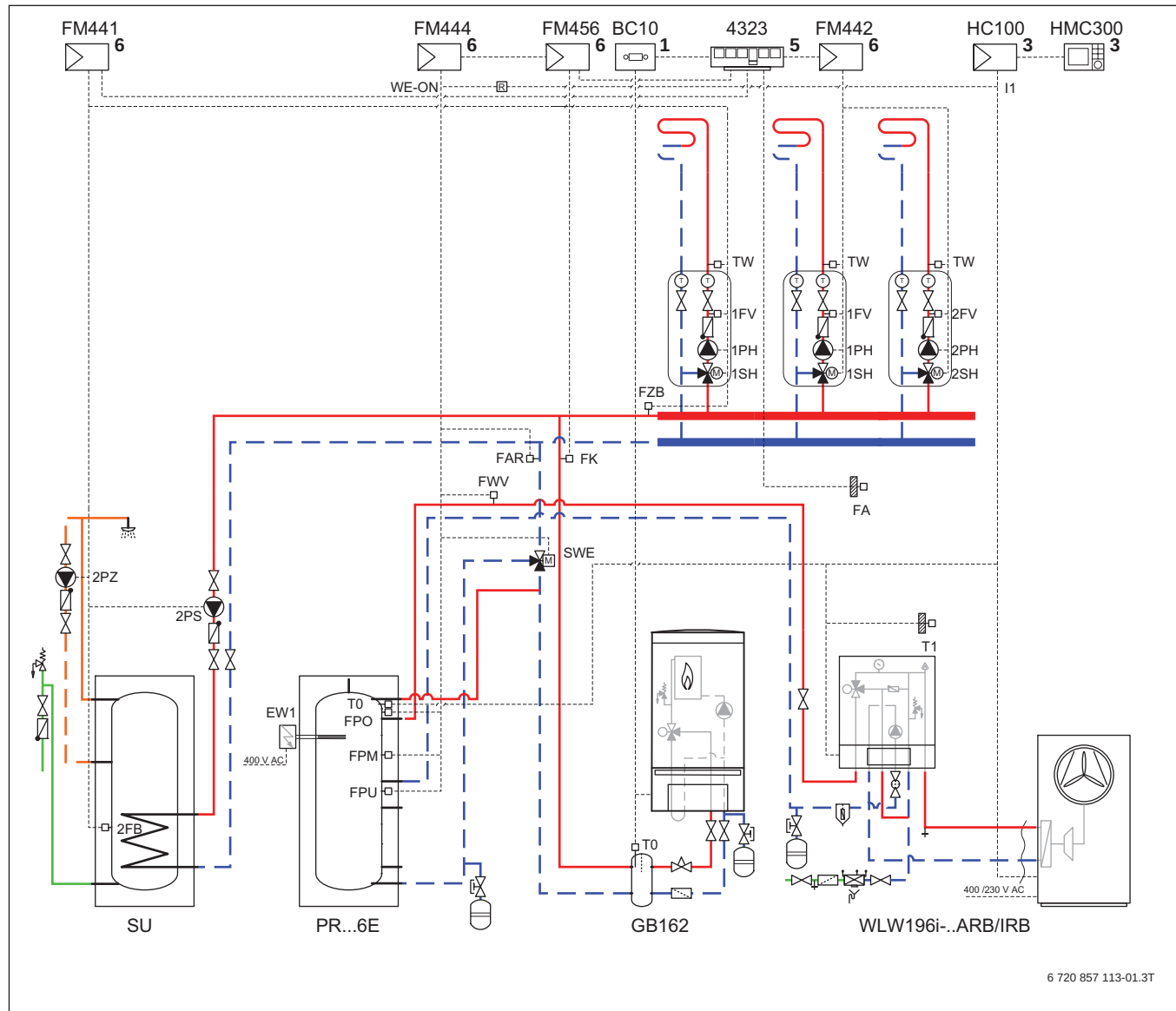
Bild 255 Anlagenschema mit Regelung (unverbindliche Prinzipdarstellung)
