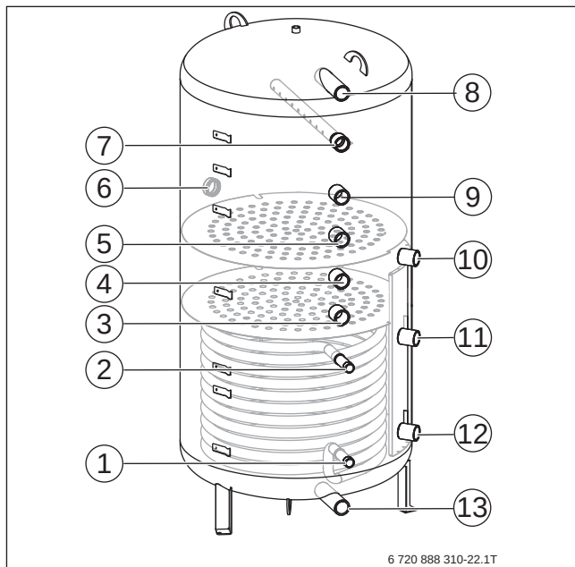
Bild 249 PNRZ-Speicher anschließen
