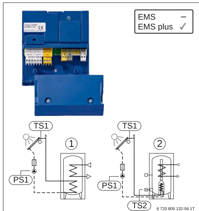
Bild 147 Solarmodul SM50
