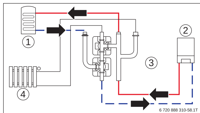
Bild 196 Hydraulik Warmwasserkreis
