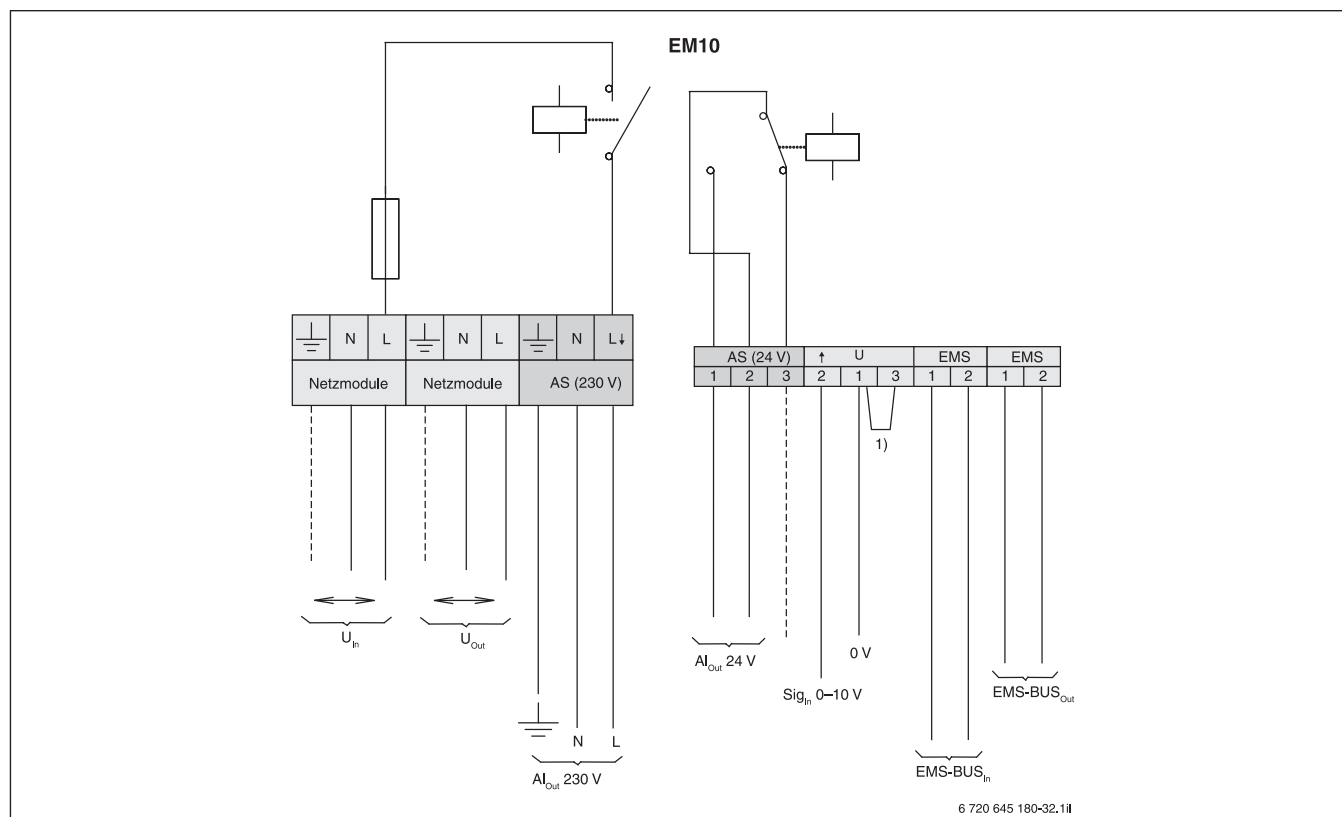
Bild 156 Anschlussplan des Störmeldemoduls EM10
