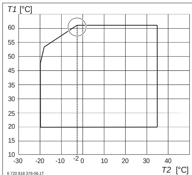
Bild 162 Ein- und Ausschaltemperatur WLW196i..IR/AR
