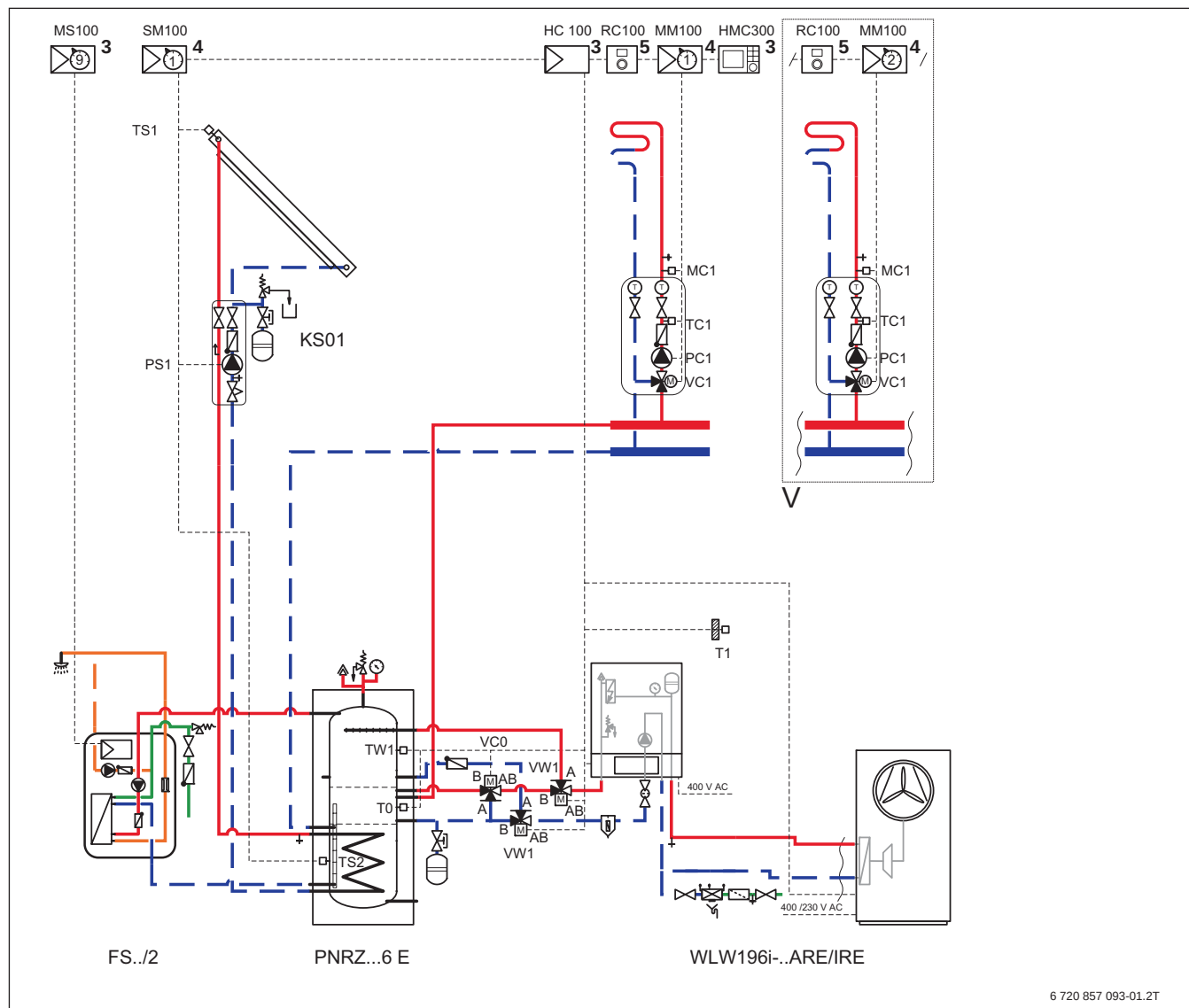
Bild 235 Anlagenschema mit Regelung (unverbindliche Prinzipdarstellung)
