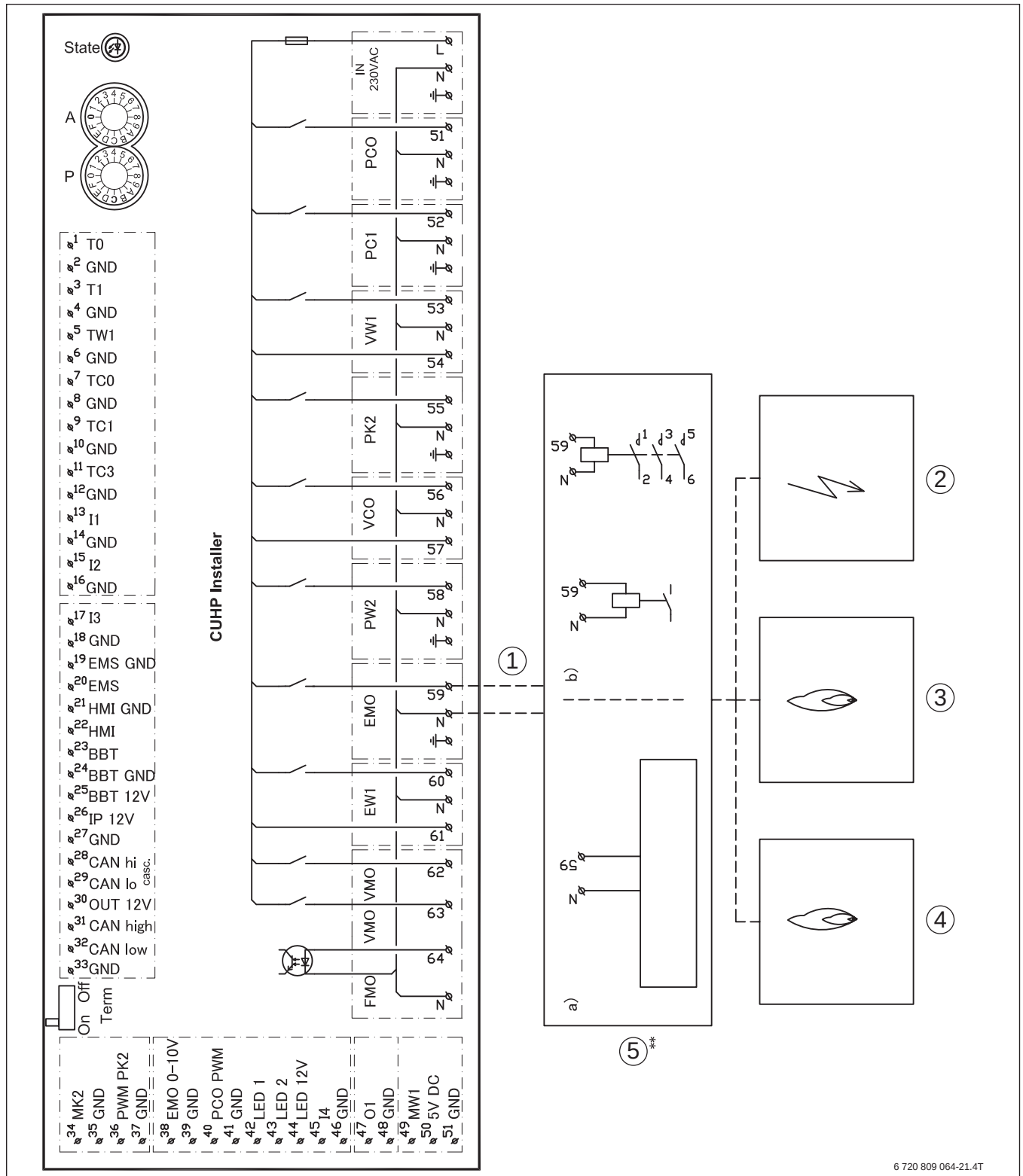
Bild 127 Schaltplan Installationsmodul, Start/Stopp
