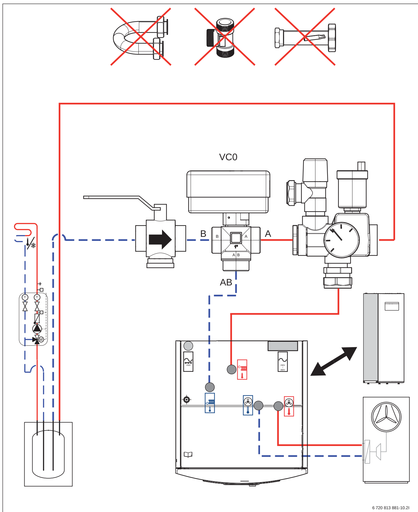
Bild 205 Umrüstung Tower
