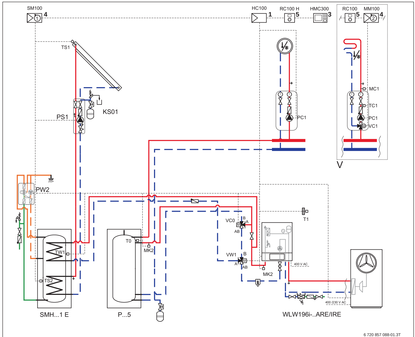
Bild 234 Anlagenschema mit Regelung (unverbindliche Prinzipdarstellung)
