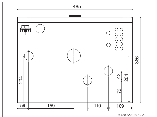
Bild 71 Abmessungen IDU-8/14 iE (Ansicht von unten; Maße in mm)
