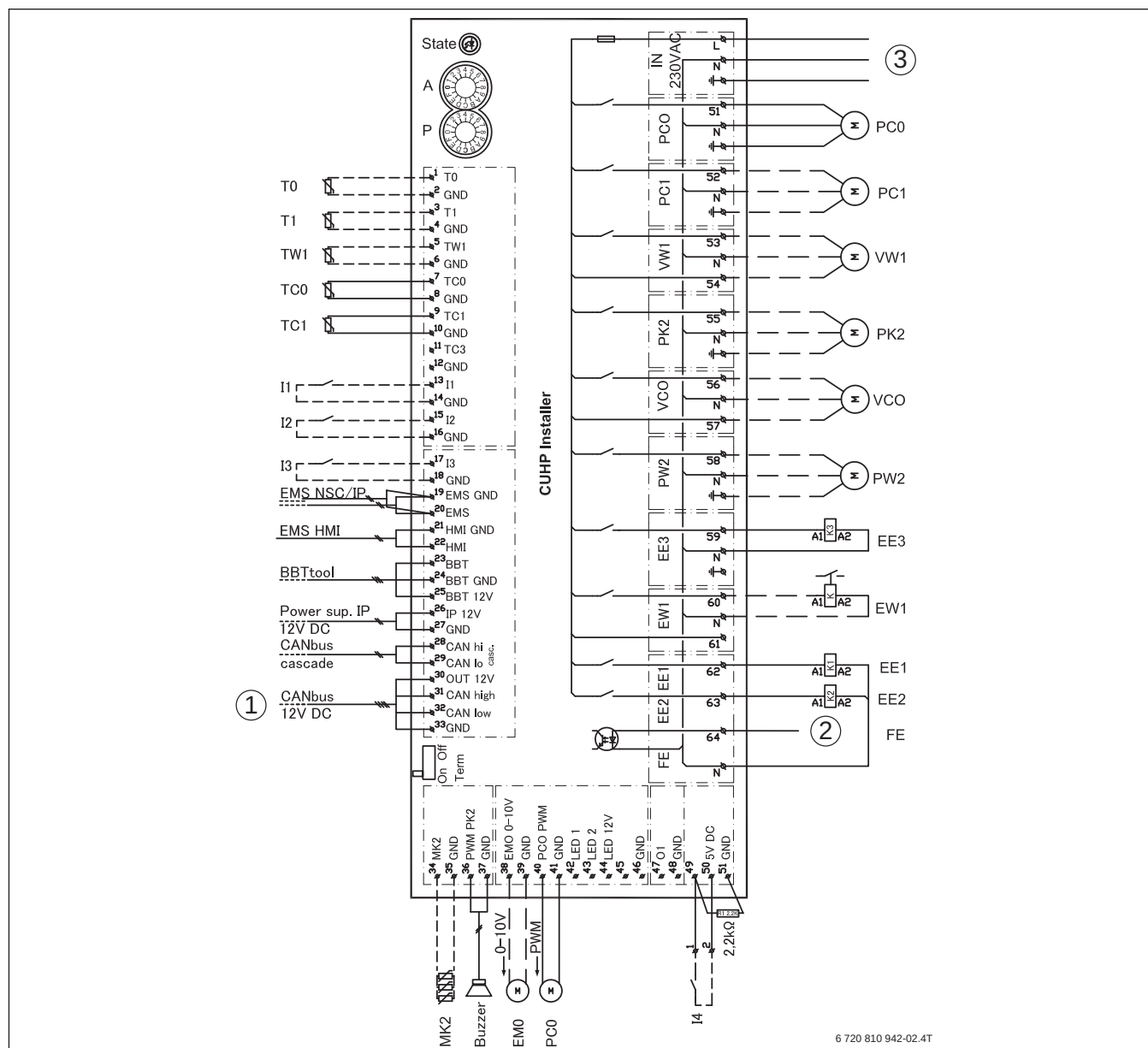
Bild 132 Schaltplan Installationsmodul
