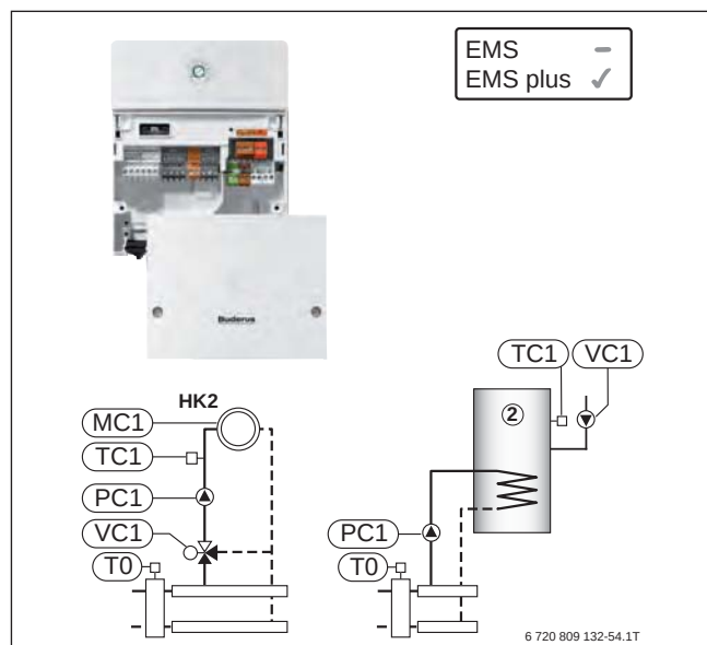
Bild 145 Heizkreismodul MM100
