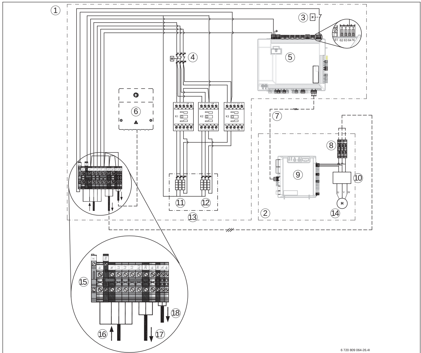
Bild 121 1-phasige Wärmepumpe WLW196i-4 AR, WLW196i-6 IR/AR und WLW196i-8 IR/AR und 3-phasiger integrierter elektrischer Zuheizer
