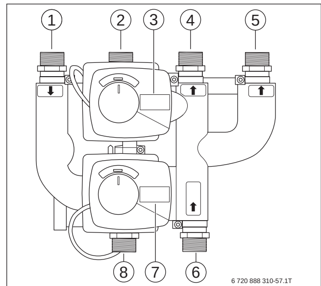
Bild 193 Hydraulik-Box VC0-VW1
