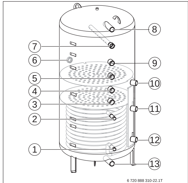
Bild 239 PNRZ-Speicher anschließen
