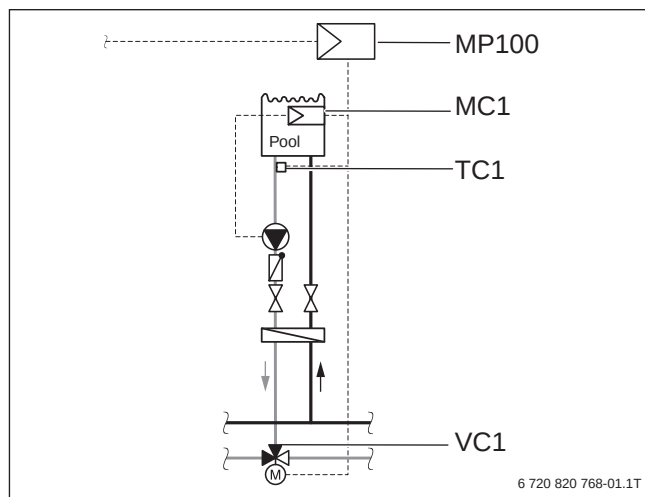
Bild 10 Beispieldarstellung für eine Schwimmbadanlage
