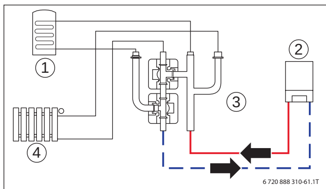
Bild 195 Hydraulik Kurzschlusskreis
