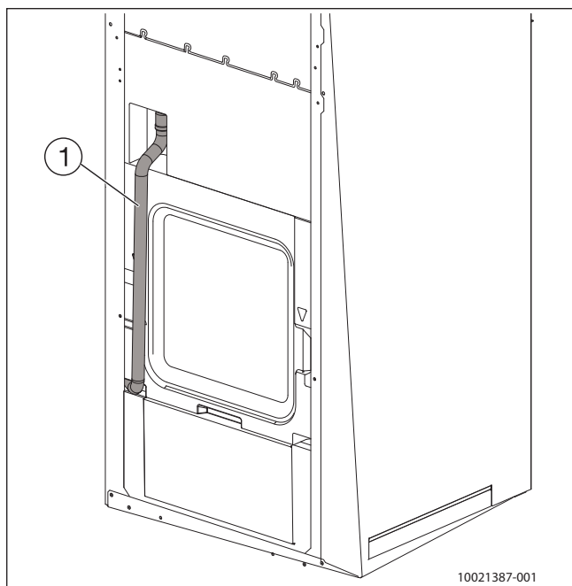
Bild 91 Rückansicht Ablaufschlauch
