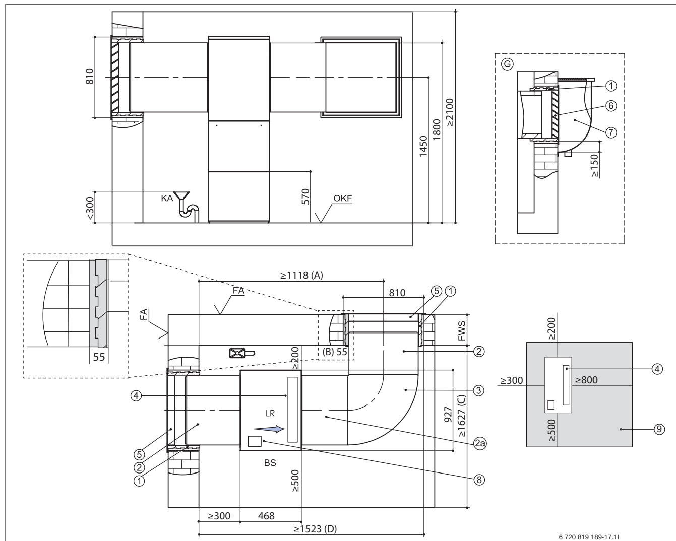
Bild 19 Kanalpläne für Luftkanalsystem für WLW196i-6 IR und WLW196i-8 IR (Maße in mm)
