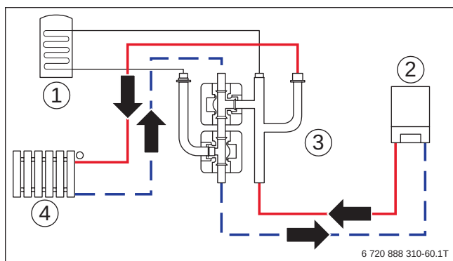
Bild 194 Hydraulik Pufferkreis
