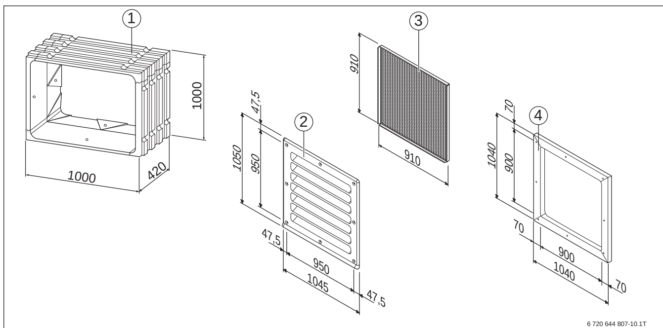
Bild 18 Wanddurchführung, Wetter-/Regenschutzgitter, Maschendrahtgitter und Verblendraahmen des Systems Luftkanal (Maße in mm)
