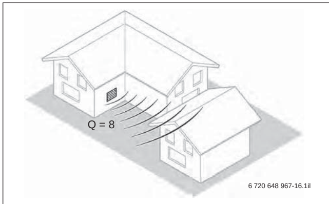
Bild 39 Wärmepumpe oder Lufteinlass/Luftauslass (bei Innenaufstellung) an einer Hauswand bei ein-springender Fassadenecke, Abstrahlung in den Achtelraum ( Q = 8 ); Bildquelle: „Leitfaden Schall“ des bwp e.V
