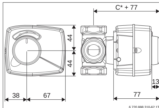
Bild 200 Abmessungen Mischermotor
