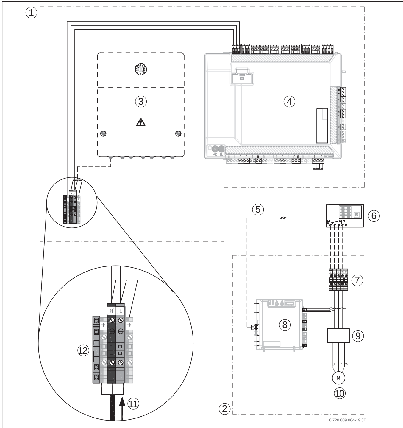
Bild 124 Inneneinheit mit externem Zuheiz – Überblick
