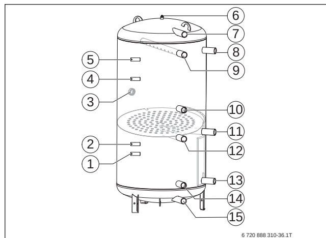
Bild 242 PRZ-Speicher anschließen
