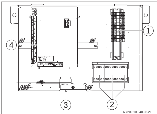
Bild 95 Klemmenkastenordnung
