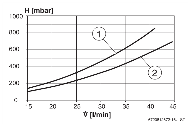
Bild 184 Druckverlust Sekundärseite
