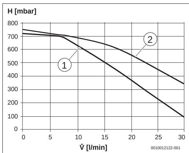
Bild 180 Restförderhöhe Primärkreispumpe
