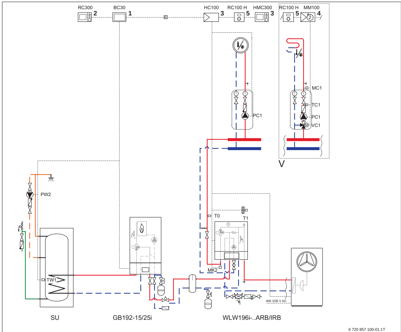
Bild 246 Anlagenschema mit Regelung (unverbindliche Prinzipsdarstellung)
