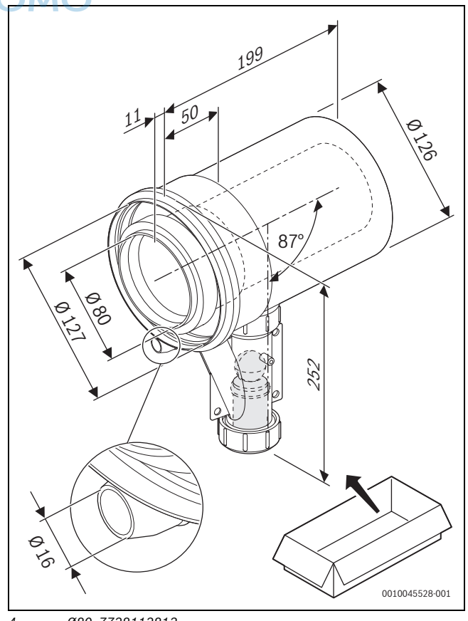
4 Ø80: 7738113813
