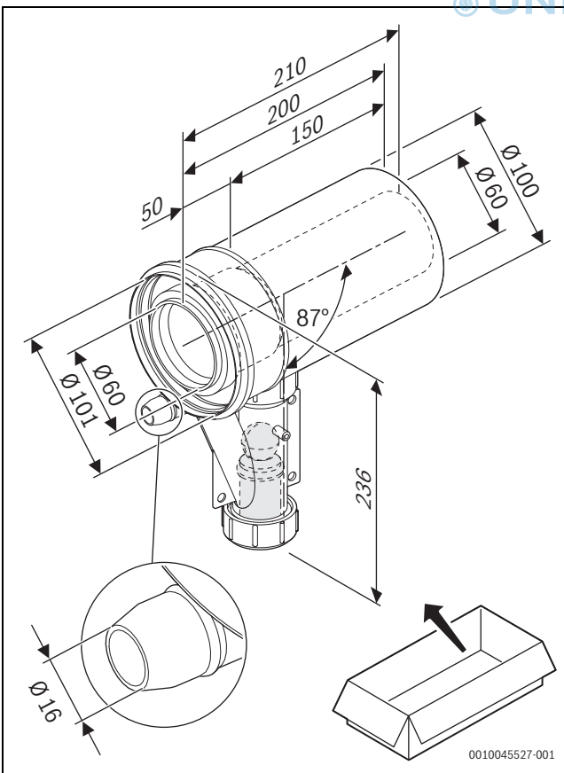
3 Ø60: 7738113814
