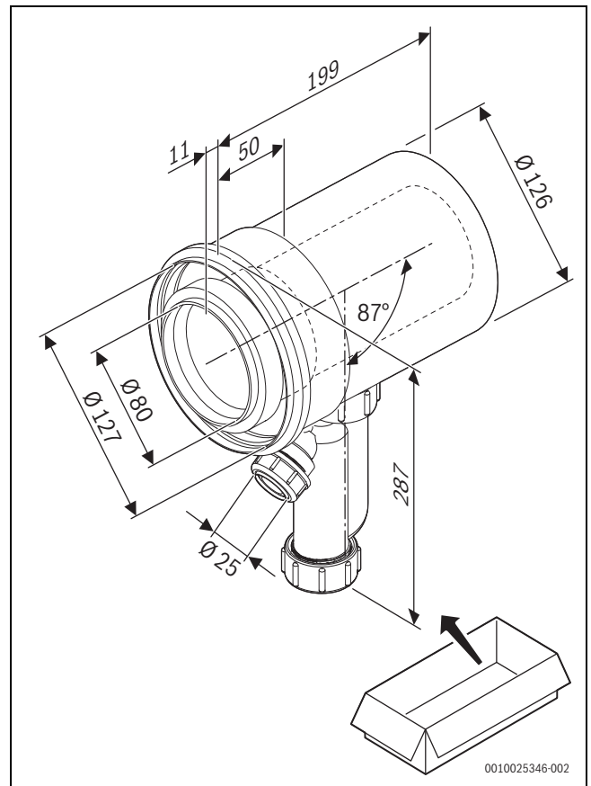
2 Ø80: 7738112768
