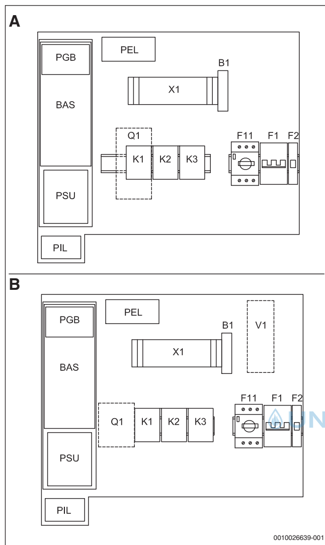
Bild 12 Leiterplatten WPS 6-1...17-1
