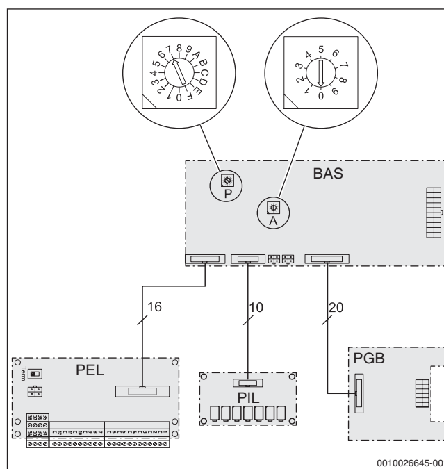
Bild 13 Elektrische Verbindung der Leiterplatten der WPS ..-1
