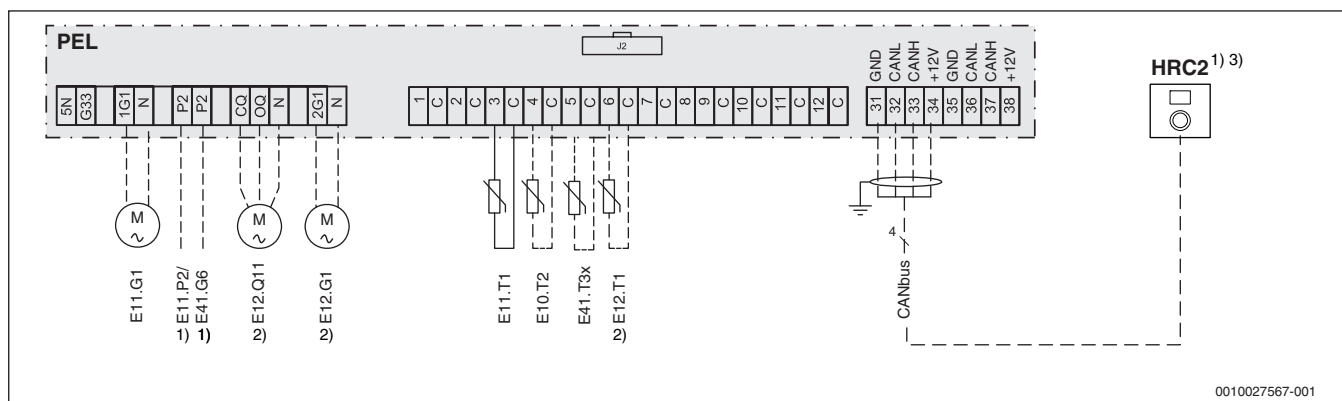
Bild 9 Schaltplan zum Anlagenbeispiel
