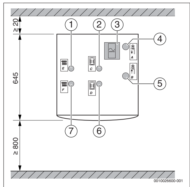
Bild 5 Abmessungen und Mindestabstände WPS 6-1...8-1 (Draufsicht)
