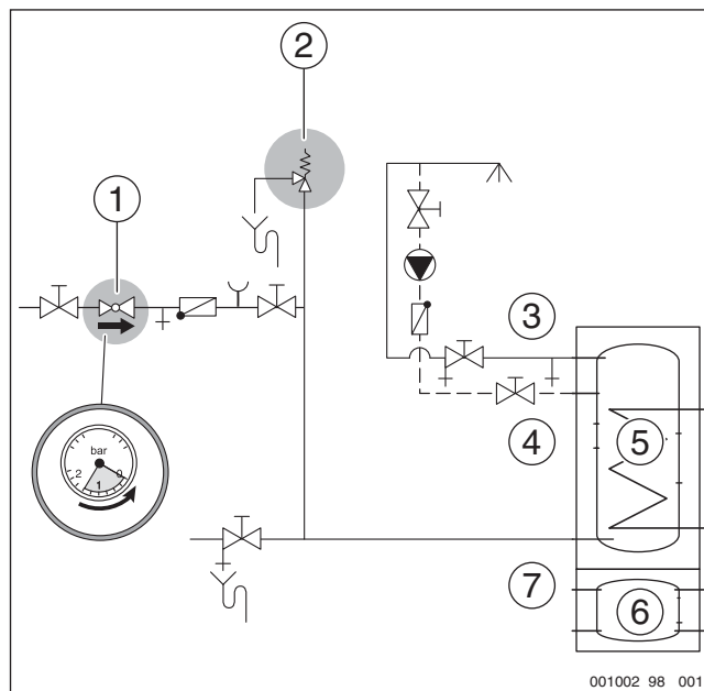
Bild 8 Hydraulischer Anschluss des Kombispeichers BPU...
