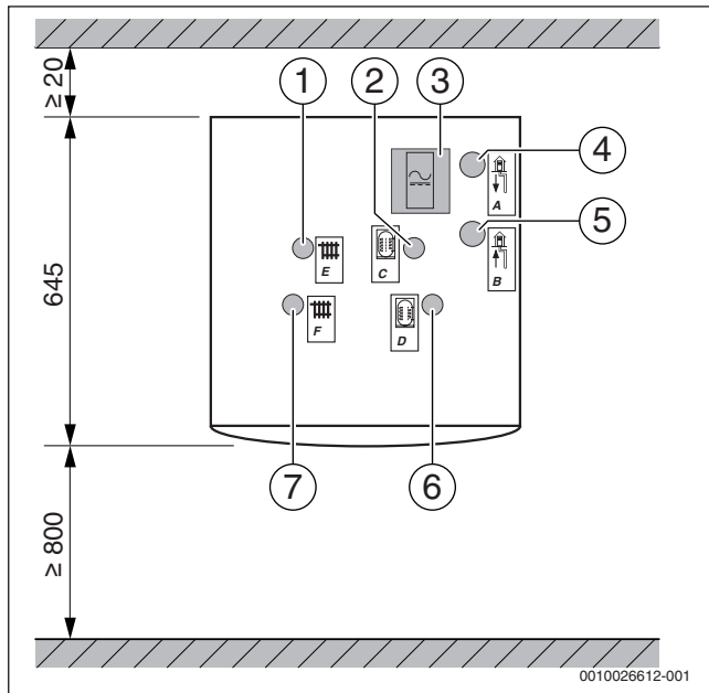
Bild 6 Abmessungen und Mindestabstände WPS 10-1...17-1 (Draufsicht)
