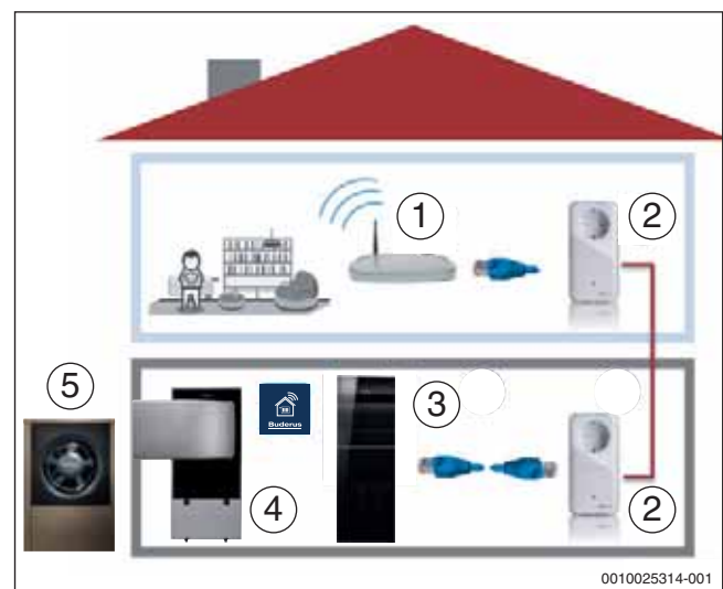
Bild 26 PowerLAN
