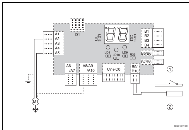
Σχ. 1 Σύνδεση της τριόδου βάνας για τη λειτουργία του συστήματος ελέγχου του ζεστού νερού χρήσης ή της εναλλακτικής πηγής
