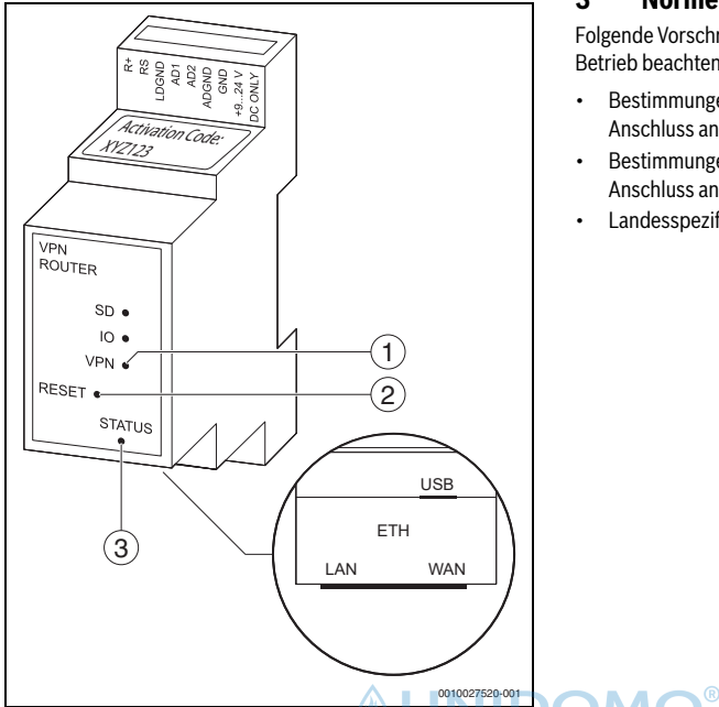
Bild 1 Geräteübersicht
