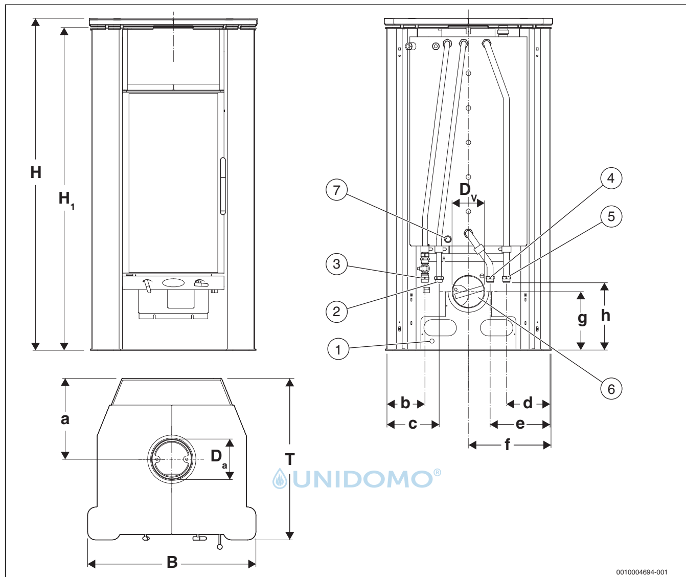
Bild 11 Abmessungen blueline 4 W
