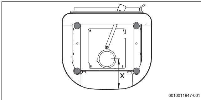
Bild 13 Anschlussmaß am Verbrennungsluftstutzen (Untersicht; beispielhafte Darstellung)
