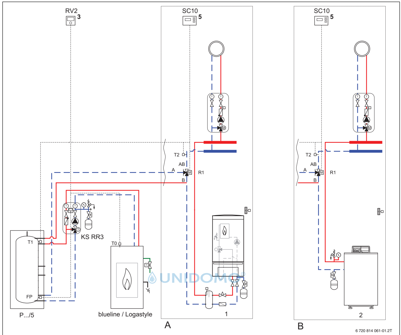
Bild 20 Anlagenbeispiel
