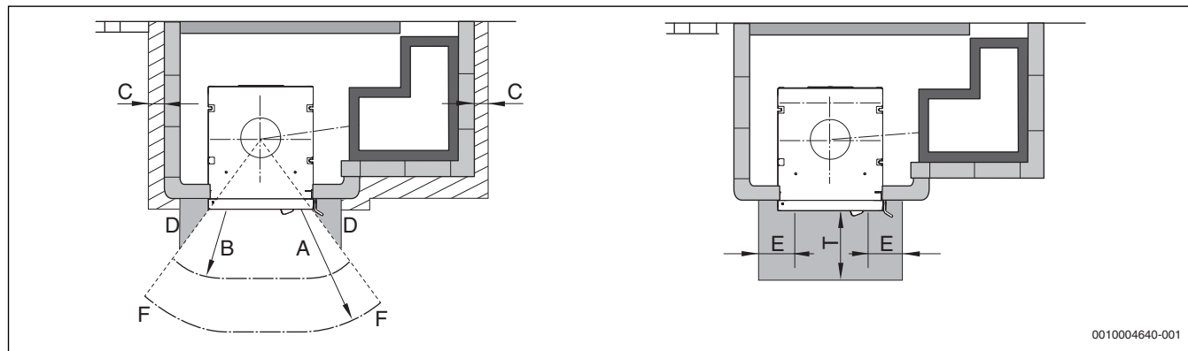
Bild 14 Äußere Mindestabstände
