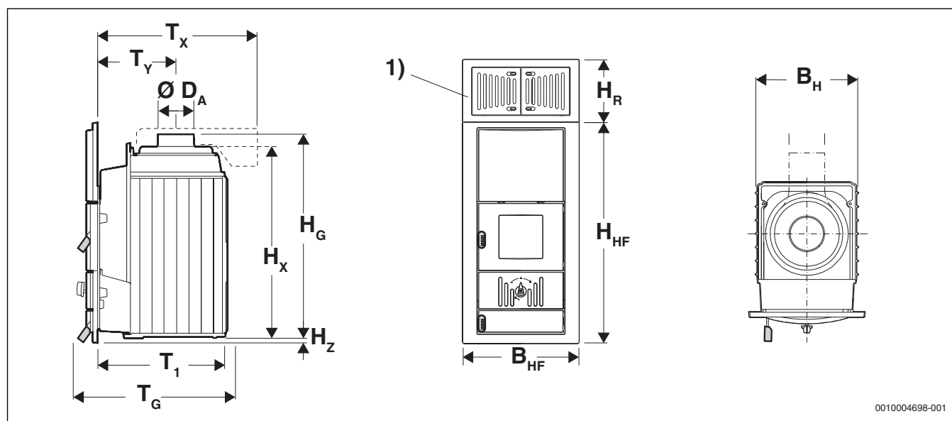
Bild 4 Abmessungen H206
