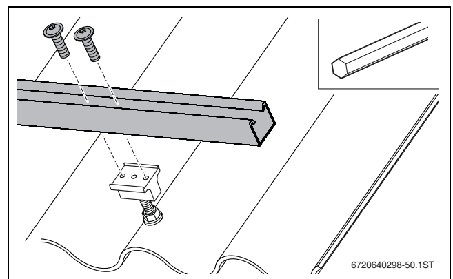
Bild 31 Profilschienen montieren
