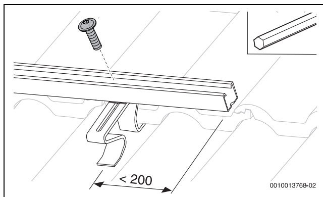
Bild 36 Profilschiene montieren
