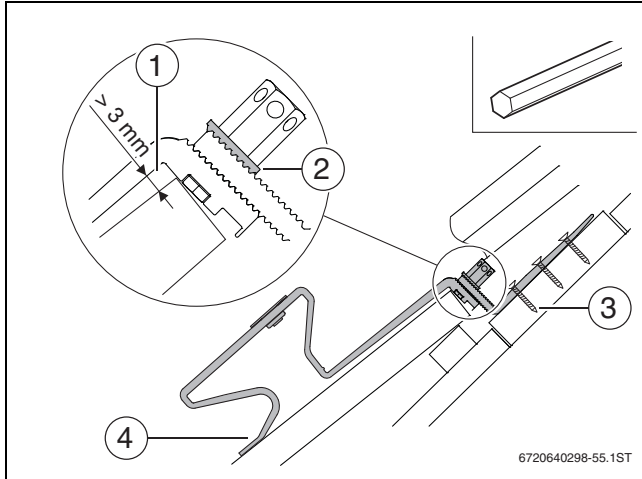
Bild 23 Sparrenanker befestigen
