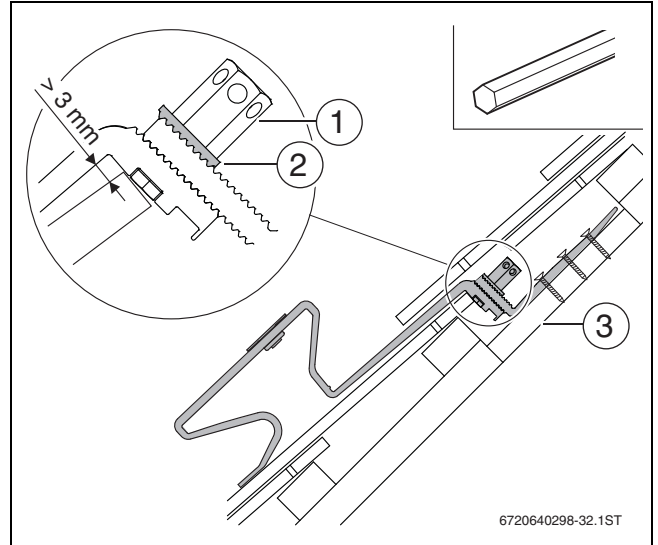
Bild 24 Sparrenanker montieren
