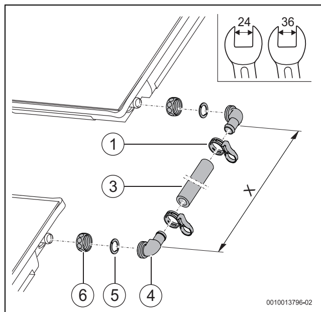
Bild 63 Verbindungs-Set montieren
