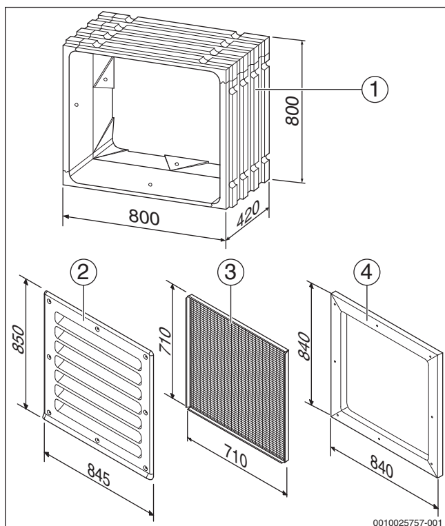
Bild 11 Wandschneidung und Zubehör
