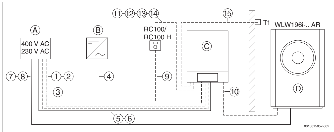
Bild 14 Kabelzugplan der elektrischen Leitungen bei Außenaufstellung (Prinzipdarstellung)
