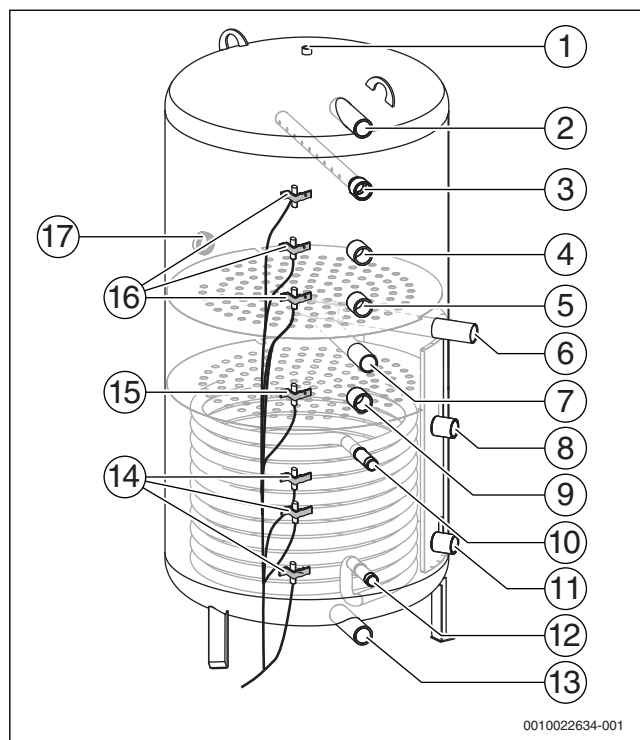
Bild 10 Übersicht der hydraulischen Anschlüsse und Fühlerpositionen
