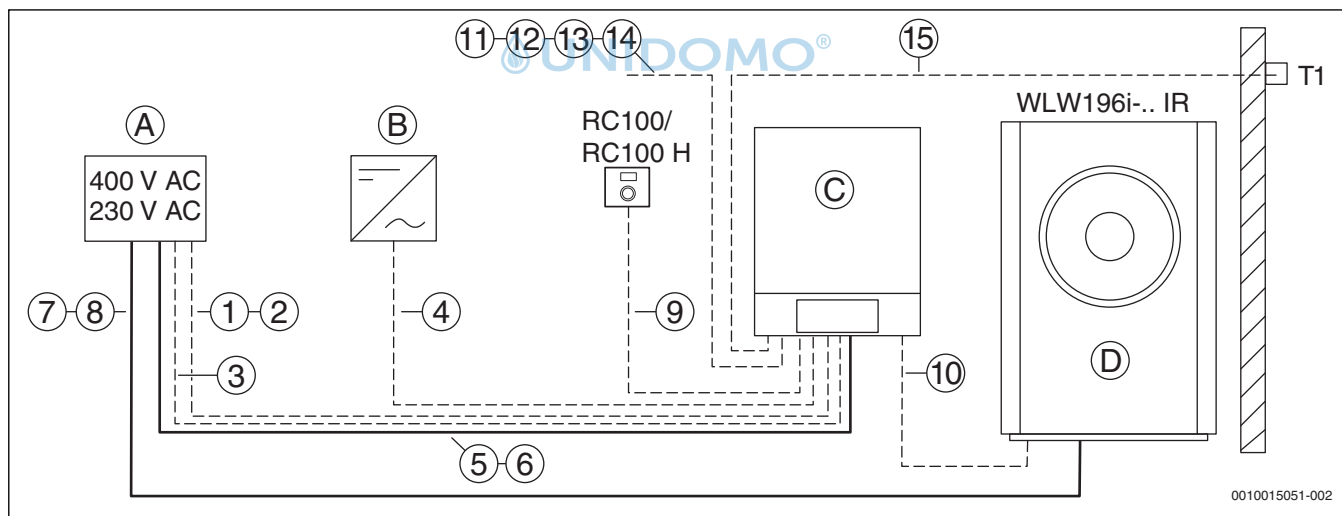
Bild 15 Kabelzugplan der elektrischen Leitungen bei Innenaufstellung (Prinzipdarstellung)
