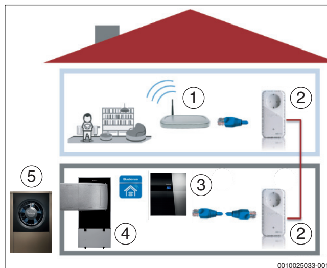
Bild 22 PowerLAN
