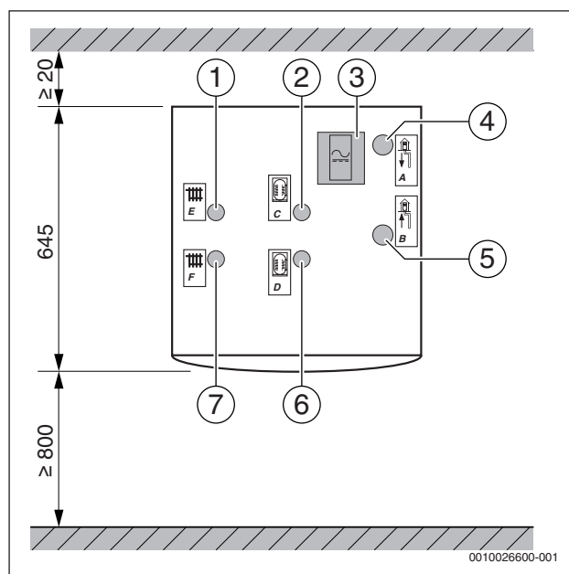
Bild 5 Abmessungen und Mindestabstände WPS 6...8-1 (Draufsicht)
