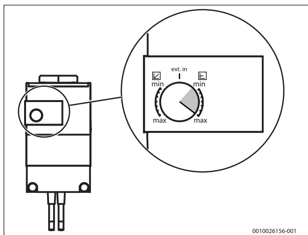
Bild 13 Einstellungen an der Solekreispumpe
