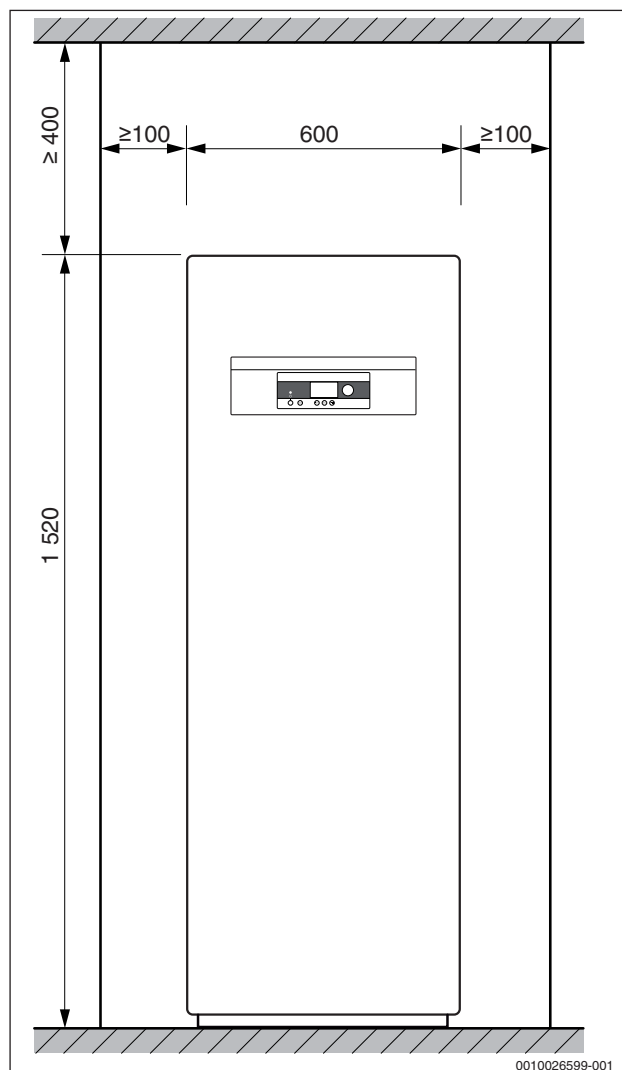
Bild 4 Abmessungen und Mindestabstände WPS 6...17-1 (Ansicht)
