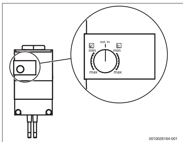
Bild 14 Einstellungen an der primären Heizkreispumpe
