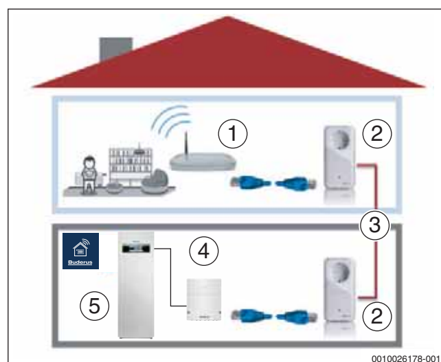
Bild 22 PowerLAN
