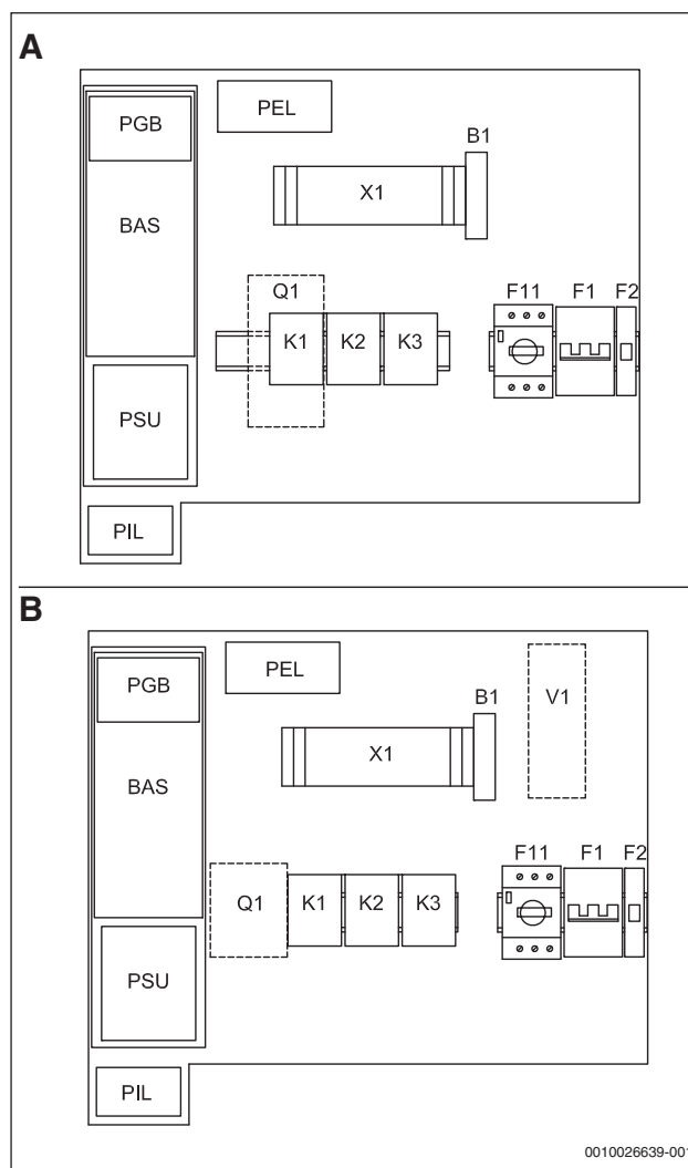
Bild 15 Leiterplatten WPS 6-1...17-1
