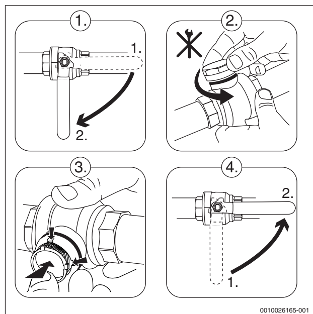
Bild 2 Reinigung der Filter
