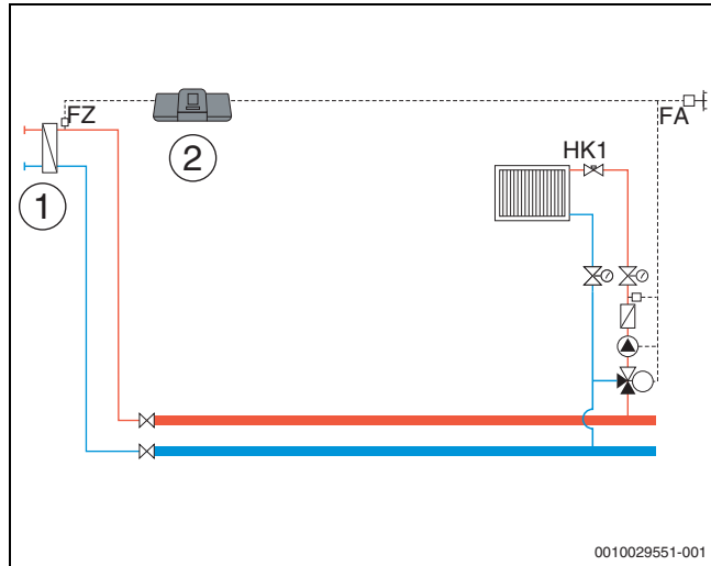
Bild 28 Variante 1: Fremde Wärmequelle mit Zubringerpumpe, Lastbegrenzung und Kompensation Wärmeverluste über FZ
