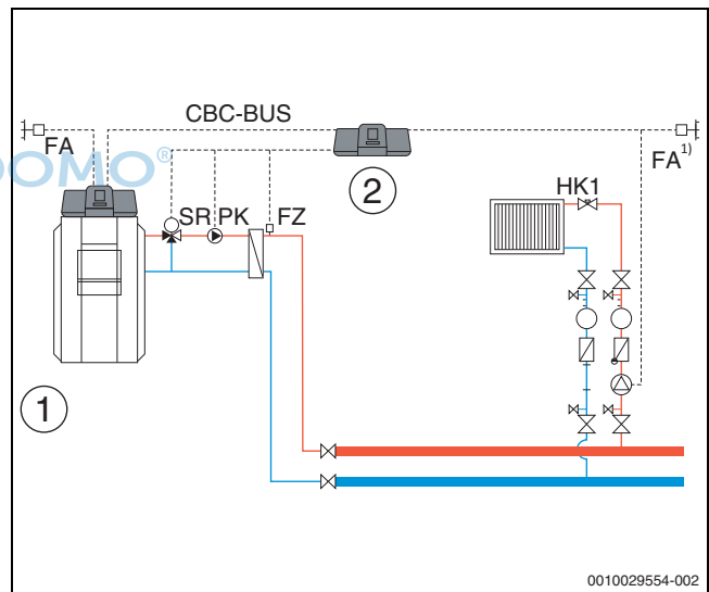
Bild 31 Variante 1: Unterstation mit Vormischfunktion, Kompensation Wärmeverluste über FZ, Lastbegrenzung
