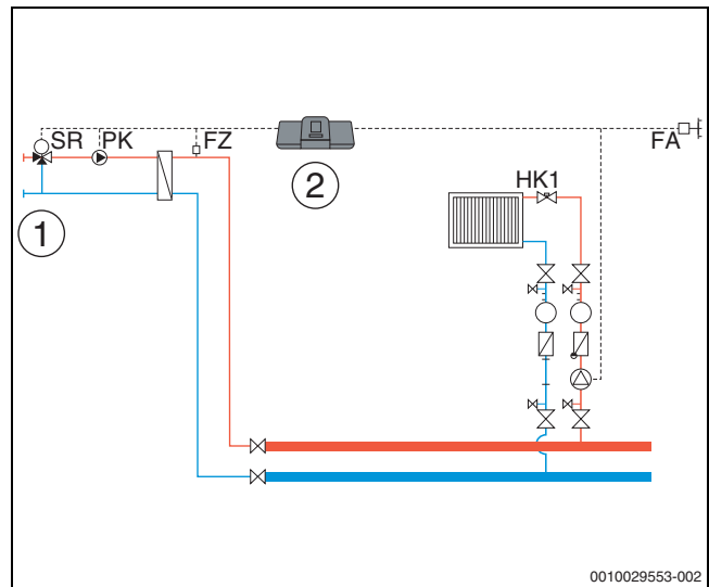
Bild 30 Variante 3: Fremde Wärmequelle ohne Zubringerpumpe, Lastbegrenzung, Vormischfunktion, Kompensation Wärmeverluste über FZ
