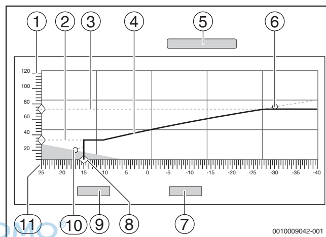
Bild 41 Heizkurve
