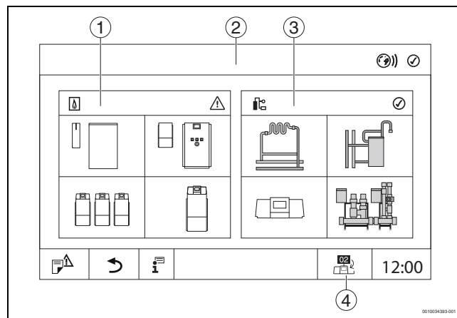
Bild 11 Systemübersicht (Beispiel)
