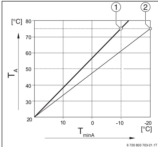
Bild 25 Einstellung der Heizkurve: Einstellung der Steigung über Auslegungstemperatur und minimale Außentemperatur
