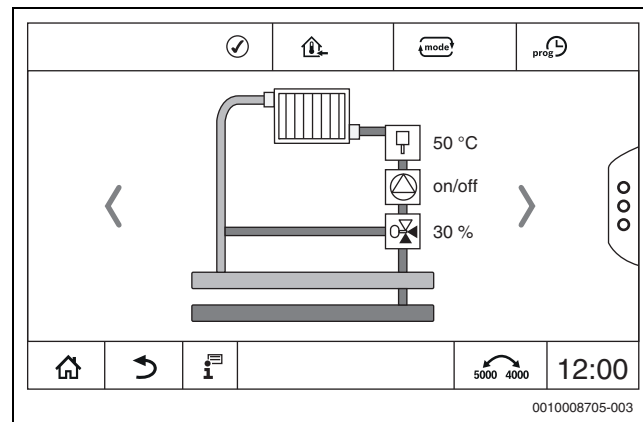
Bild 12 Heizkreisansicht Serie 5000
