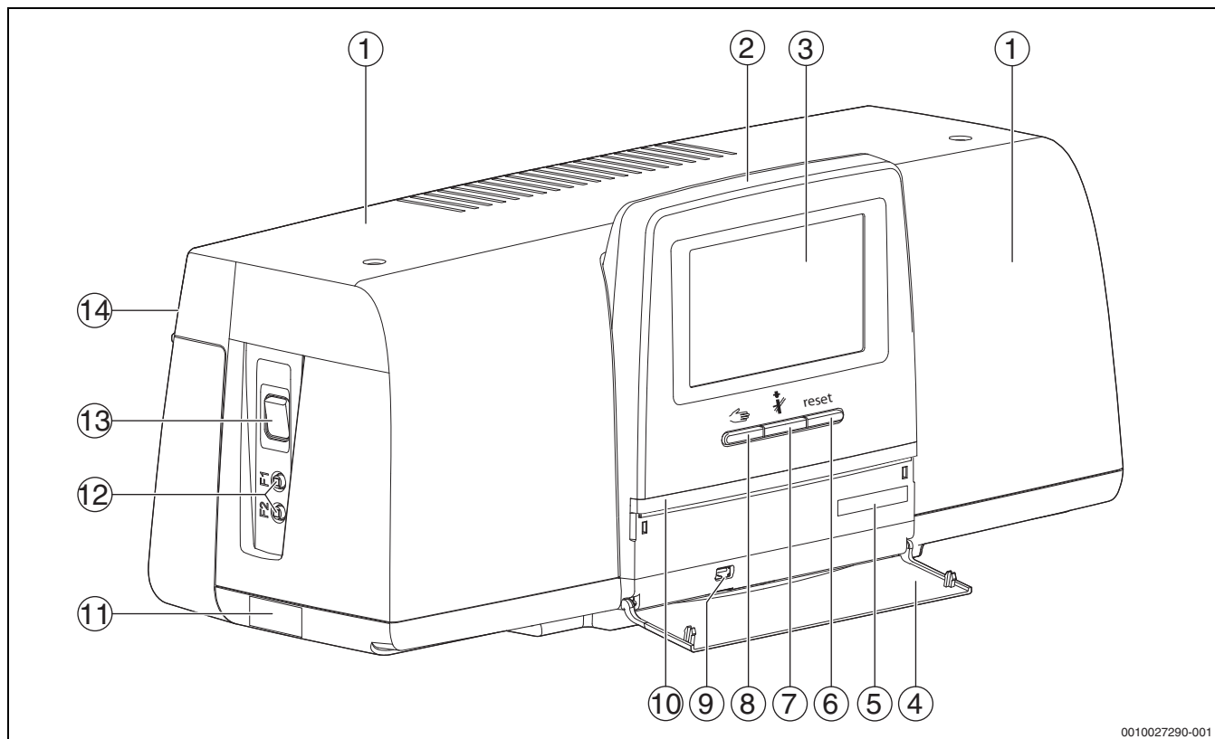
Bild 1 Übersicht des Regelgeräts und der Bedienelemente
