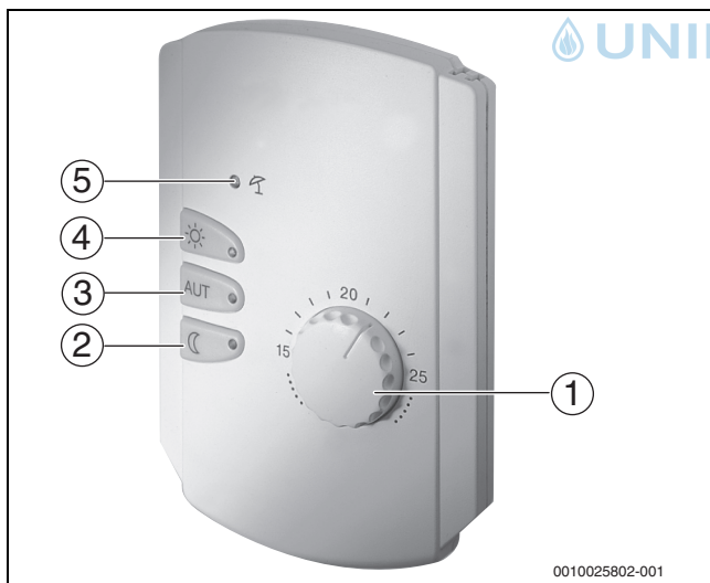
Bild 23 Fernbedienung
