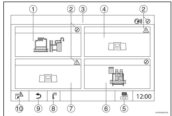
Bild 3 Anlagenübersicht (Beispiel)
