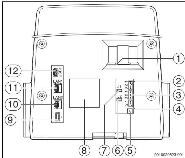
Bild 7 Anschlüsse Bedieneinheit
