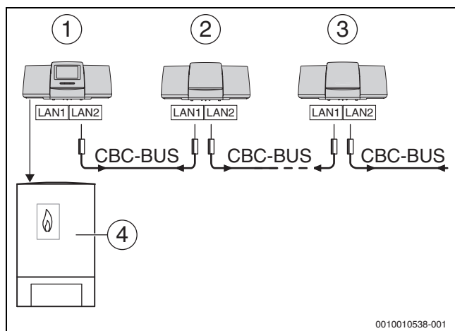
Bild 9 Regelgeräteanbindung
