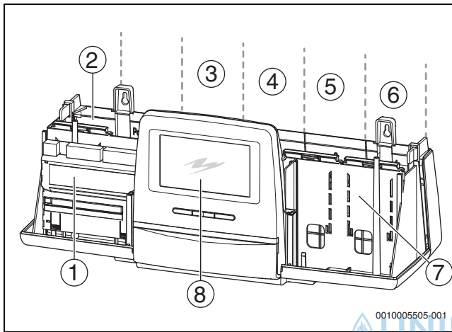
Bild 5 Übersicht Steckplätze
