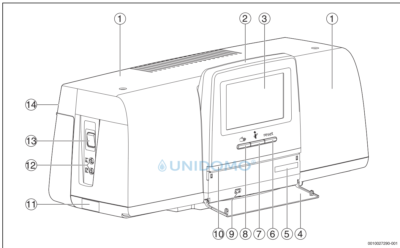
Bild 1 Übersicht Regelgerät
