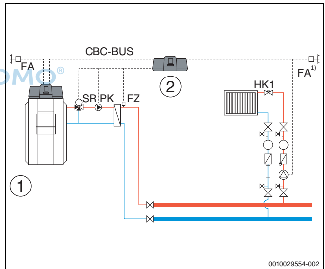
Bild 28 Variante 1: Unterstation mit Vormischfunktion, Kompensation Wärmeverluste über FZ, Lastbegrenzung
