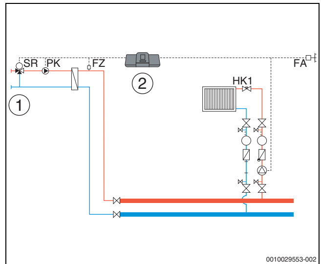
Bild 27 Variante 3: Fremde Wärmequelle ohne Zubringerpumpe, Lastbegrenzung, Vormischfunktion, Kompensation Wärmeverluste über FZ
