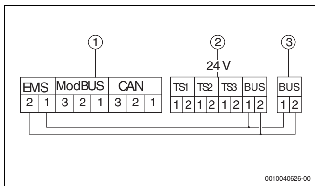
Bild 5 Elektrischer Anschluss
