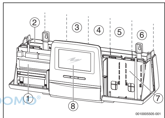
Bild 1 Übersicht Steckplätze
