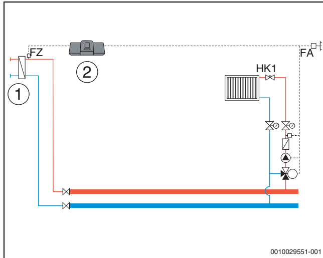
Bild 25 Variante 1: Fremde Wärmequelle mit Zubringerpumpe, Lastbegrenzung und Kompensation Wärmeverluste über FZ
