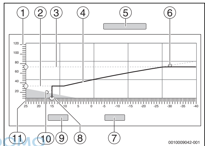
Bild 38 Heizkurve
