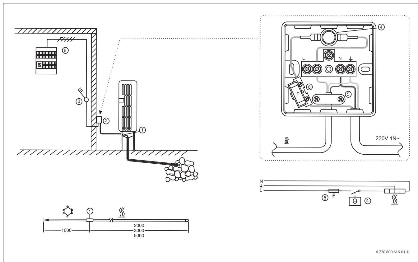
Fig. 52 Instrucțiuni de racordare pentru pompa de căldură cu conductă de apă între partea interioară și cea exterioră
