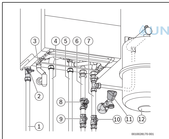
Bild 1 Anschlusszubehör (Beispiel)
