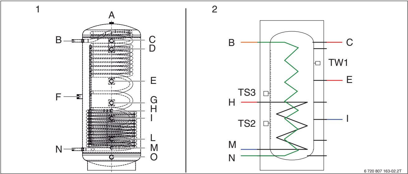
Bild 5 Übersicht der Kombispeicher-Anschlüsse und Fühlerpositionen
