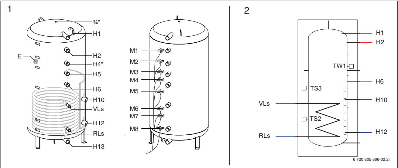
Bild 6 Übersicht der Pufferspeicher-Anschlüsse und Fühlerpositionen
