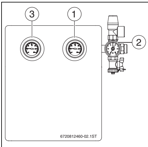
Bild 9 Solarstation
