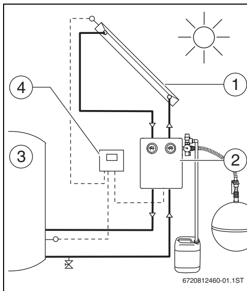
Bild 3 Anlagenschema
