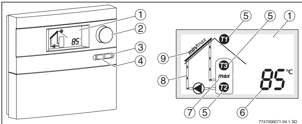
Bild 10 Regler und Display
