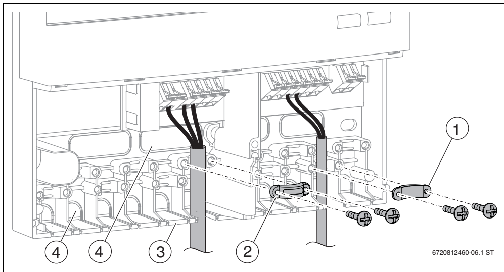
Bild 7 Durchführung und Befestigung der Kabel
