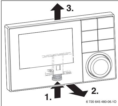
Bild 5 Bedieneinheit abnehmen
