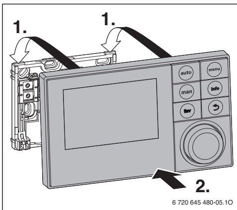
Bild 4 Bedieneinheit einhängen
