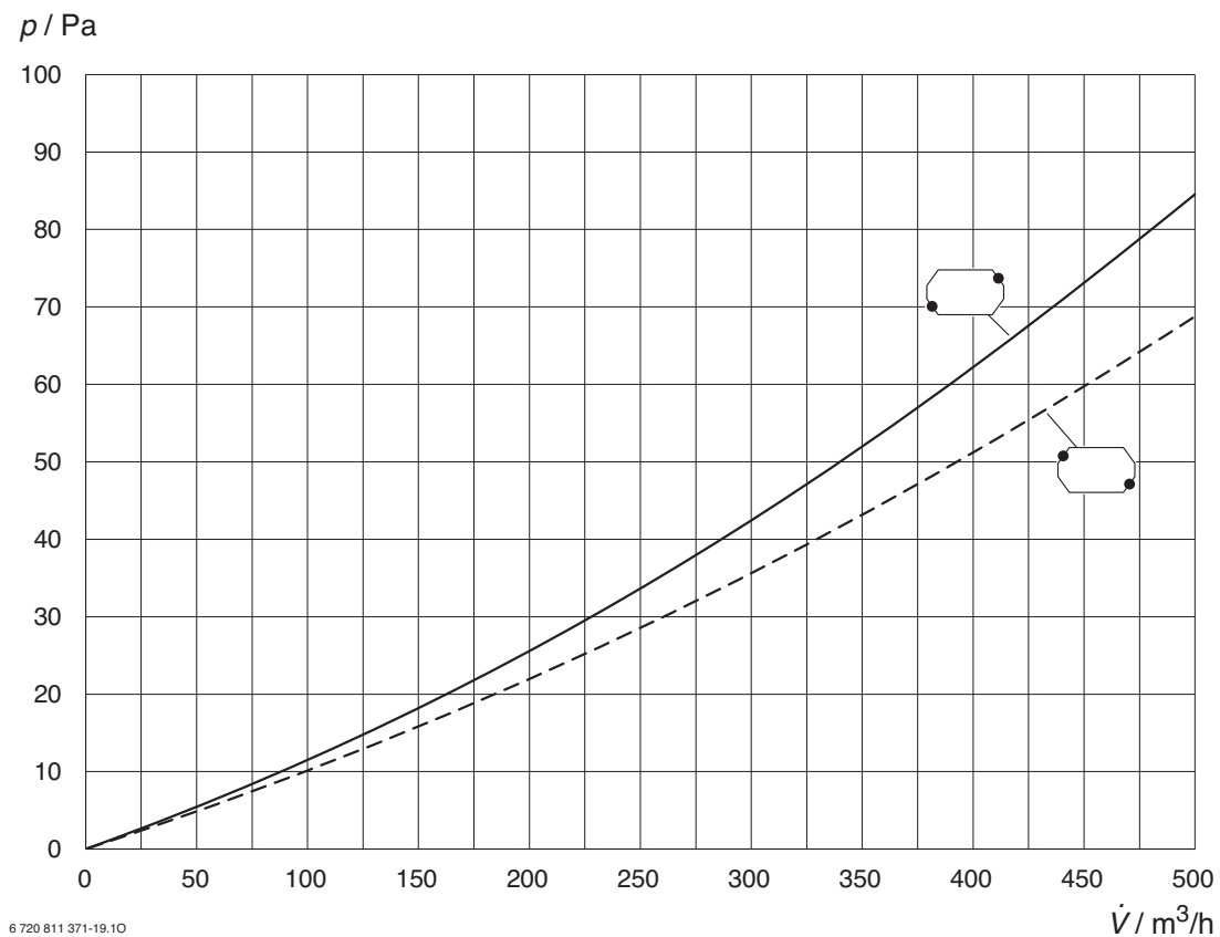
Bild 47 Volumenstrom und Differenzdruck HRV2-350 (S)
