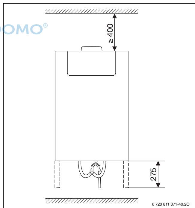
Bild 22 HRV2-230 (S), HRV2-350 (S)
