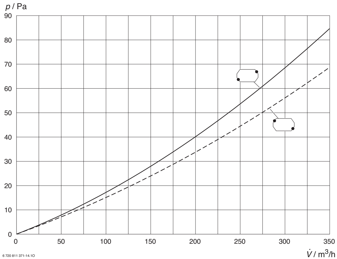
Bild 46 Volumenstrom und Differenzdruck HRV2-230 (S)
