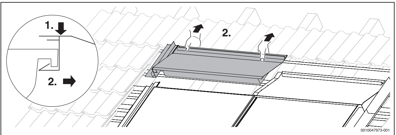
Bild 86 Eindeckblech abziehen
