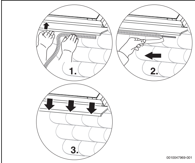
Bild 81 Unteres Eindeckblech auf Eindeckung kleben
