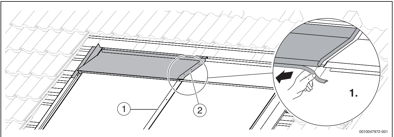
Bild 85 Dichtlippe abziehen
