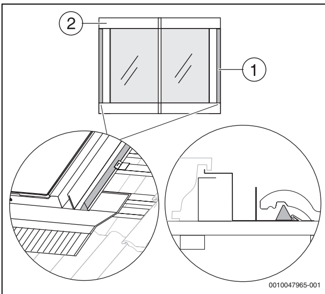
Bild 77 Dreieckdichtband einlegen
