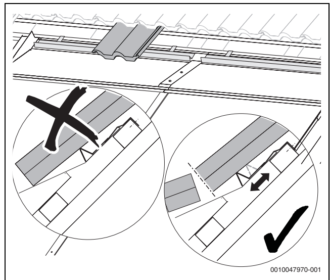
Bild 82 Dachziegelauflage positionieren
