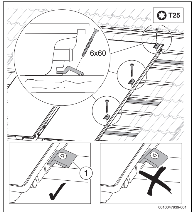
Bild 50 Niederhalter festschrauben
