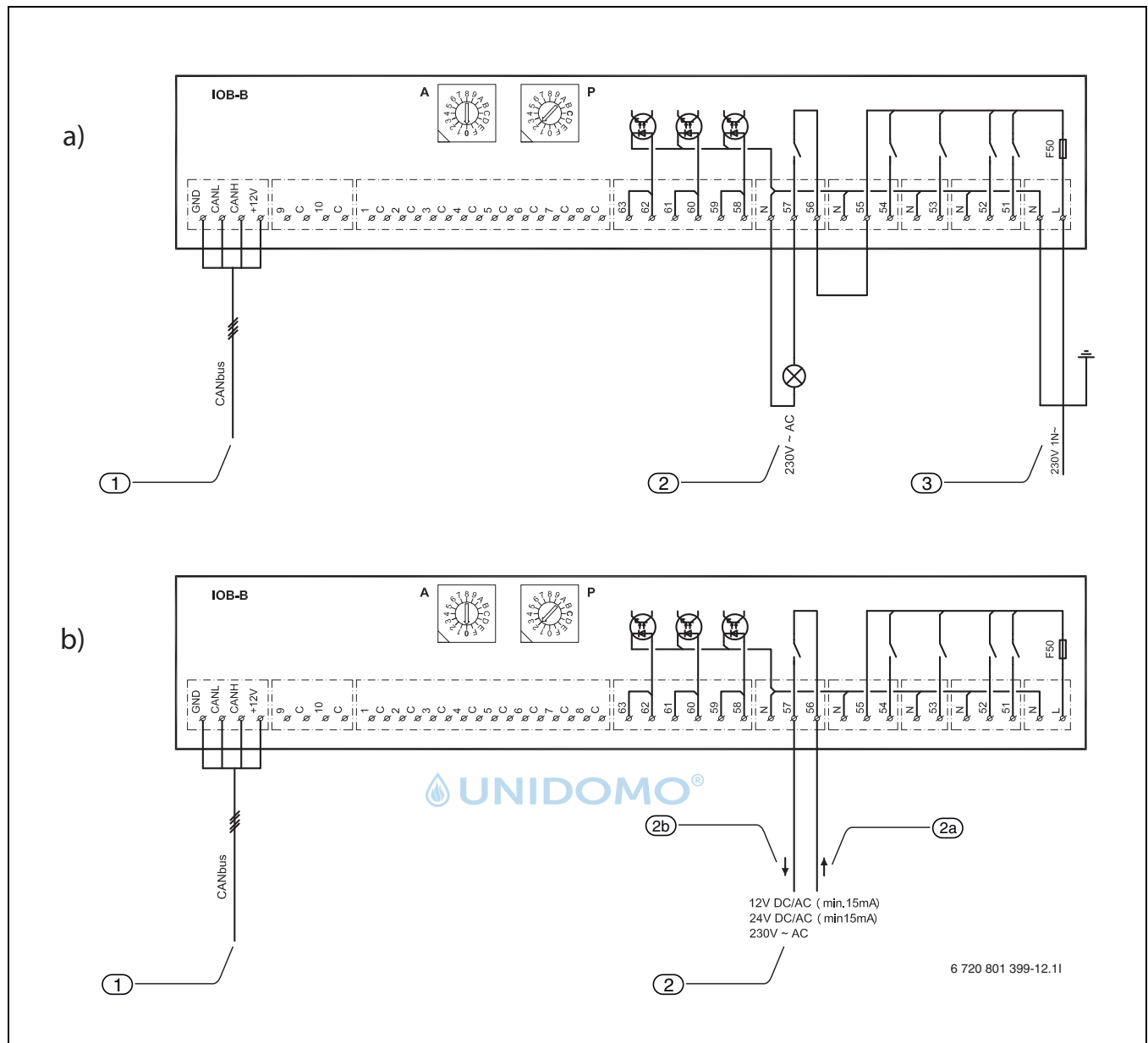
Afb. 25 Schakelschema. a) 230 V uitgangssignaal b) potentiaalvrij contact
