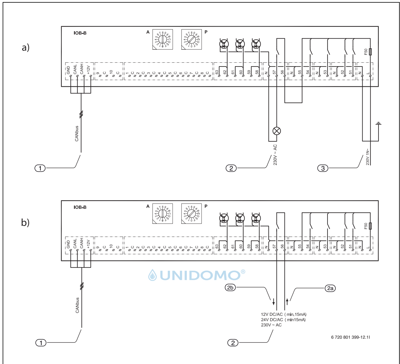
Fig. 16 Schéma de connexion. a) Signal de sortie de 230 V b) Contact libre de potentiel
