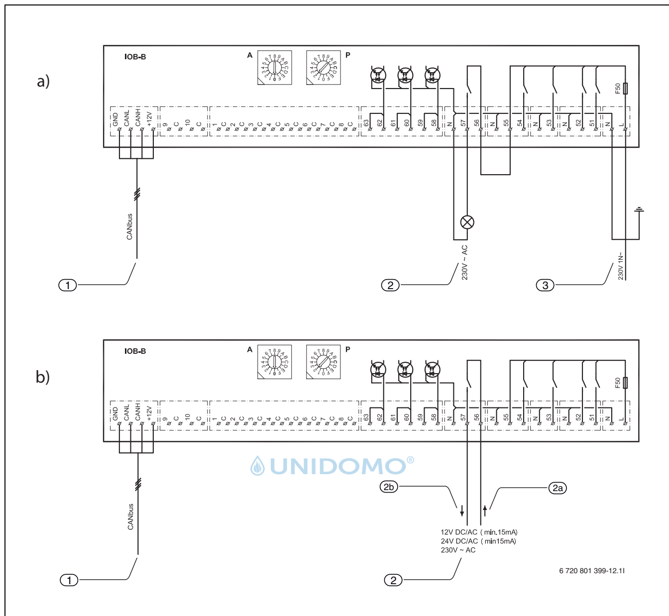
Fig. 43 Schema elettrico. a) segnale di uscita 230 V b) con contatto a potenziale zero
