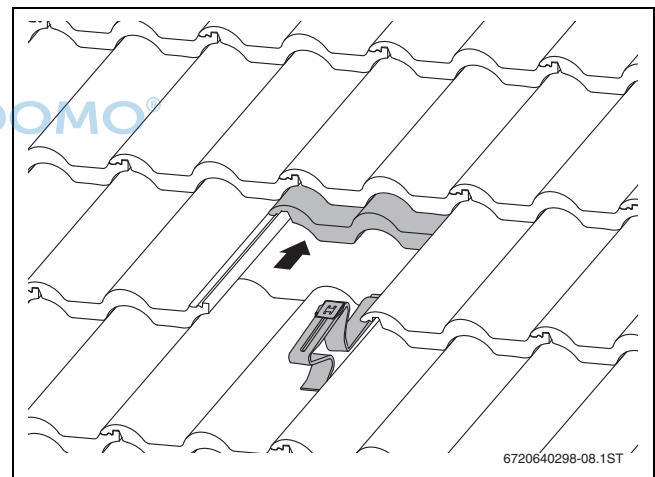
Bild 14 Eingängter Dachhaken
