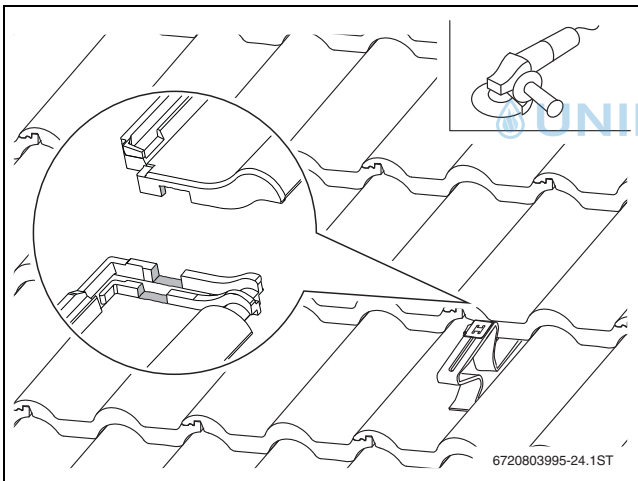
Bild 16 Dachziegel anpassen
