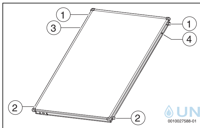
Bild 1 Kollektortyp senkrecht
