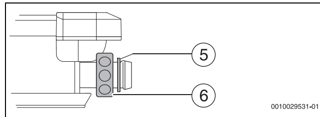
Bild 56 Überwurfmutter montieren
