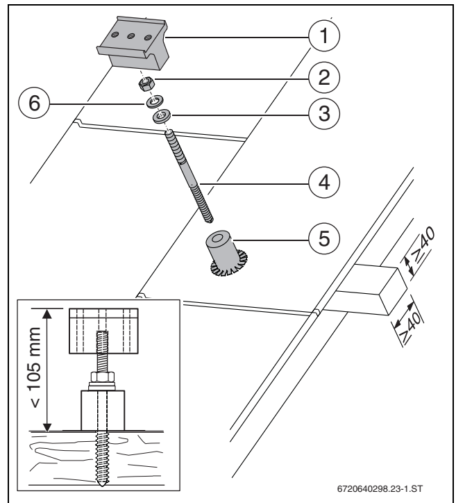
Bild 23 Stockschrabe montieren
