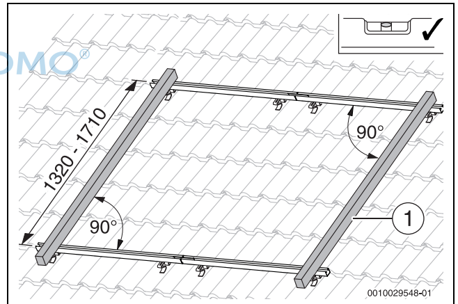
Bild 31 Profilschienen ausrichten
