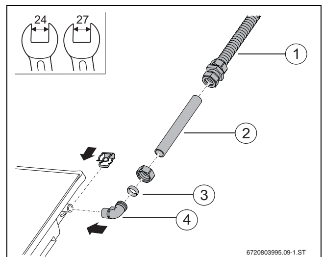
Bild 63 Verbindungs-Set montieren
