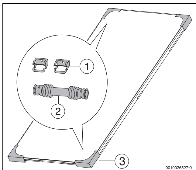
Bild 7 2 Transportschutzdecken beinhalten je 1 Verbindungs-Set (1 Verbindungs-Set enthält 2 Klammern und 1 Wellrohrverbinder)
