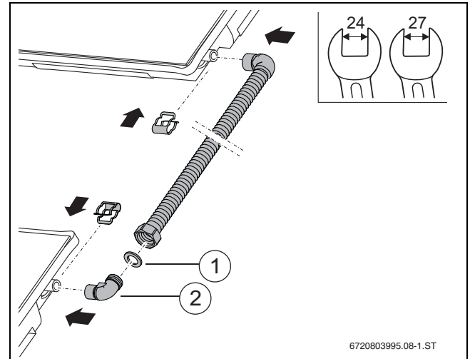
Bild 62 Anschlussrohr montieren
