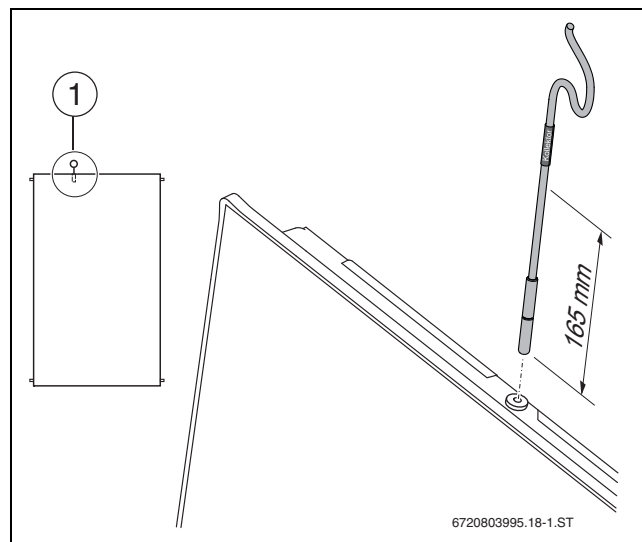
Bild 53 Kollektortemperaturfühler montieren
