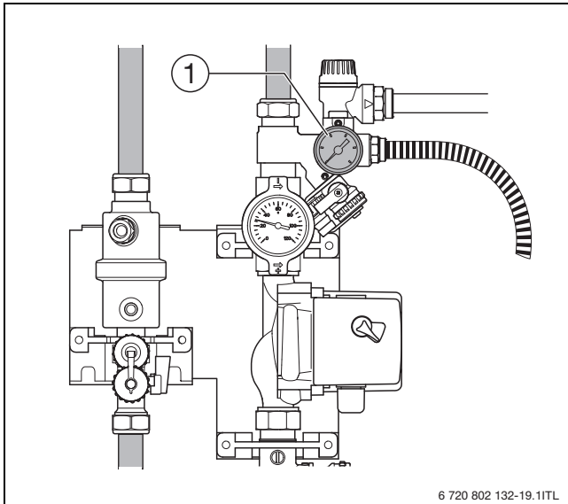
Bild 22 Manometeranzeige prüfen
