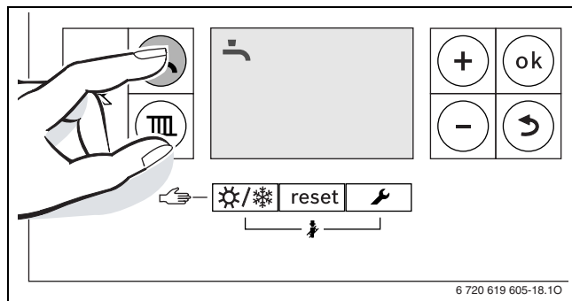
Bild 31 Anzeige Warmwasserbetrieb
