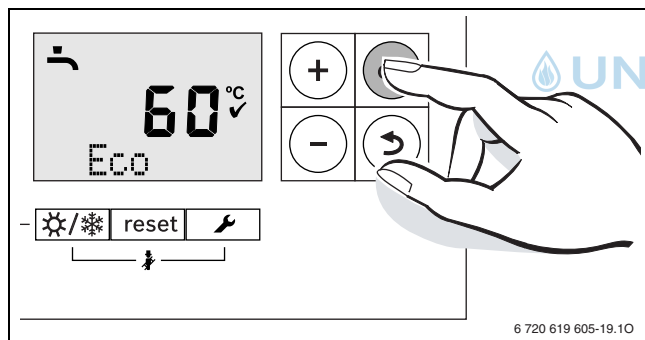
Bild 32 Anzeige eco-Betrieb
