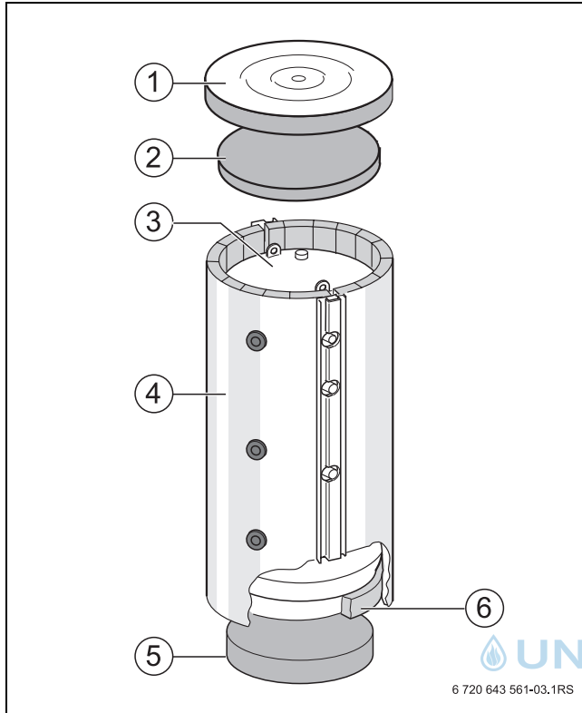
Bild 1 Pufferspeicher
