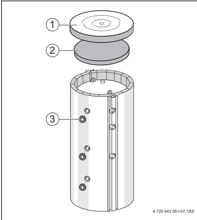
Bild 7 Speicherhaube montieren
