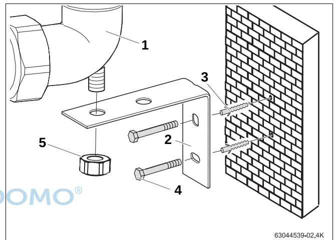
Abb. 5 Wandhalter montieren (Darstellung ohne hintere Wärmedämmschale)
