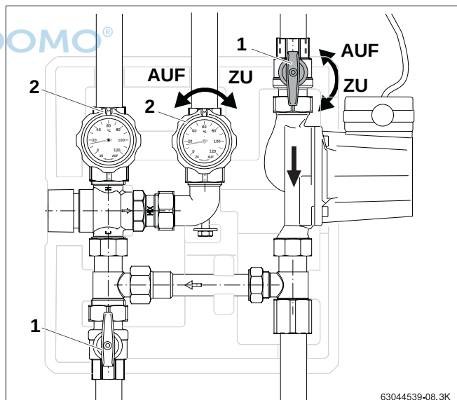
Abb. 11 Kugelhähne schließen und öffnen
