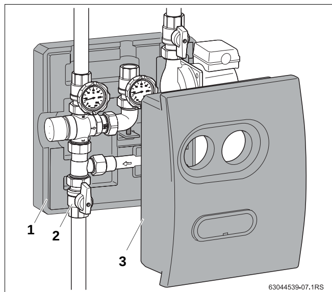
Abb. 8 Wärmedämmschalen montieren
