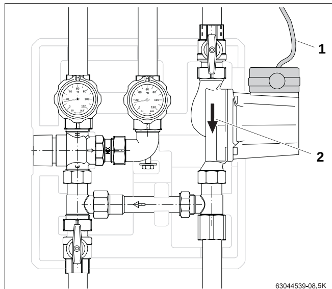
Abb. 7 Mischgruppe elektrisch anschließen
