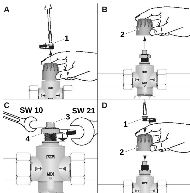
Abb. 9 Temperatur einstellen bei Ausführung A mit blauem Drehknopf
