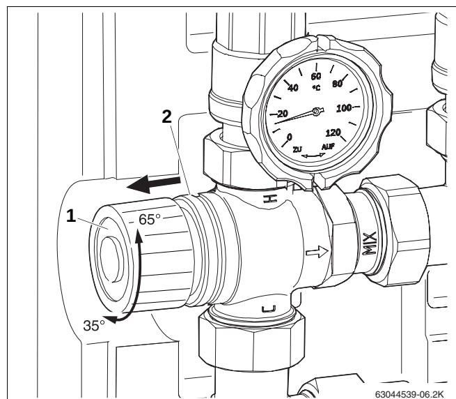
Abb. 10 Temperatur einstellen (Ausführung B, mit schwarzem Drehknopf)
