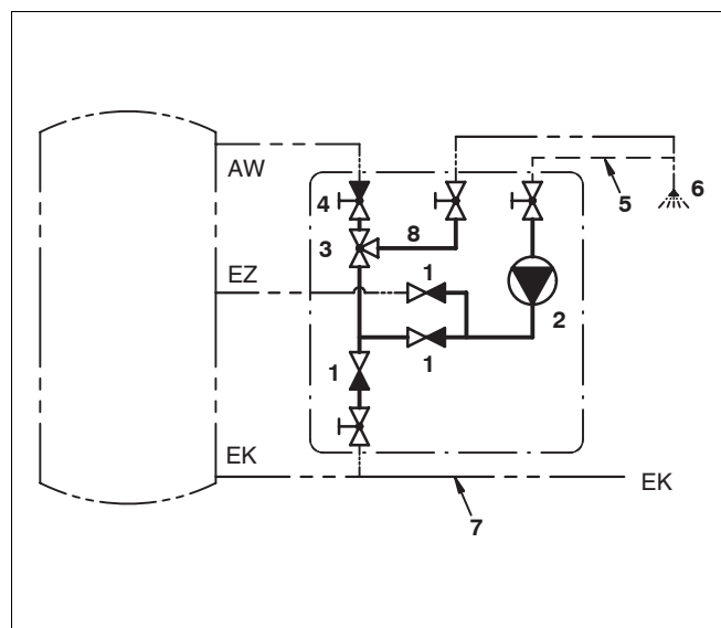
Abb. 4 Schaltbild
