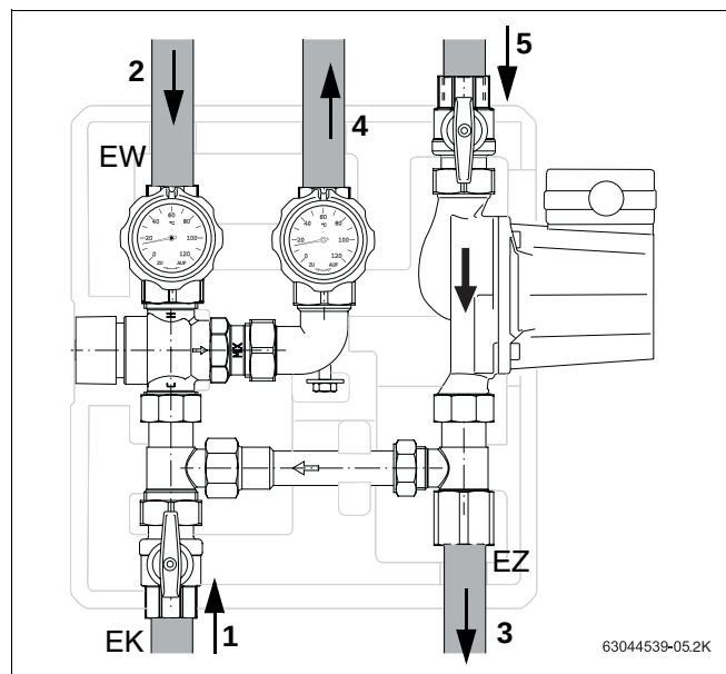
Abb. 6 Mischgruppe mit Speicher- und Trinkwassernetz verbinden
