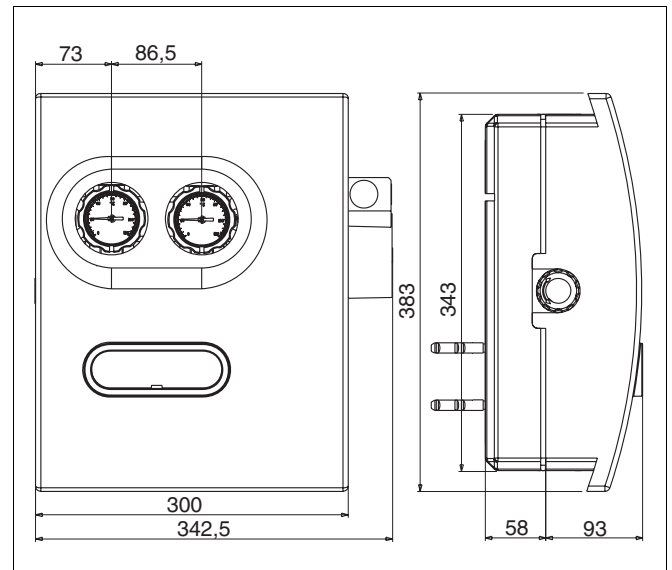
Abb. 1 Abmessungen
