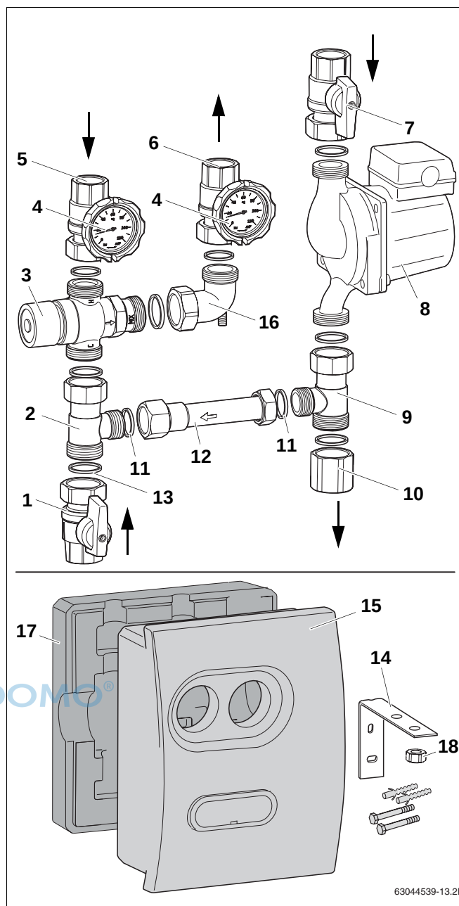
Abb. 3 Lieferumfang Mischgruppe
