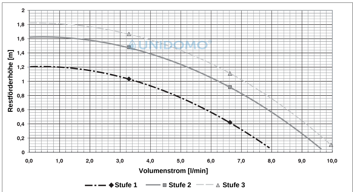
Abb. 2 Restförderhöhe Zirkulationspumpe
