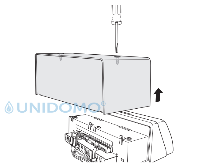
Abb. 4 Abdeckhaube abnehmen
