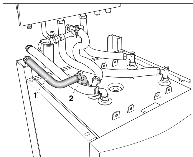
Abb. 14 Zirkulationspumpenanschluss montieren (Unterputzmontage)
