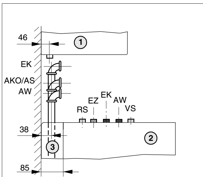
Abb. 7 Abmessungen der Hydraulikanschlüsse S135/S160, Aufputzmontage (Seitenansicht)
