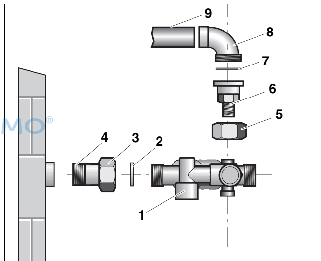
Abb. 26 Zirkulationspumpenanschluss montieren (Unterputzmontage)
