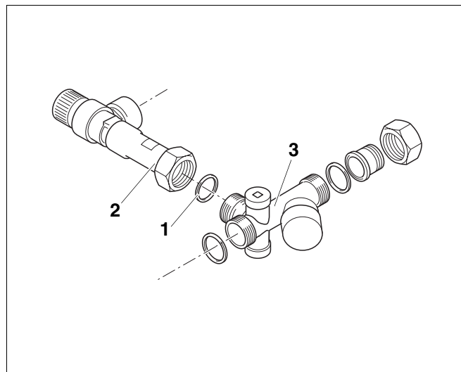
Abb. 12 Sicherheitsgruppe montieren
