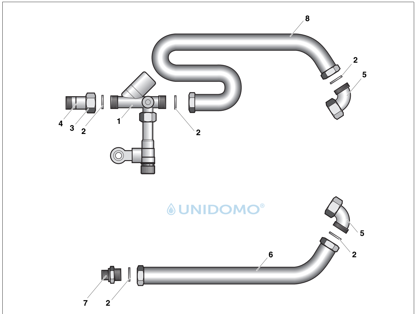
Abb. 1 Lieferumfang sanitärseitiges Anschluss-Set S-Flex
