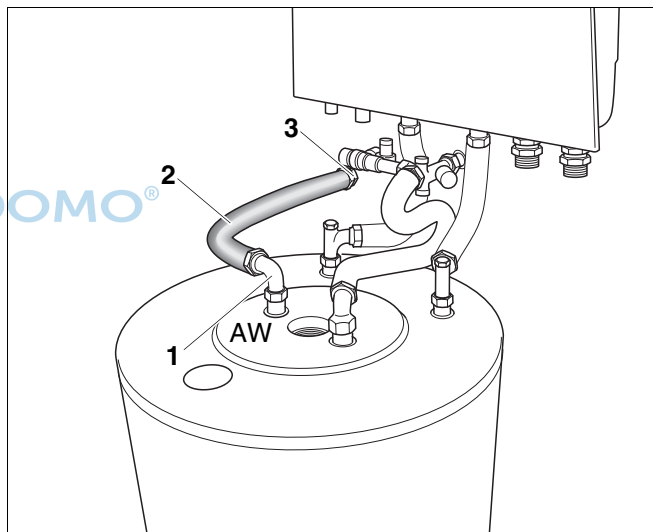
Abb. 28 Warmwasser-Anschlussrohr montieren
