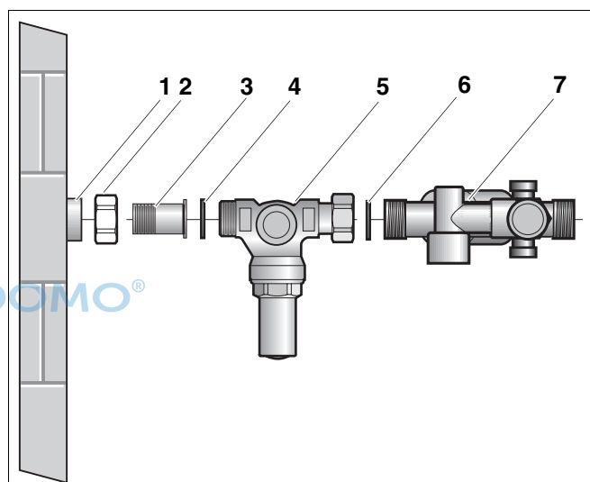
Abb. 13 Druckminderer U-DM montieren (Unterputzmontage)
