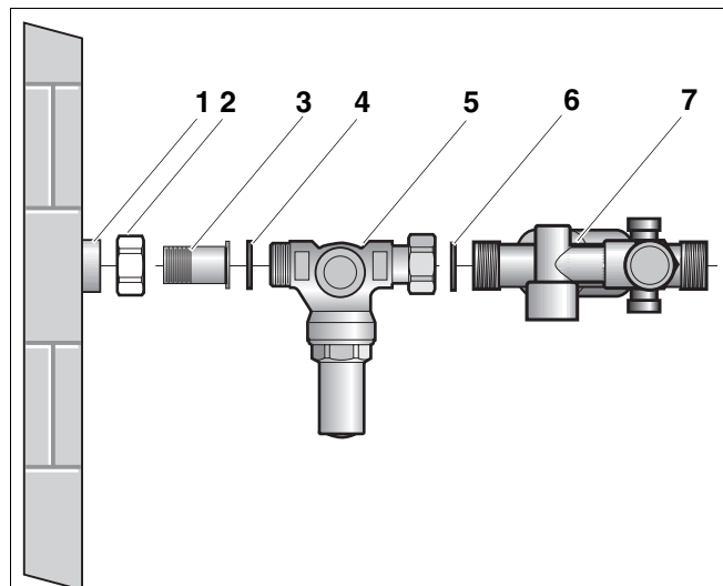
Abb. 25 Druckminderer U-DM montieren (Unterputzmontage)
