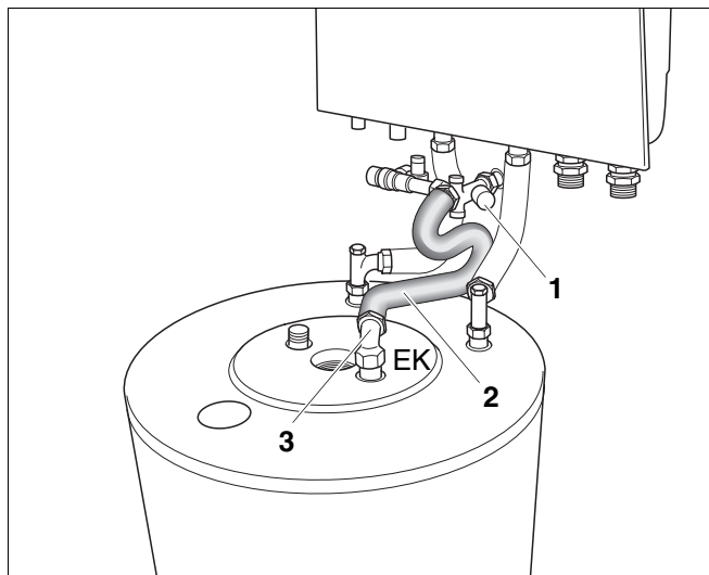
Abb. 27 Kaltwasser-Anschlussrohr montieren
