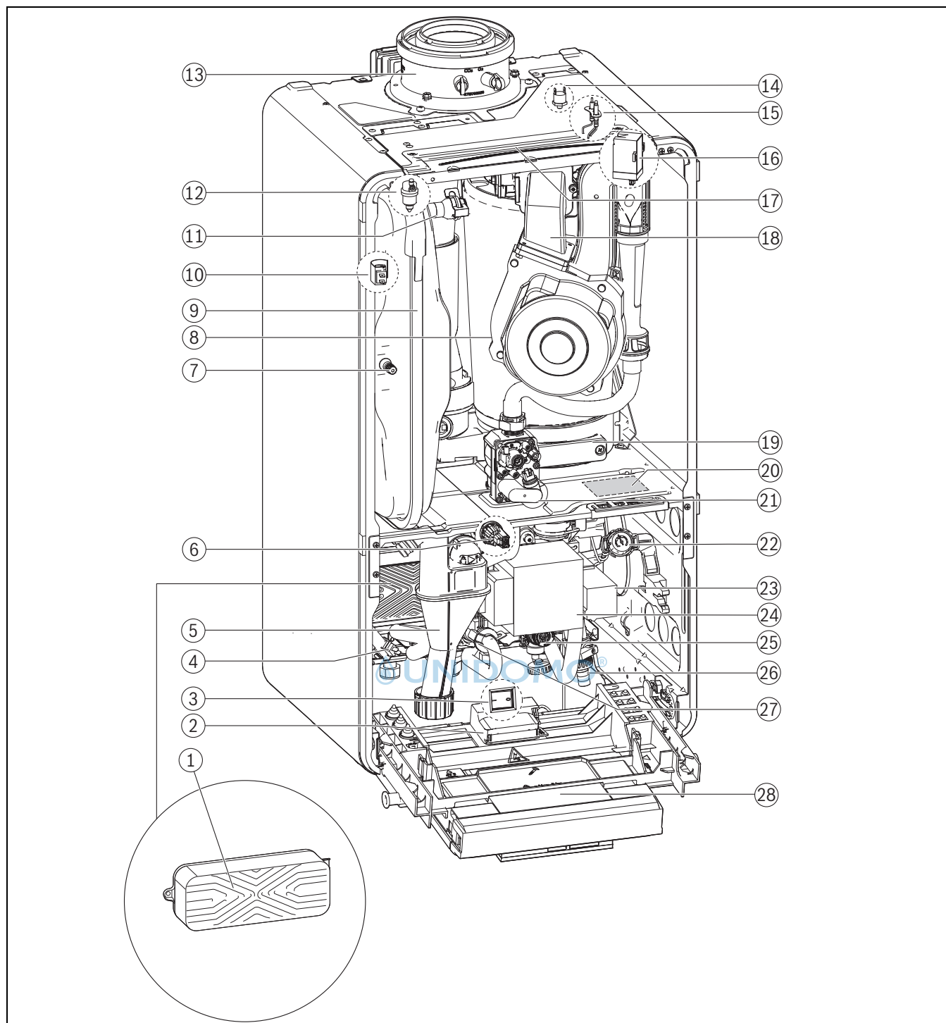
Bild 1 Produktübersicht Kombigerät
