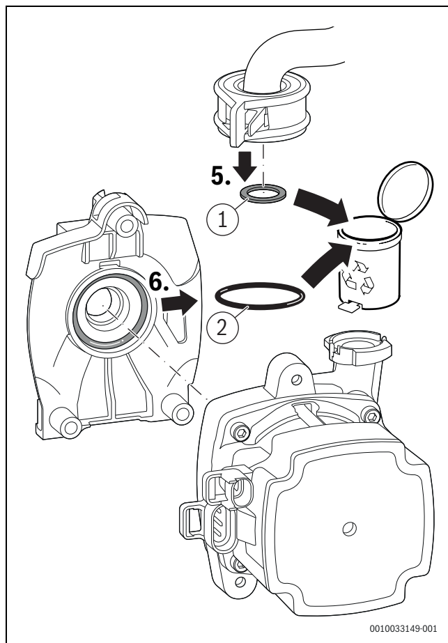
Bild 30 Dichtungen entsorgen
