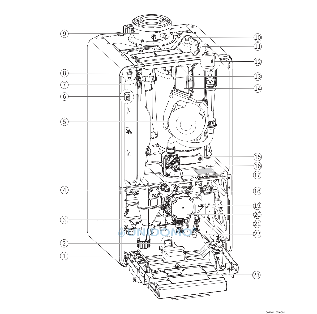
Bild 2 Produktübersicht Speichergerät
