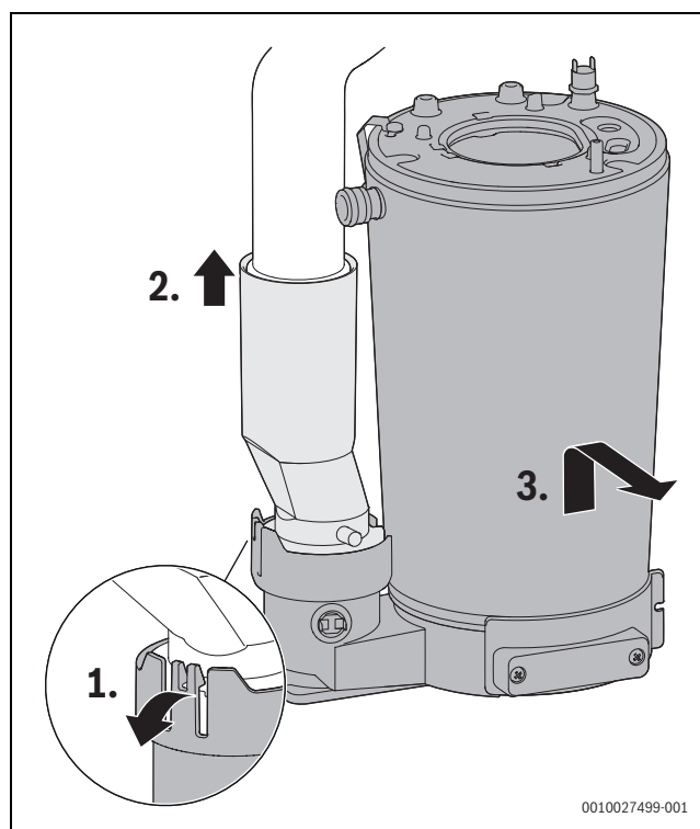
Bild 26 Wärmeblock ausbauen
