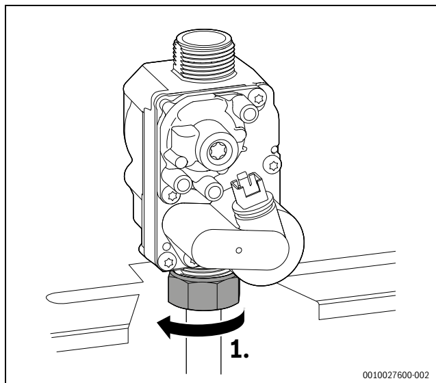
Bild 33 Überwurfmutter lösen
