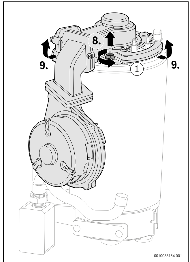
Bild 13 Brennerdeckel mit Gebläse und Mischeinrichtung abnehmen [1] M 8
