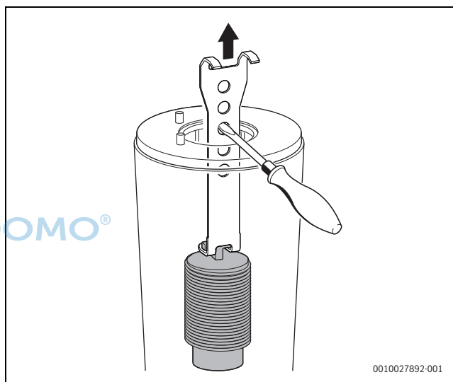
Bild 18 Unteren Verdrängungskörper herausnehmen
