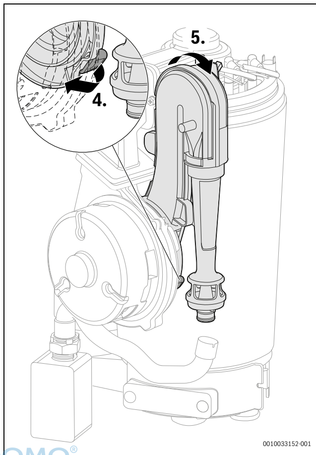
Bild 11 Venturirohr abnehmen
