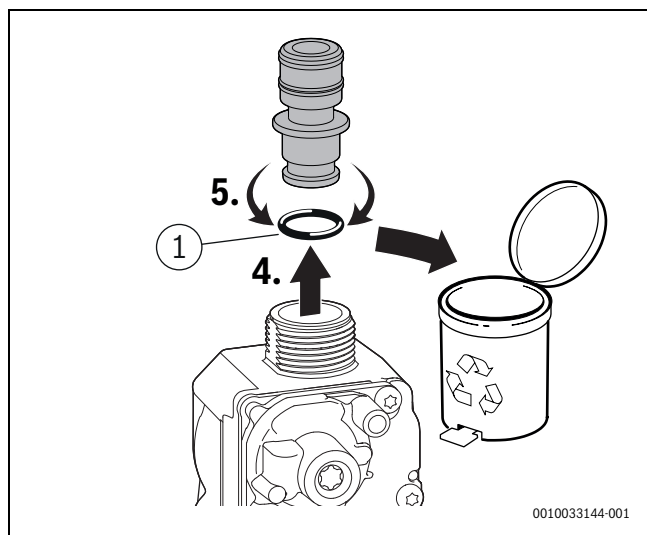
Bild 32 Gasdrossel abnehmen
