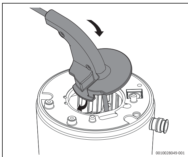
Bild 19 Bürste in den Wärmeblock einsetzen
