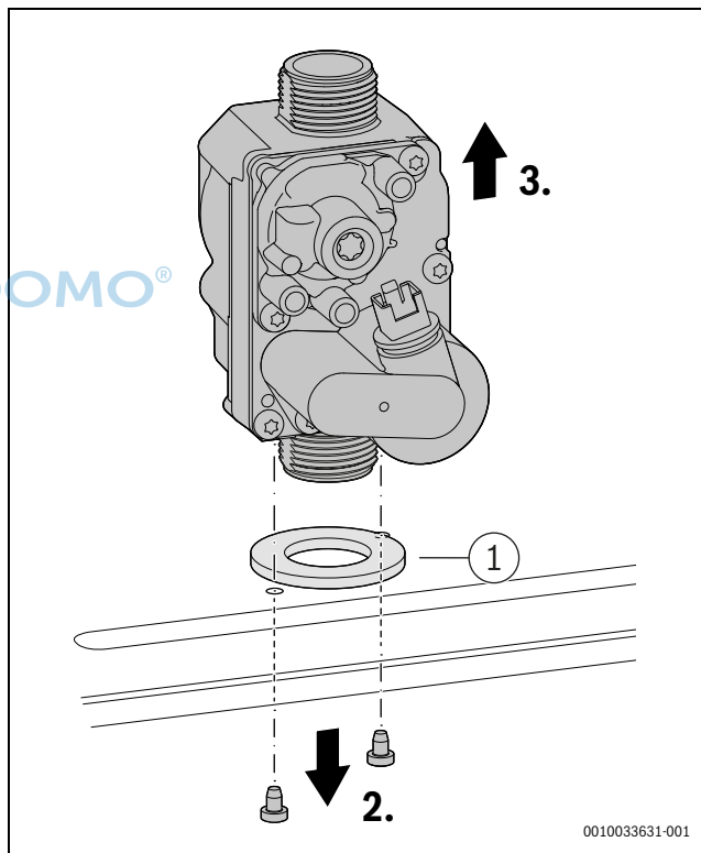
Bild 34 Gasarmatur ausbauen
