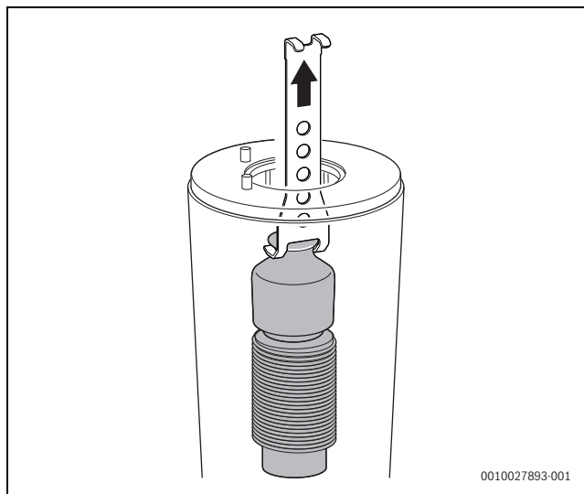
Bild 17 Oberen Verdrängungskörper herausnehmen
