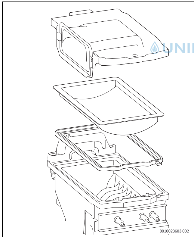
Bild 11 Brenner
