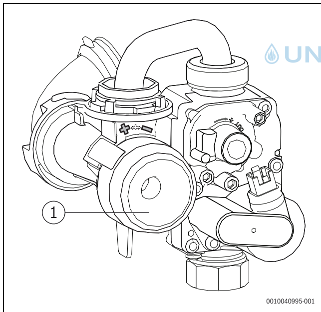
Bild 3 Gas-Luft-Verhältnis einstellen
