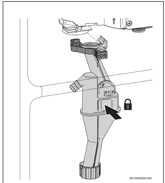
Bild 19 Kondensatsiphon einsetzen
