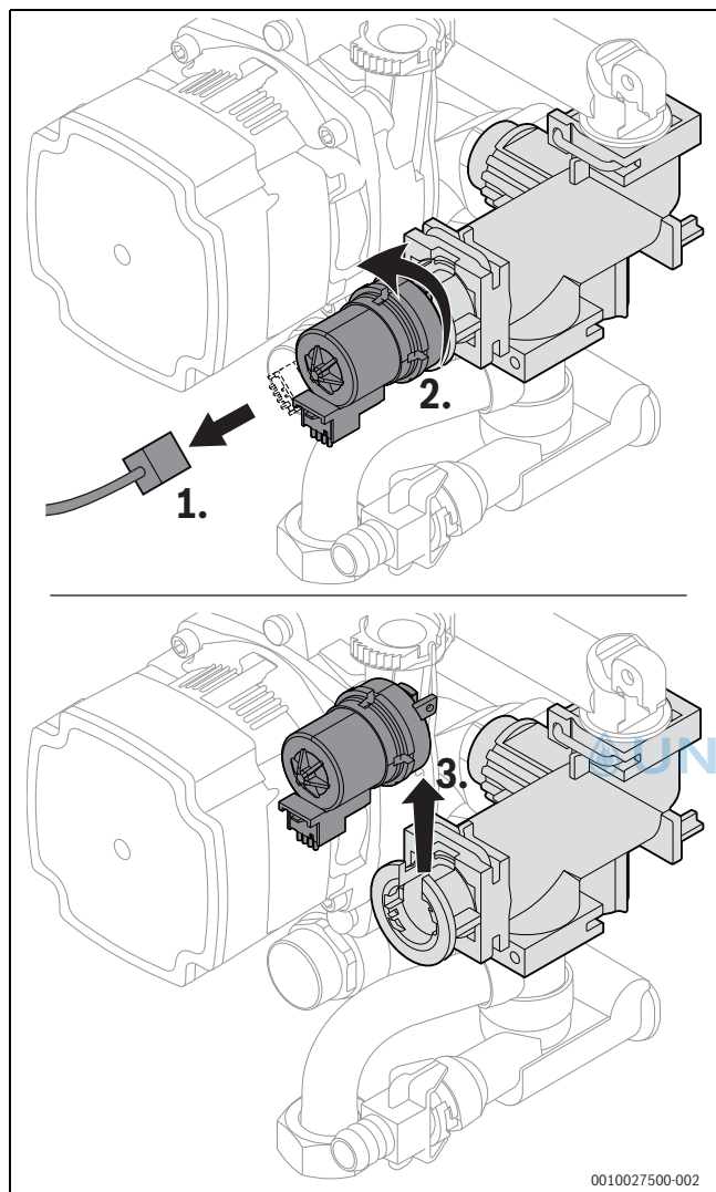
Bild 20 Motor am 3-Wege-Ventil ausbauen (Variante ohne Schrauben)
