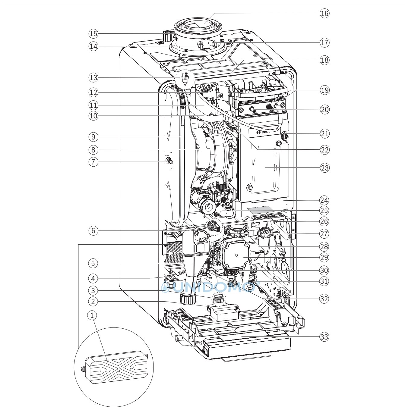
Bild 1 Produktübersicht Kombigerät
