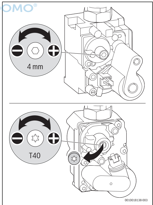
Bild 5 CO 2 - oder O 2 -Gehalt einstellen
