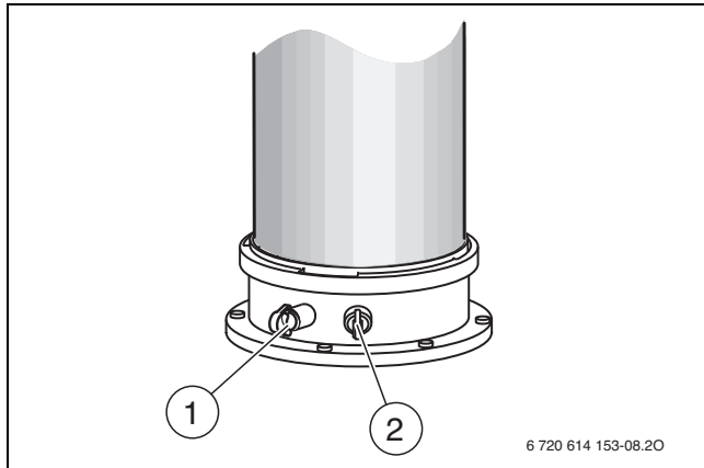
Bild 7 Abgasmessstutzen und Verbrennungsluft-Messstutzen
