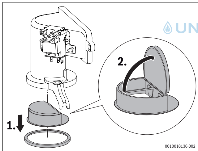
Bild 14 Rückschlagklappe in der Mischeinrichtung
