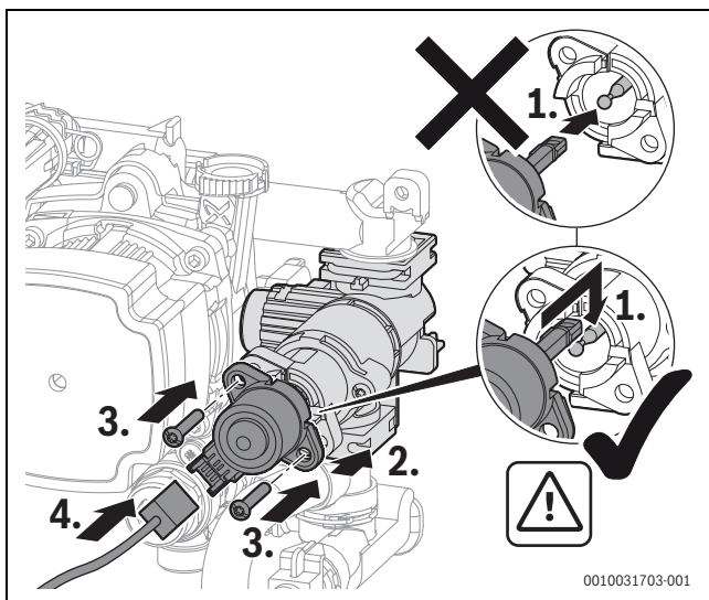
Bild 23 Motor am 3-Wege-Ventil einbauen (Variante mit Schrauben)
