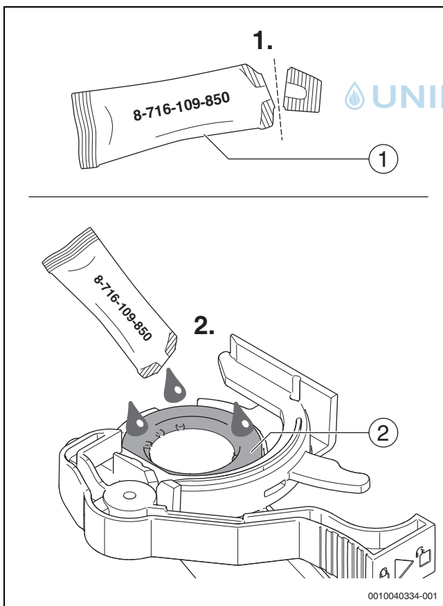
Bild 18 Dichtung fetten
