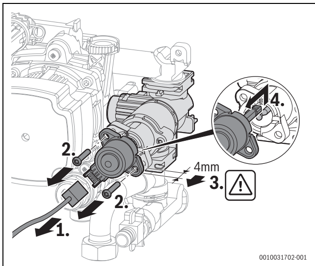
Bild 22 Motor am 3-Wege-Ventil ausbauen (Variante mit Schrauben)
