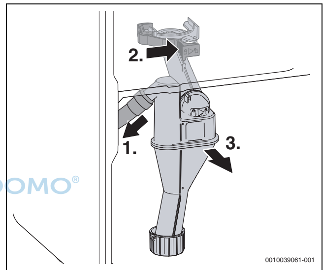
Bild 15 Kondensatsiphon ausbauen
