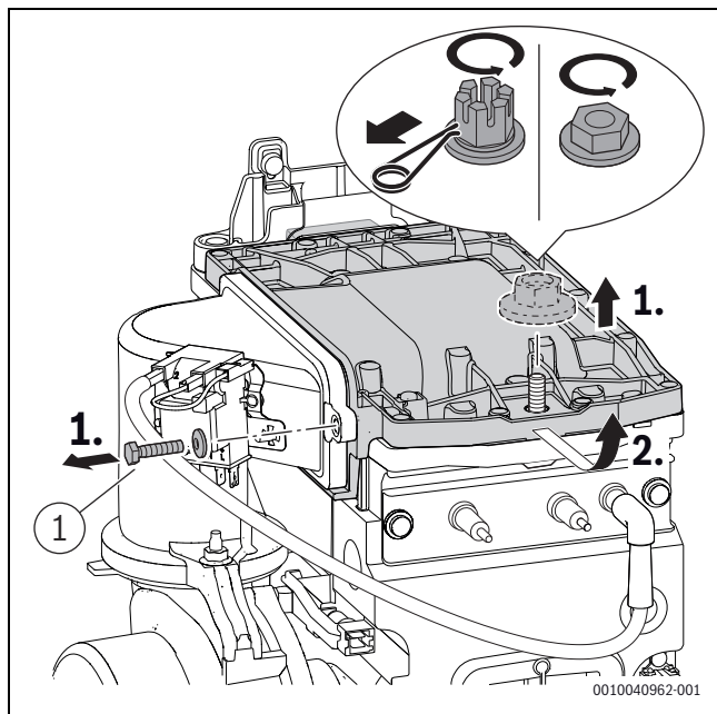
Bild 10 Brennerdeckel ausbauen
