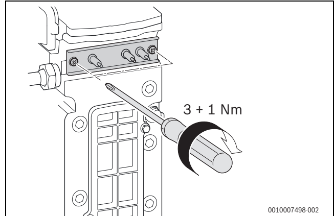
Bild 8 Elektroden-Set montieren
