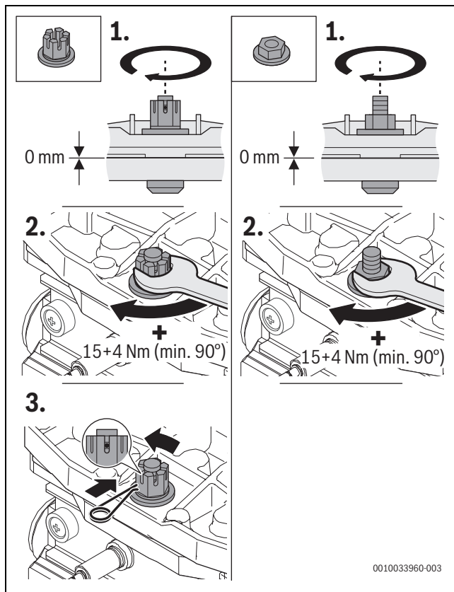
Bild 12 Mutter am Brennerdeckel festziehen
