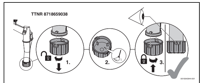
Bild 16 Schmutzfänger reinigen
