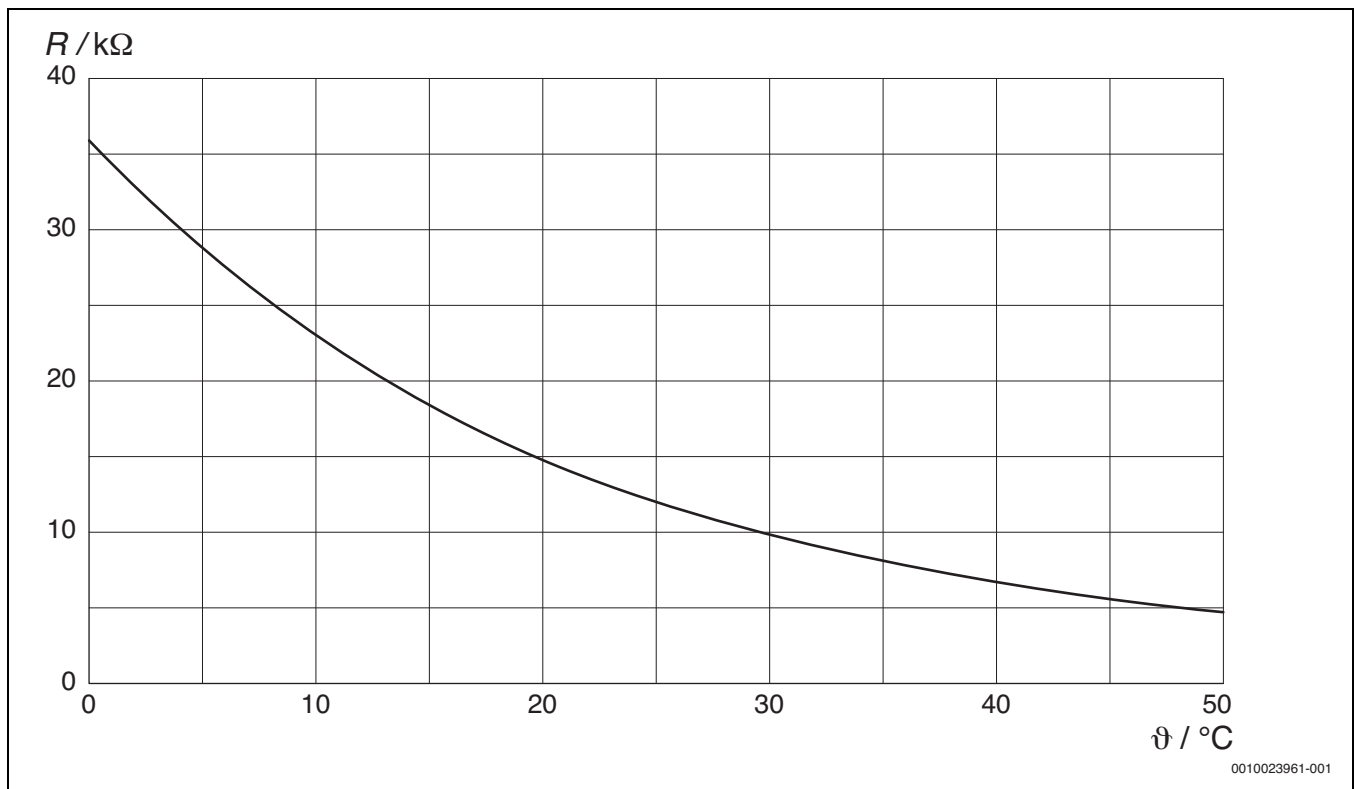
Bild 53 Widerstandskennlinie Temperaturfühler
