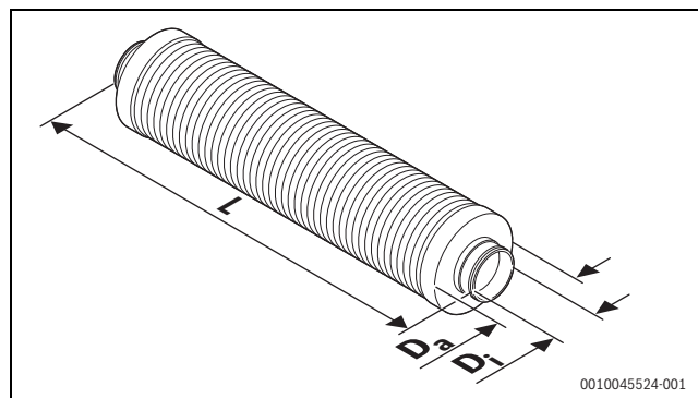
Bild 94 Schalldämpfer SDF... (Maße in mm)
