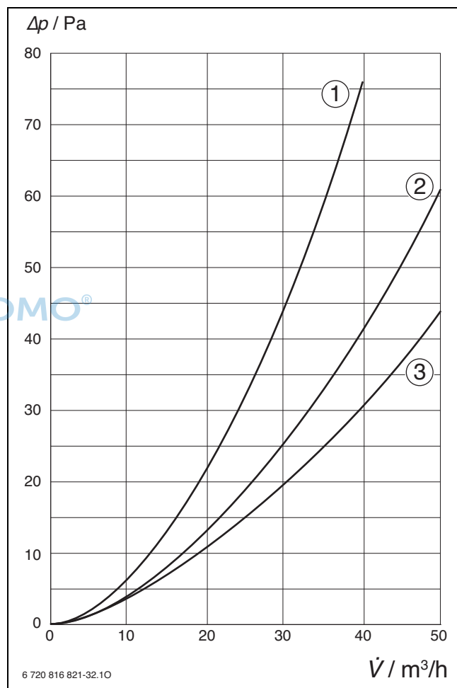
Bild 206 Druckverlust
