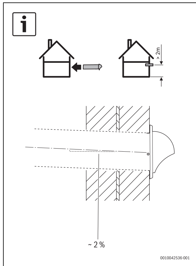
Bild 90 Einbausituation
