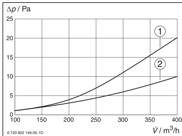
Bild 88 Druckverluste Wanddurchführung WGE 160-2, mit Anschluss DN 160
