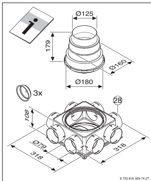
Bild 112 VK 125-1-8 (Maße in mm)
