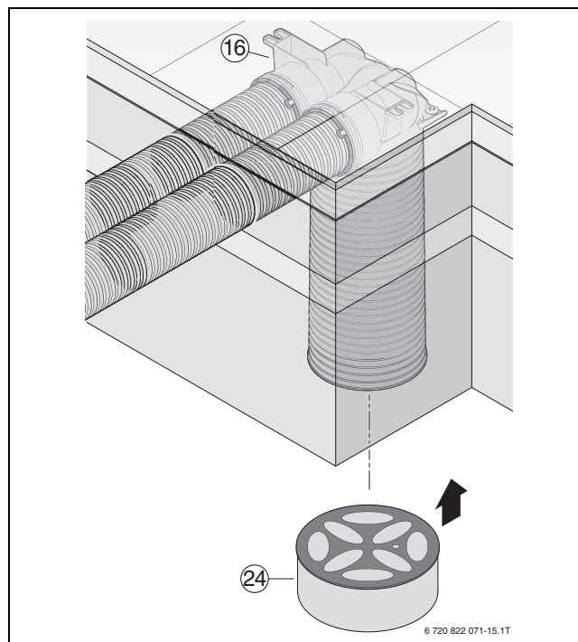
Bild 192 SDE – Anwendungsbeispiel
