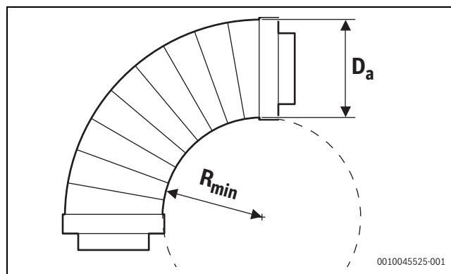
Bild 95 Kleinster Biegeradius Schalldämpfer SDF...
