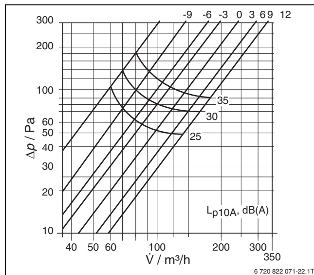
Bild 190 Strömungsgeräusche AV 125 bei Stellung des Ventilkonus S
