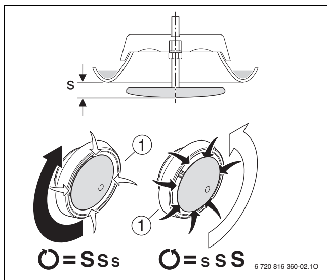
Bild 188 Luftmengen-Feineinstellung
