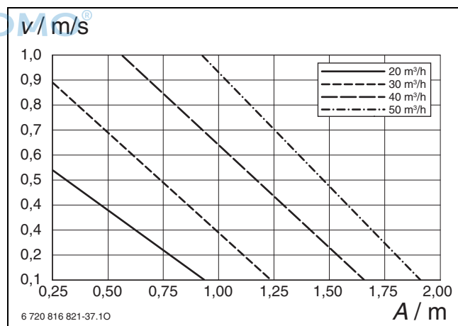
Bild 198 Wurfweite bei verschiedenen Volumenströmen
