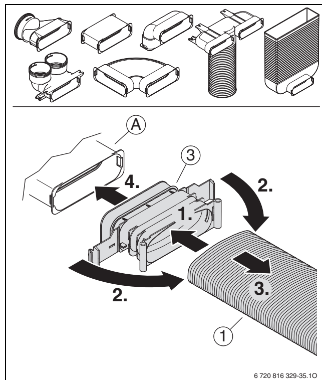
Bild 166 FK 140 + FKV.../FKB.../FKU.../RRB 75-3
