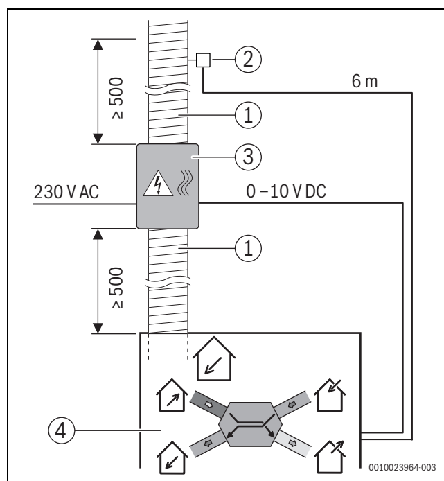
Bild 49 Position Nachheizregister HRE-A 160-1200
