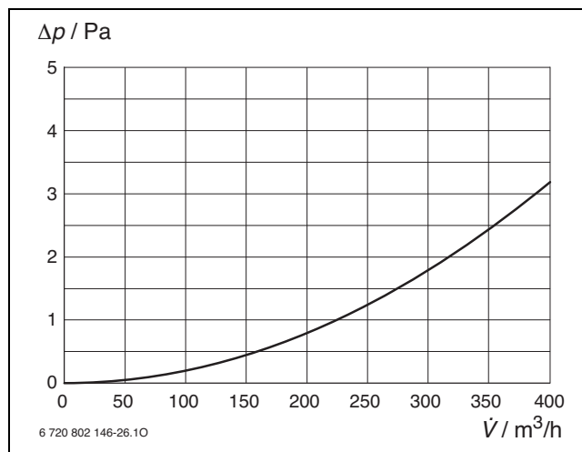
Bild 69 Druckverlust BEPP 160-1
