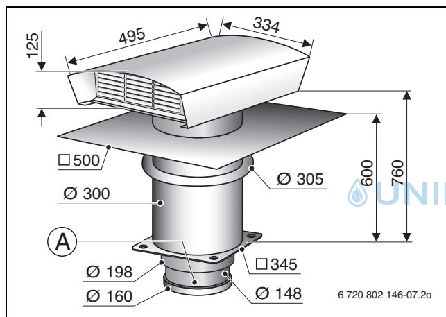
Bild 82 Abmessungen Dachdurchführung DDF 160/1 (Maße in mm)
