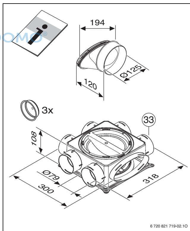
Bild 113 VK 125-1S (Maße in mm)
