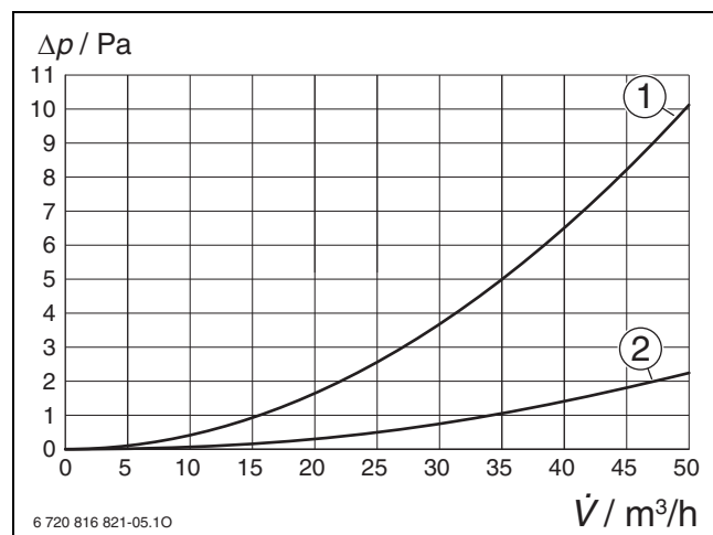
Bild 160 Druckverlust FKU 140-3 – Zuluft
