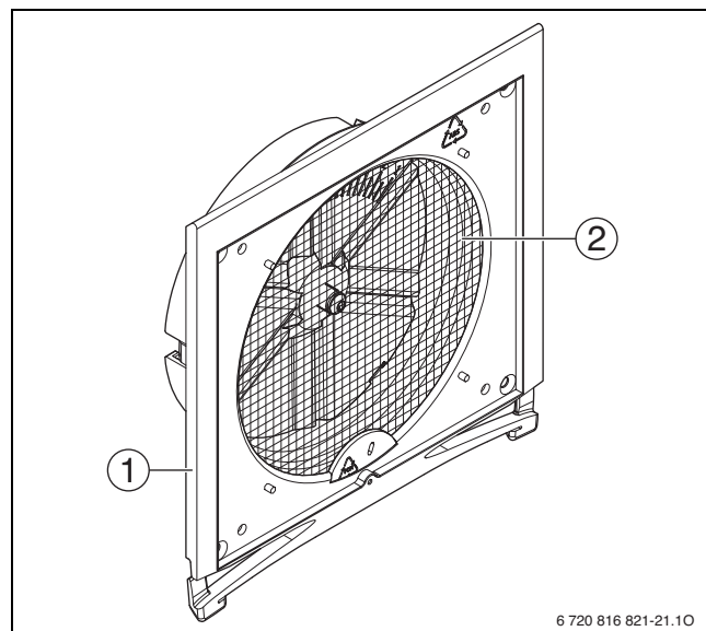
Bild 194 Luftdurchlass Wand/Decke
