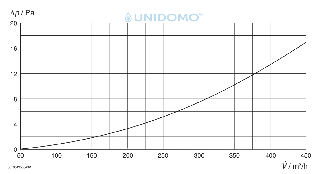
Bild 54 Kennlinie Druckverlust/Volumenstrom
