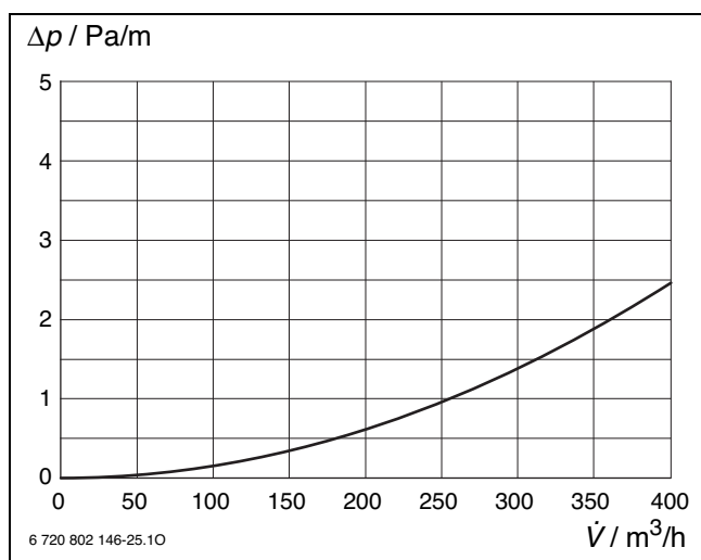
Bild 71 Druckverlust DEPP 160-3
