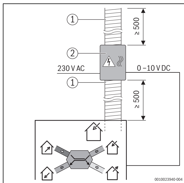
Bild 48 Position zusätzliches Vorheizregister HRE 160-1200
