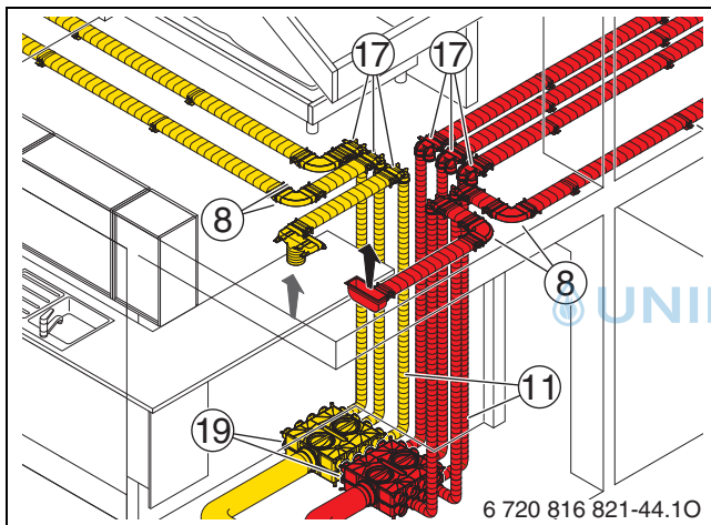
Bild 97 Luftverteilung-Kanalsystem
