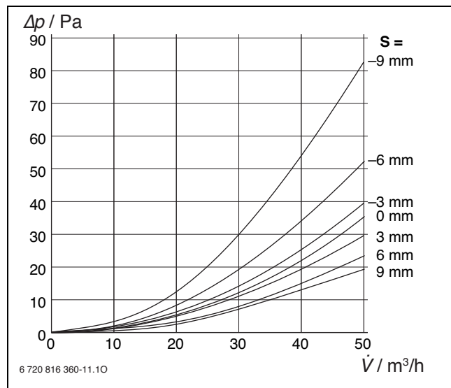
Bild 189 Druckverlust AV 125
