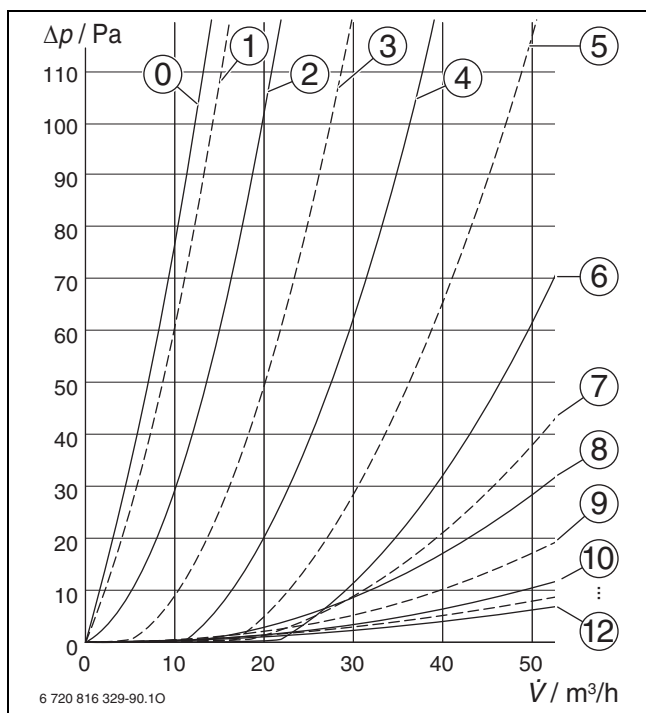
Bild 130 Druckverlust Volumenstromdrossel VKD-E
