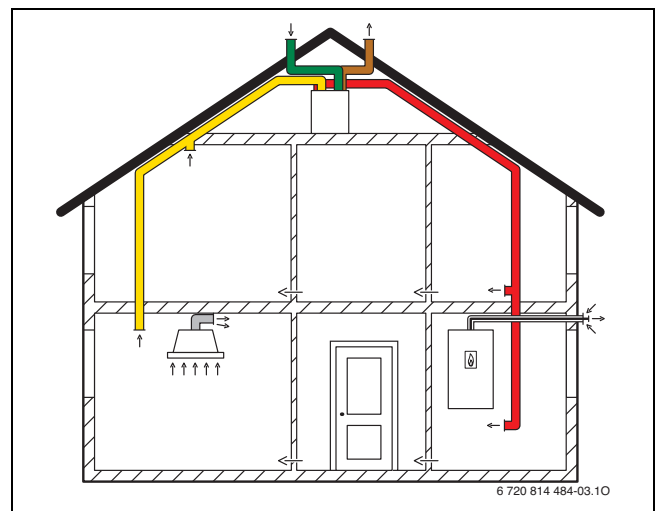
Bild 215 Ventilator 5000 C und raumluftunabhängige Feuerstätte
