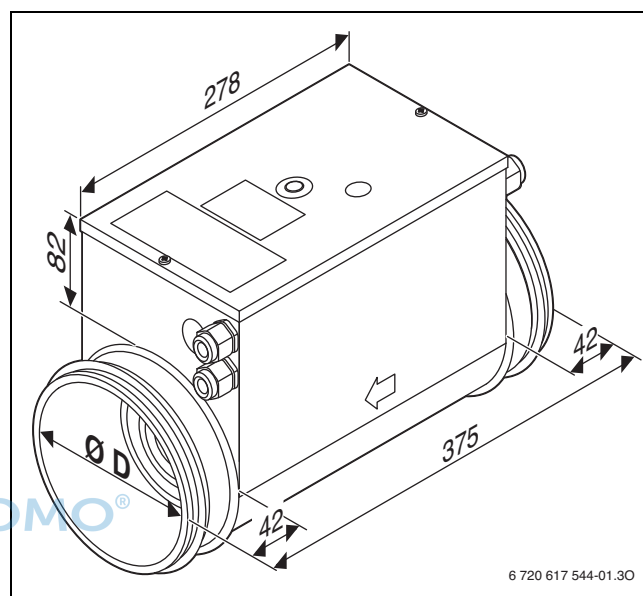
Bild 52 Einbaumaße der Heizregister (Maße in mm)
