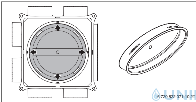
Bild 107 Revisionsdeckel
