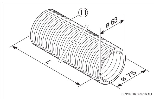
Bild 133 RR 75-1/2 (Maße in mm)
