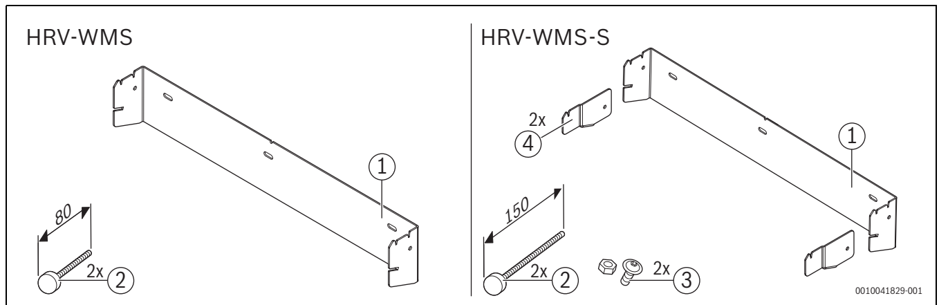
Bild 16 Lieferumfang HRV-WMS/HRV-WMS-S
