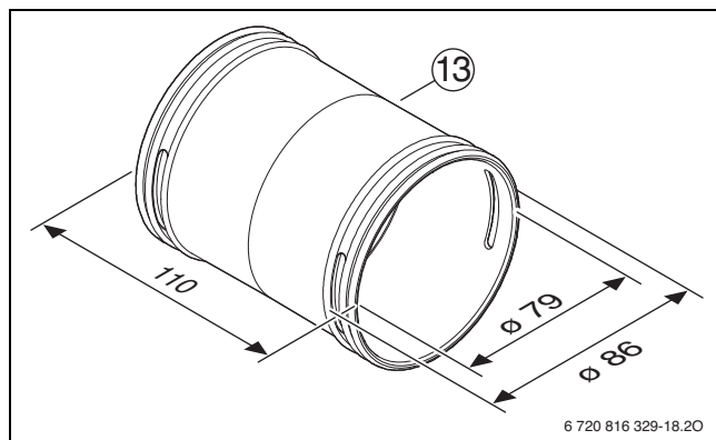
Bild 148 RRV 75-2 (Maße in mm)
