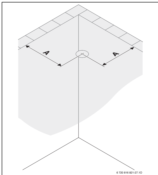
Bild 179 Mindestabstände bei Deckeninstallation
