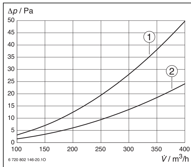
Bild 84 Druckverluste Dachdurchführung DDF 160/1 Anschluss DN 160
