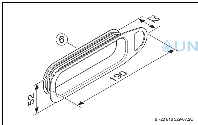
Bild 168 FKS 140 (Maße in mm)
