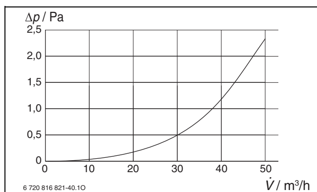
Bild 193 Druckverlust SDE
