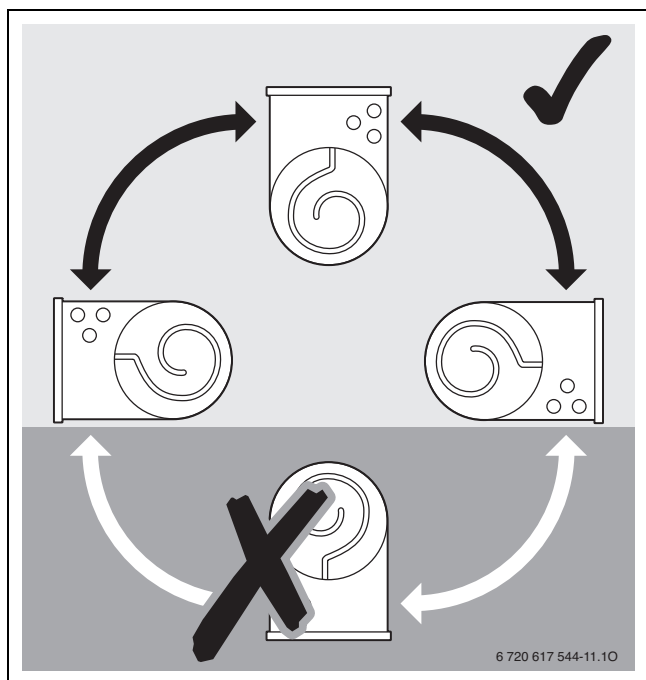
Bild 50 Einbaulagen Heizregister
