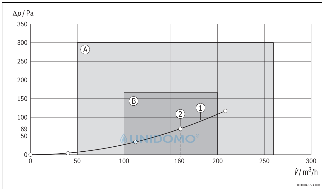
Bild 233 Kennlinien Druckerhöhung/Volumenstrom V5001C 260
