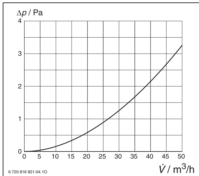
Bild 157 Druckverlust FKB 140-2
