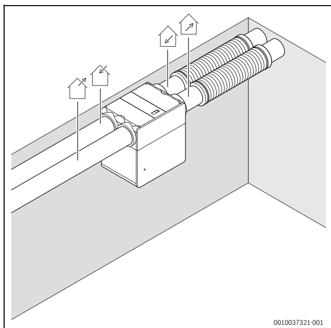
Bild 58 Variante 2: Geräteanschlüsse waagerecht - Luftführung Variante B
