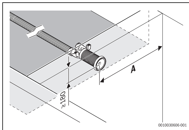
Bild 181 Mindestabstände bei Wandinstallation bei Verwendung von geradem Ventilanschluss RRU 75-5
