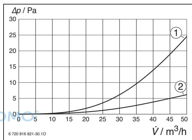
Bild 176 Druckverlust RRU 75-2 mit Luftgitter AG/...
