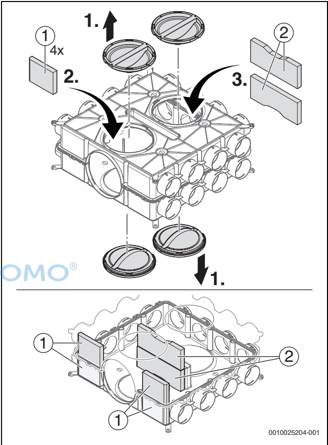
Bild 118 Montage Schalldämmset SDE VK 160
