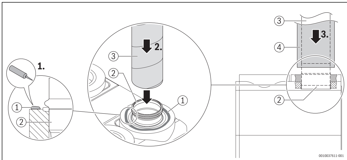
Bild 56 Wickelfalzrohr und Dämmung montieren
