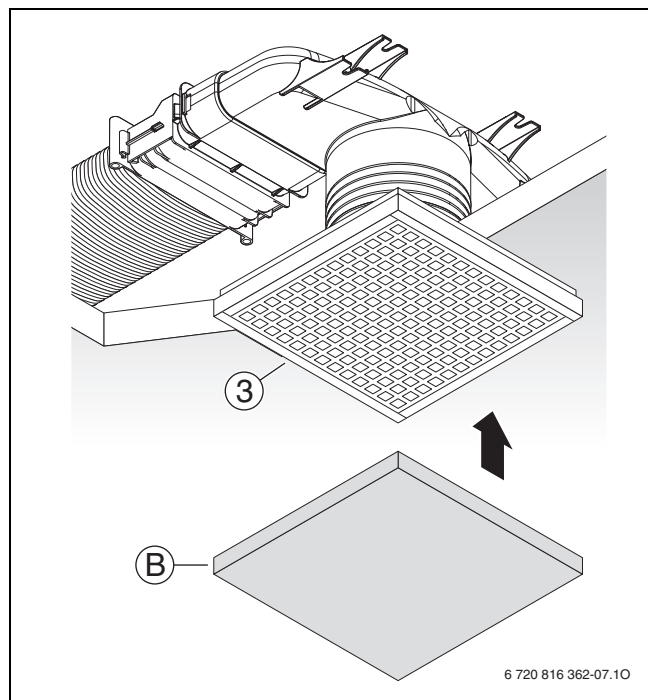
Bild 214 Blende
