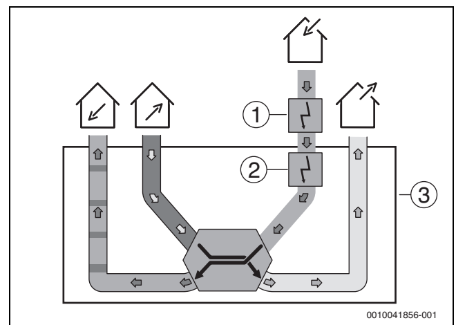
Bild 45 Lüftungsgerät mit zusätzlichem elektrischem Vorheizregister
