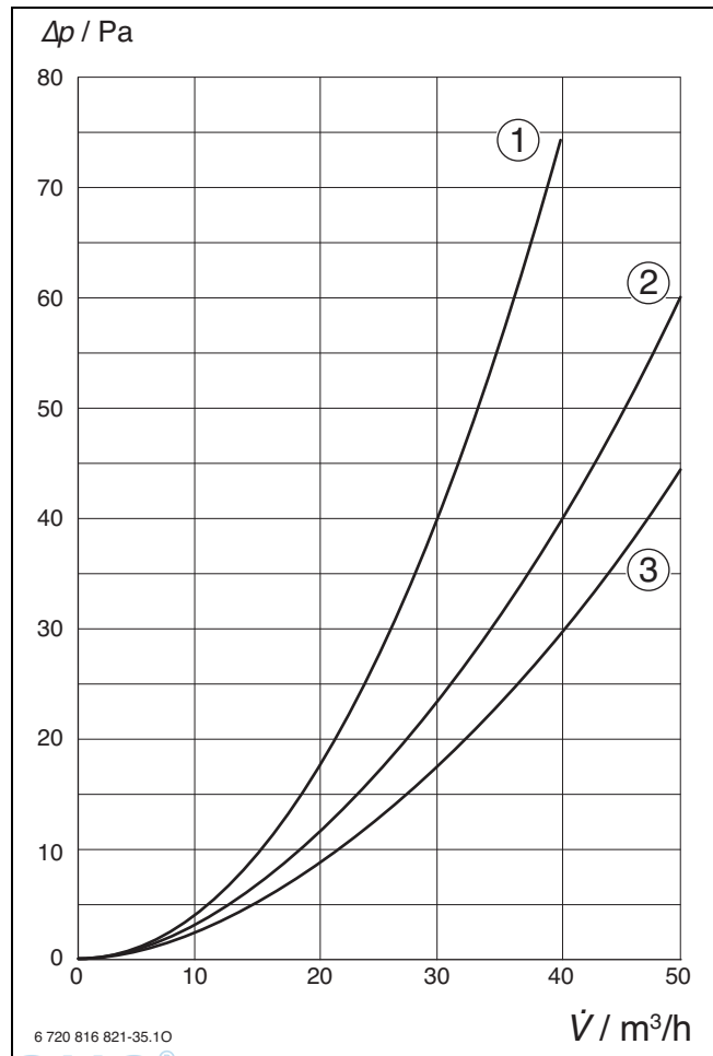
Bild 210 Druckverlust
