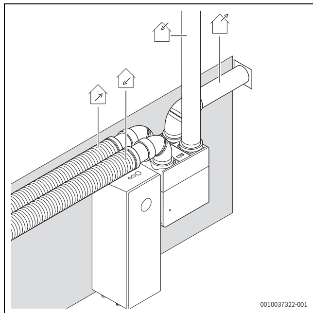
Bild 59 Variante 3: Geräteanschlüsse senkrecht - Luftführung Variante A
