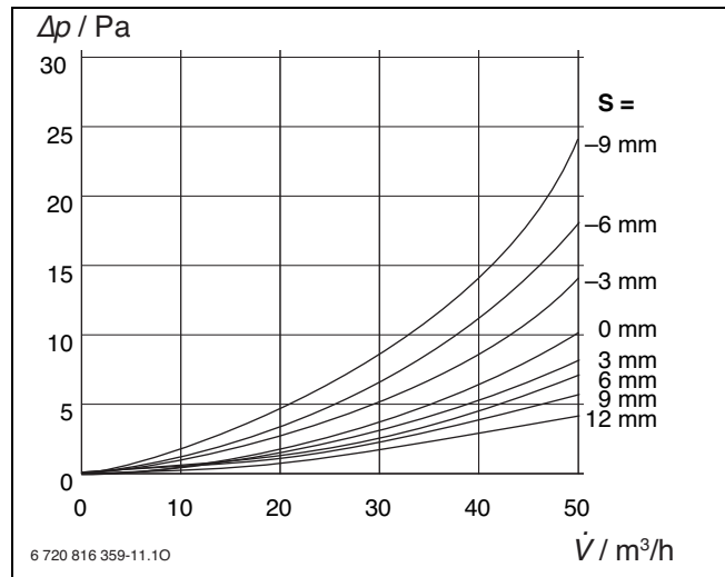
Bild 185 Druckverlust ZU 125
