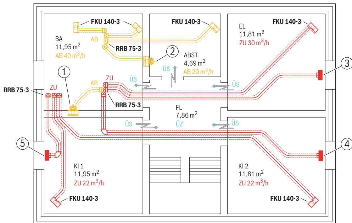
Bild 232 Grundriss Dachgeschoss mit Lüftungsinstallation
