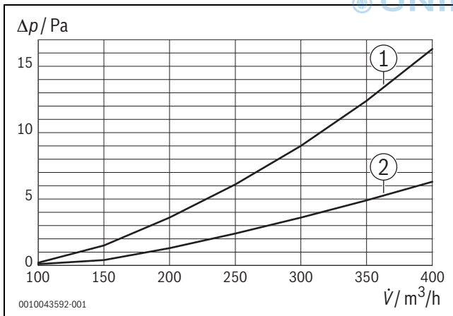
Bild 64 Druckverlust
