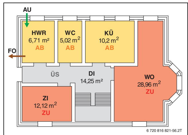
Bild 3 Aufteilung Lüftungsbereiche
