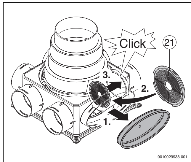
Bild 126 VKD + VK 125-1/VK 125-2V/VK 125-3V
