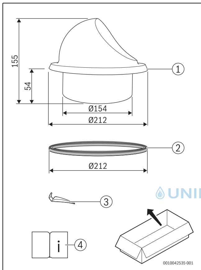
Bild 89 Lieferumfang WGK 160
