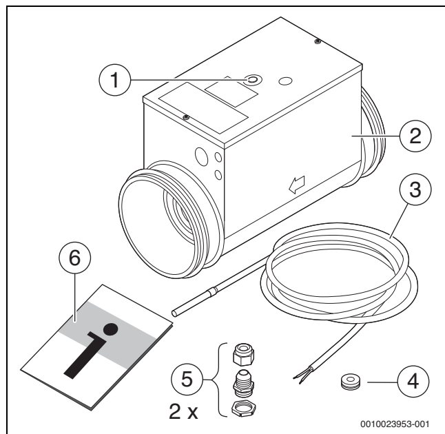
Bild 46 Lieferumfang Nachheizregister HRE-A 160-1200
