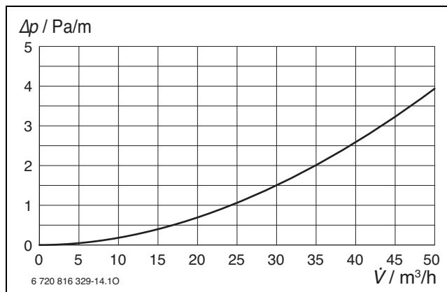
Bild 136 zusätzlicher Druckverlust pro 90°-Bogen Rundkanal RR 75-1/2 – gebogen mit Radius 150 mm
