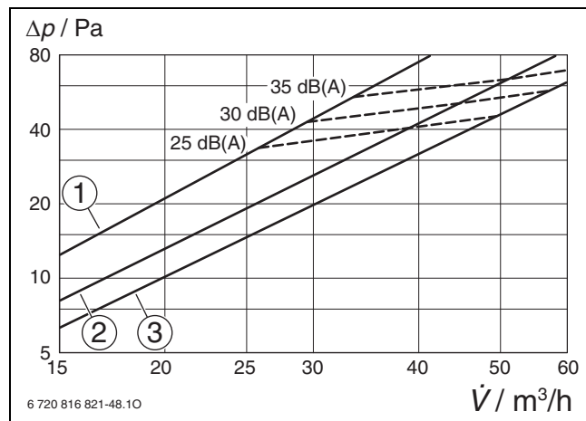
Bild 205 Strömungsgeräusche bei verschiedenen Volumenströmen
