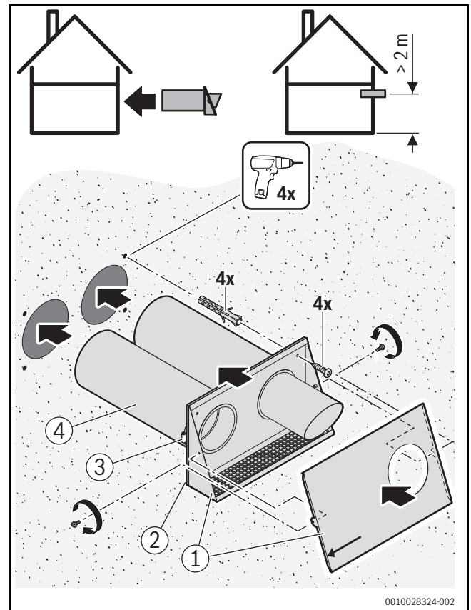
Bild 73 Montagebeispiel
