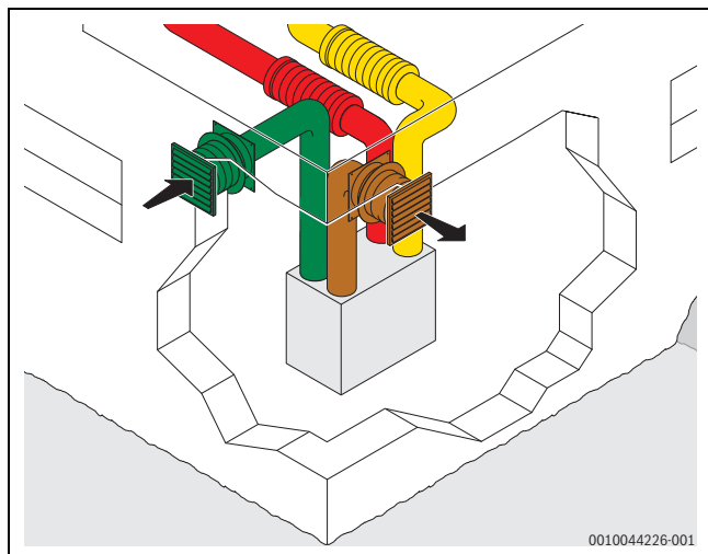
Bild 55 Hauptleitungen
