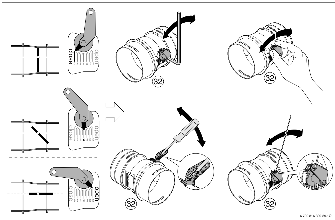
Bild 129 VKD-E einstellen
