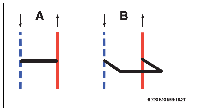
Bild 237 Bypass
