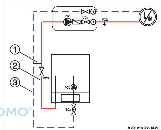
Bild 238 Inneneinheit mit Heizkreis und Bypass
