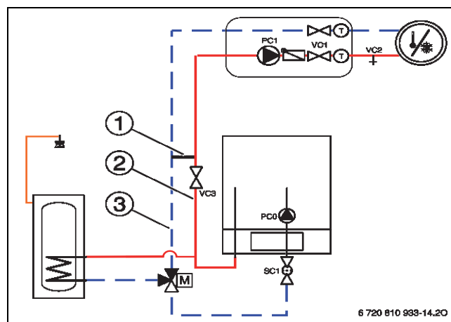
Bild 239 Inneneinheit mit Heizkreis, Warmwasserbereitung und Bypass
