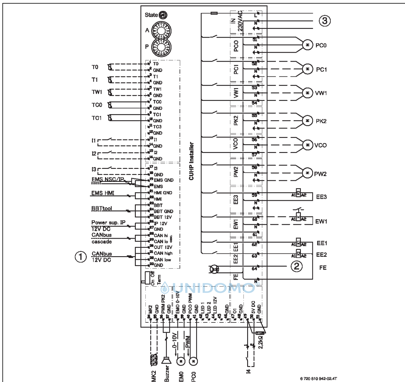
Bild 157 Schaltplan Installationsmodul integrierter elektrischer Zuheizter
