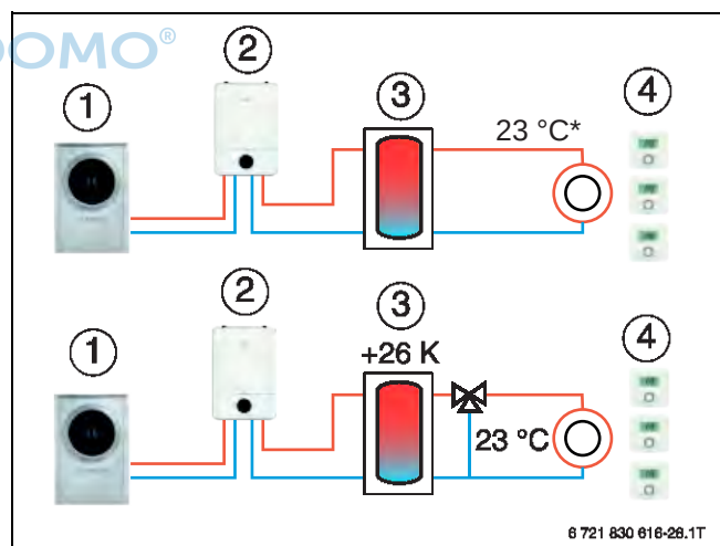
Bild 135 Thermische Speicherung über die Gebäudehülle
