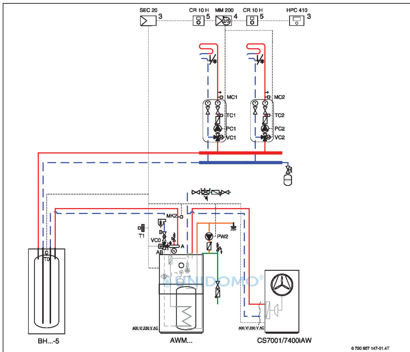
Bild 6 Anlagenschema mit Regelung (unverbindliche Prinzipskizze)
