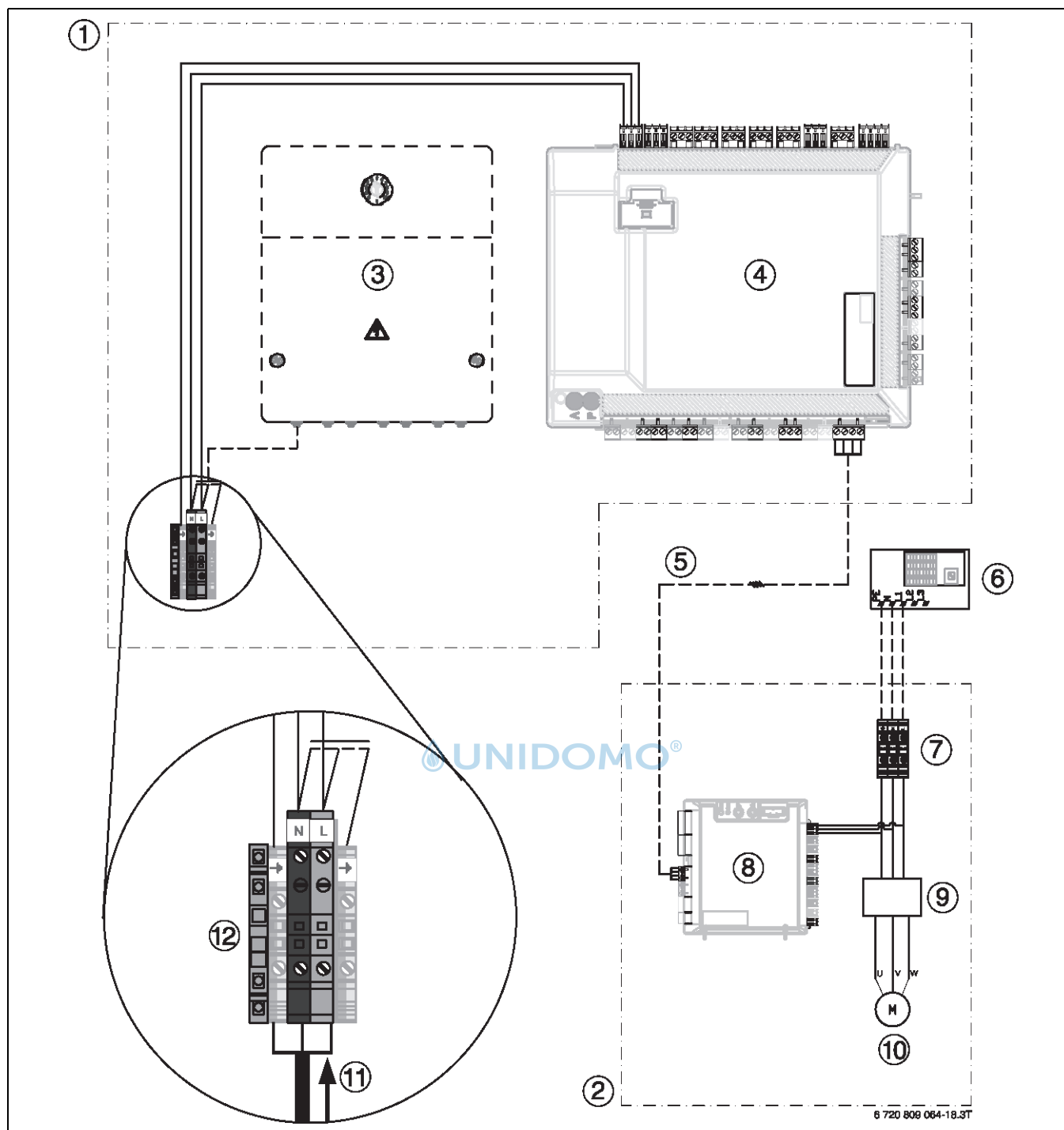
Bild 155 Wärmepumpen-Inneneinheit mit externem Zuheizer – Überblick
