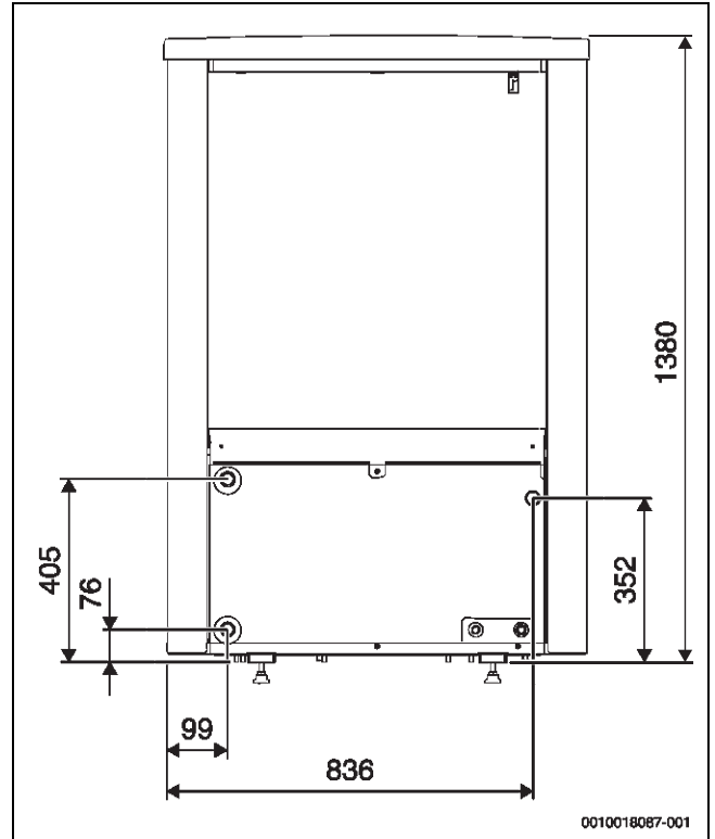
Bild 74 Abmessungen und Anschlüsse der Wärmepumpenmodelle CS7001iAW 5 OR...-S und CS7001iAW 7 OR...-S, Rückseite
