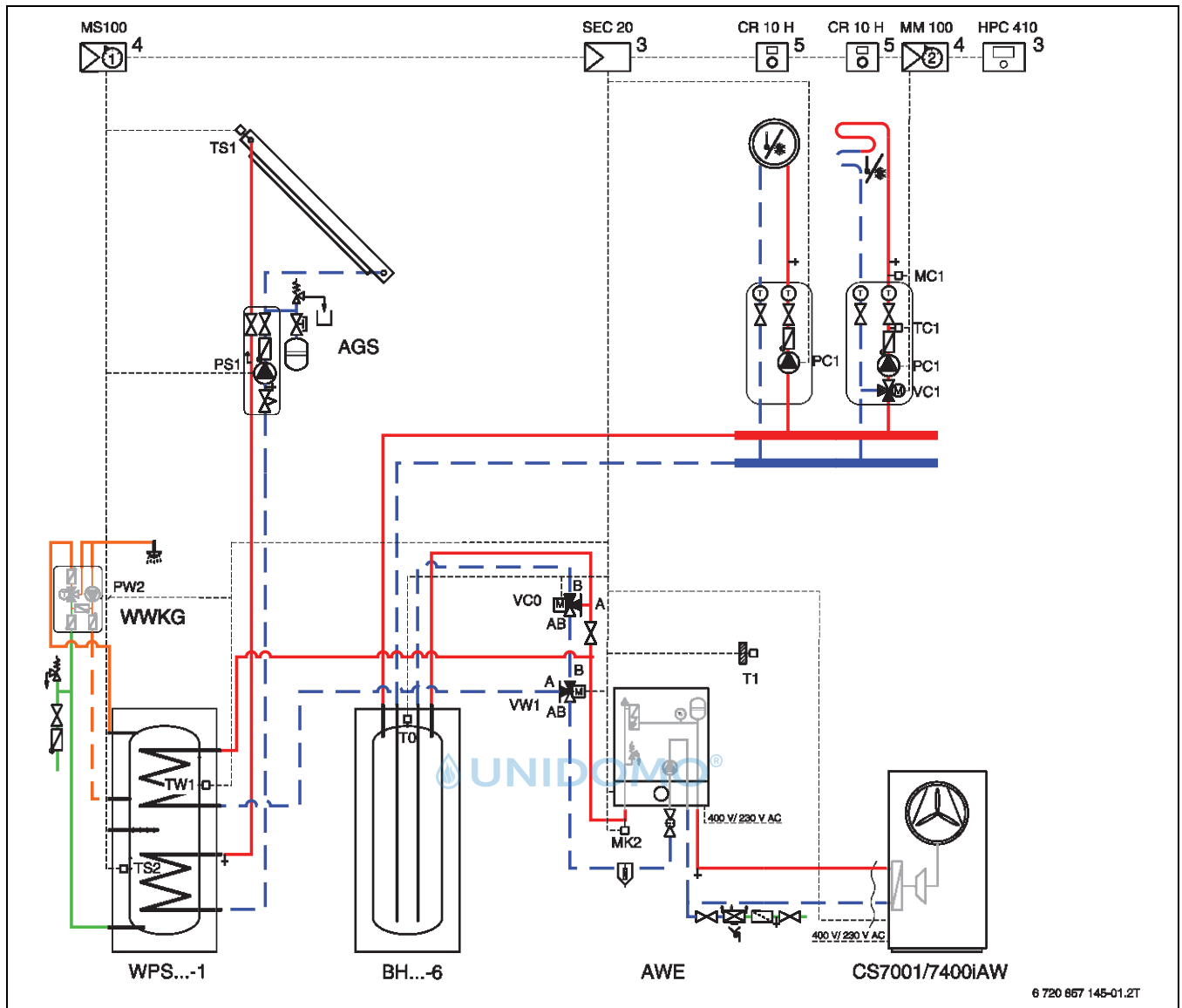
Bild 21 Anlagenschema mit Regelung (unverbindliche Prinzipdarstellung)
