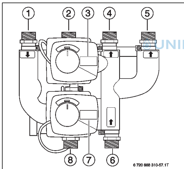
Bild 228 Anschlussgruppe VC0-VW1
