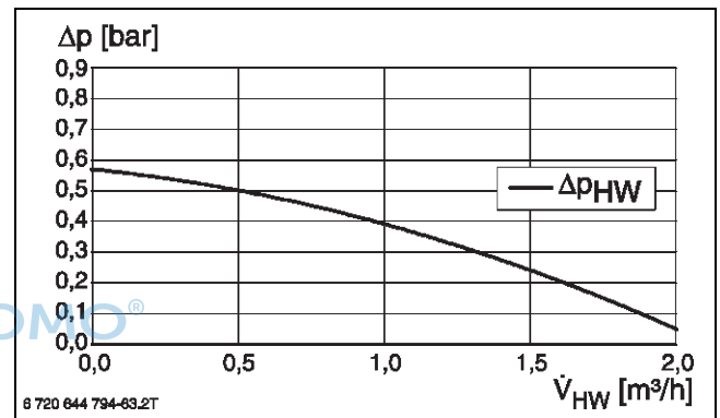
Bild 93 Restförderdruck CS7001iAW 9 OR...-S/CS7000iAW 9 IR...-S
