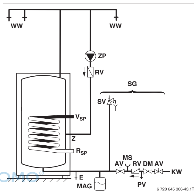
Bild 38 Warmwasserseitiges Anschluss-Schema
