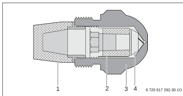
Bild 23 Öl-Druckzerstäuberdüse
