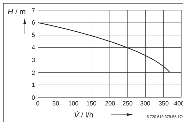
Bild 26 Restförderhöhe Nr. 1620
