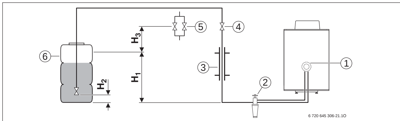
Bild 21 Installationsbeispiel
