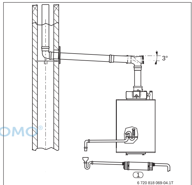
Bild 18 Kondensatableitung aus dem Abgasrohr und dem Öl-Brennwertkessel über die Neutralisationseinrichtung
