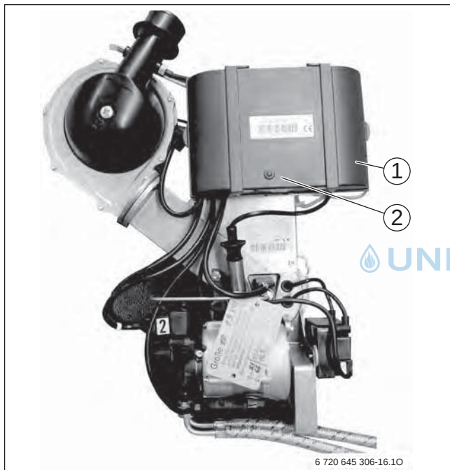
Bild 6 Öl-Blaubrenner
