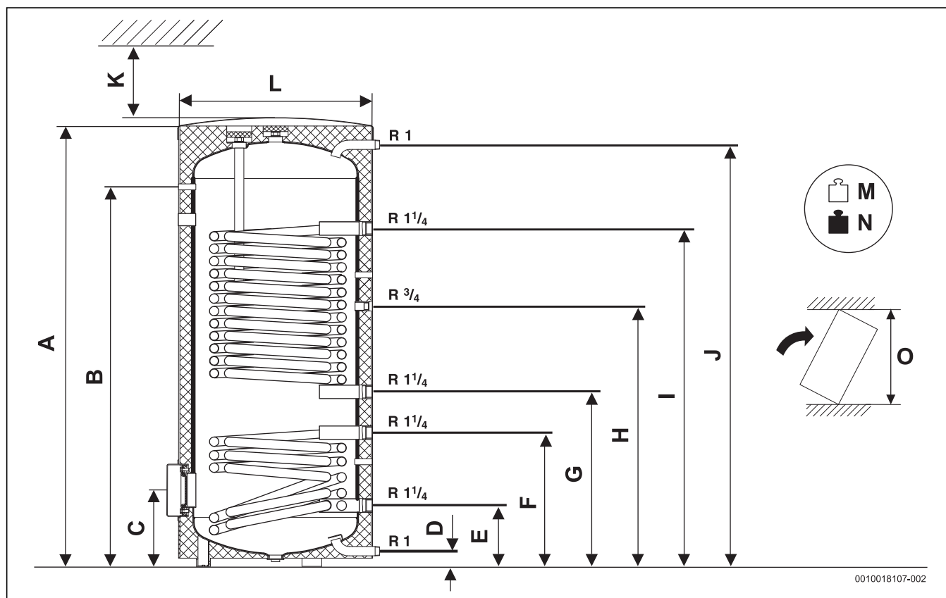
Bild 181 Anschlussmaße und Abmessungen der Solarspeicher WPS 390/490-1 EP
