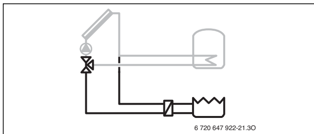
Bild 170 Pool(P)
