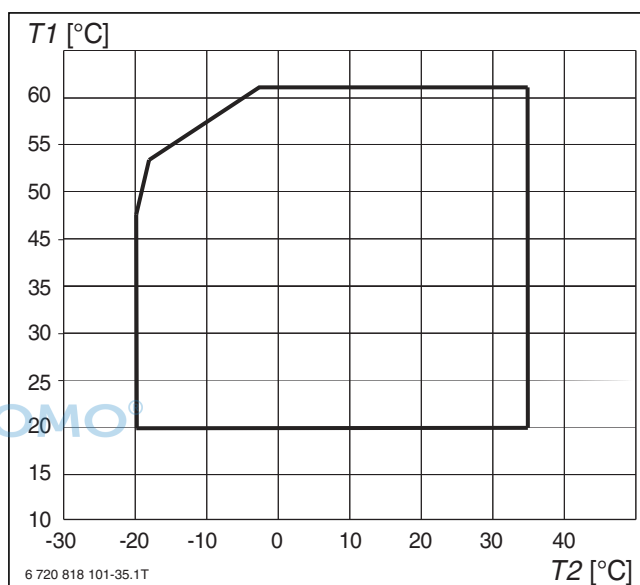
Bild 94 Betriebsbereich ohne Zuheizung
