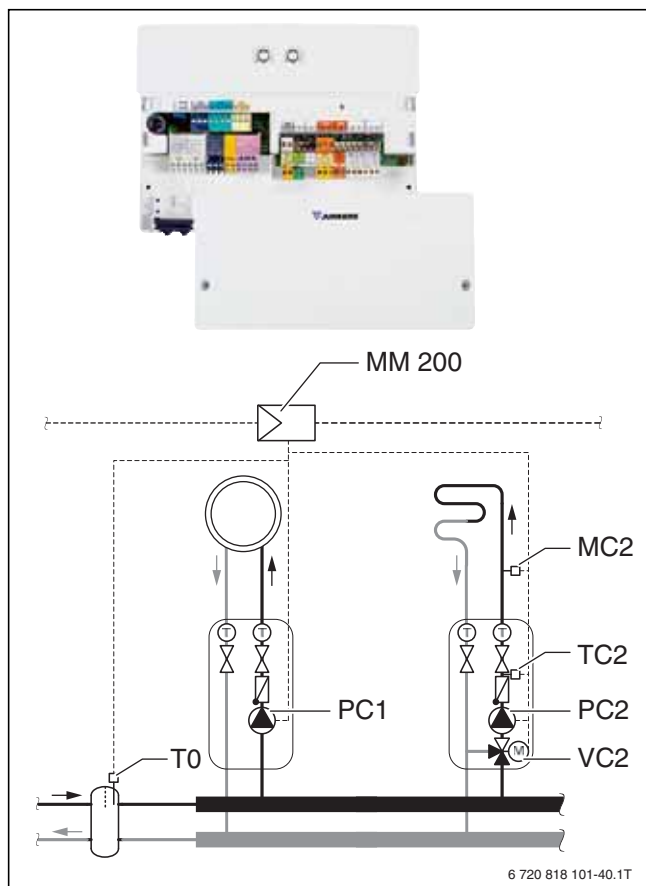
Bild 148 Heizkreismodul MM 200
