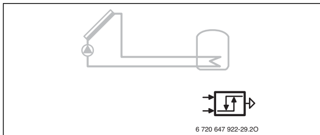
Bild 168 Temperaturdifferenz Regler(M)
