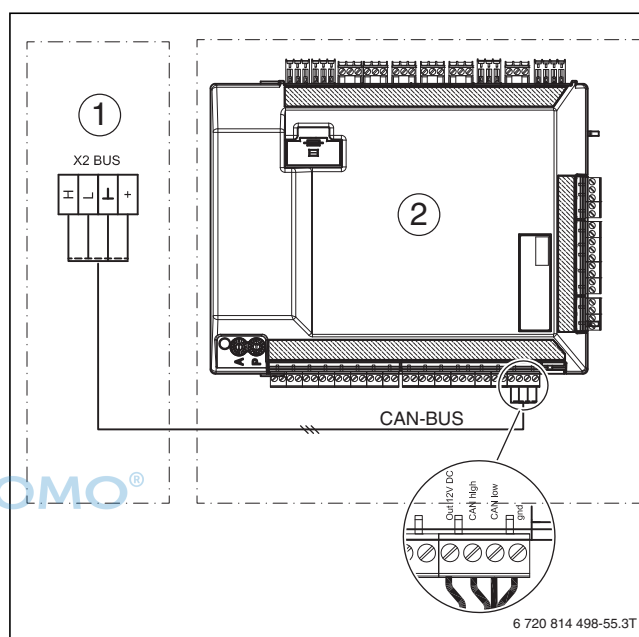
Bild 123 CAN-BUS Verbindung zwischen Wärmepumpeneinheit und Inneneinheit
