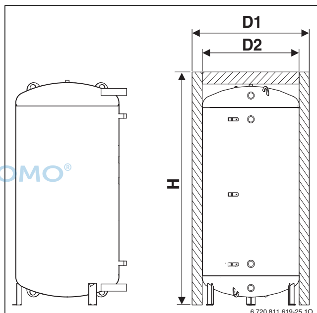
Bild 188 Maße BH ...-6
