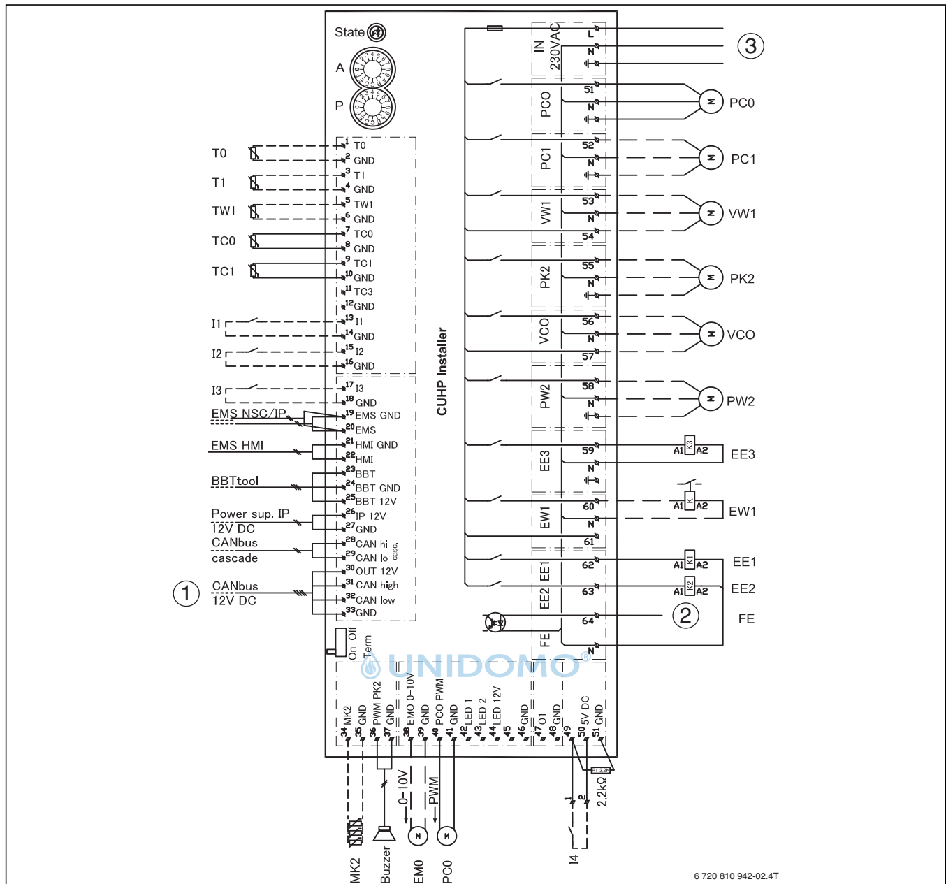
Bild 135 Schaltplan Installationsmodul integrierter elektrischer Zuheizer
