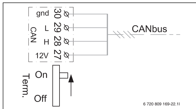
Bild 122 CANbus-Terminierung
