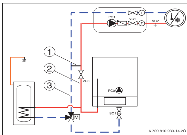
Bild 209 Inneneinheit mit Heizkreis, Warmwasserbereitung und Bypass
