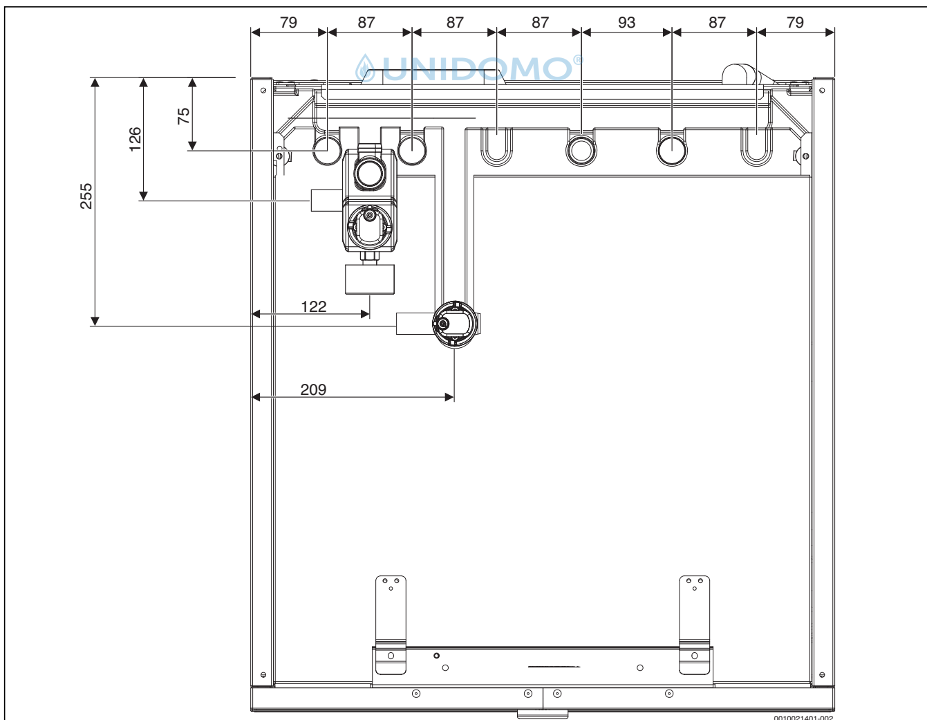
Bild 116 Abmessungen – Draufsicht
