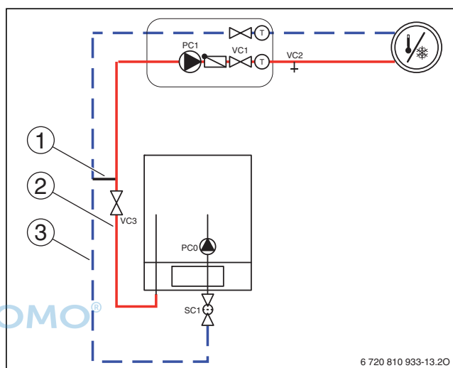
Bild 208 Inneneinheit mit Heizkreis und Bypass
