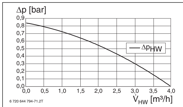
Bild 93 Restförderhöhe CS7000iAW 17 OR-T
