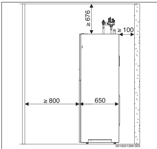
Bild 114 Mindestabstand Inneneinheit
