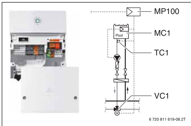
Bild 173 Schwimmbadmodul MP 100
