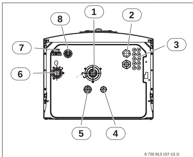
Bild 26 Rohranschlüsse für Inneneinheit mit elektrischem Zuheizer (Ansicht von unten)
