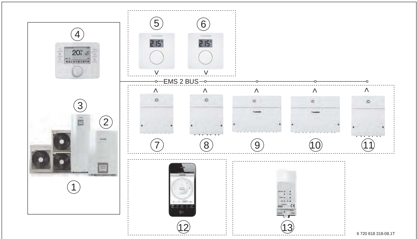
Bild 60 Regelsystem
