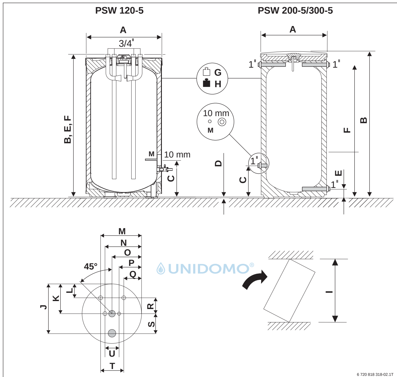
Bild 107 Abmessungen PSW 120/200/300-5
