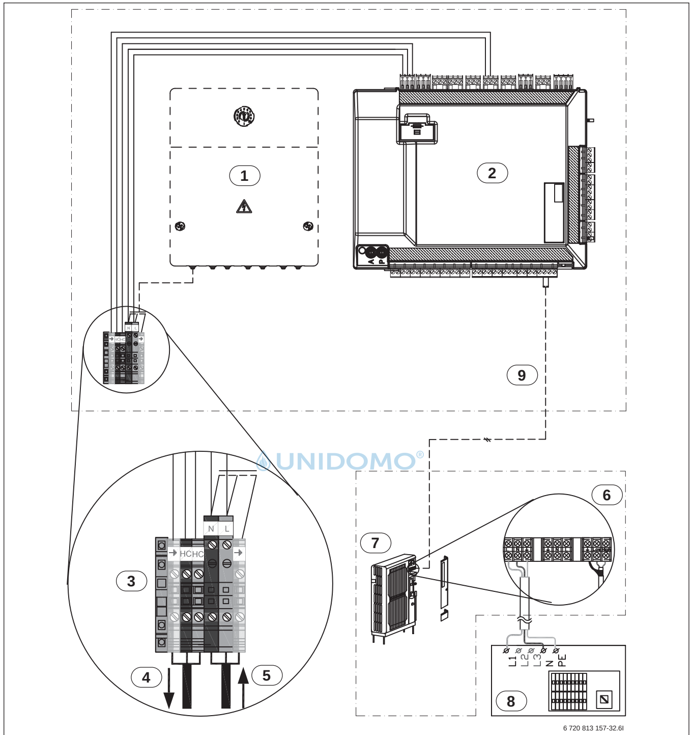
Bild 54 230 V~ 1N Inneneinheit mit 230 V~ 1N Außeneinheit
