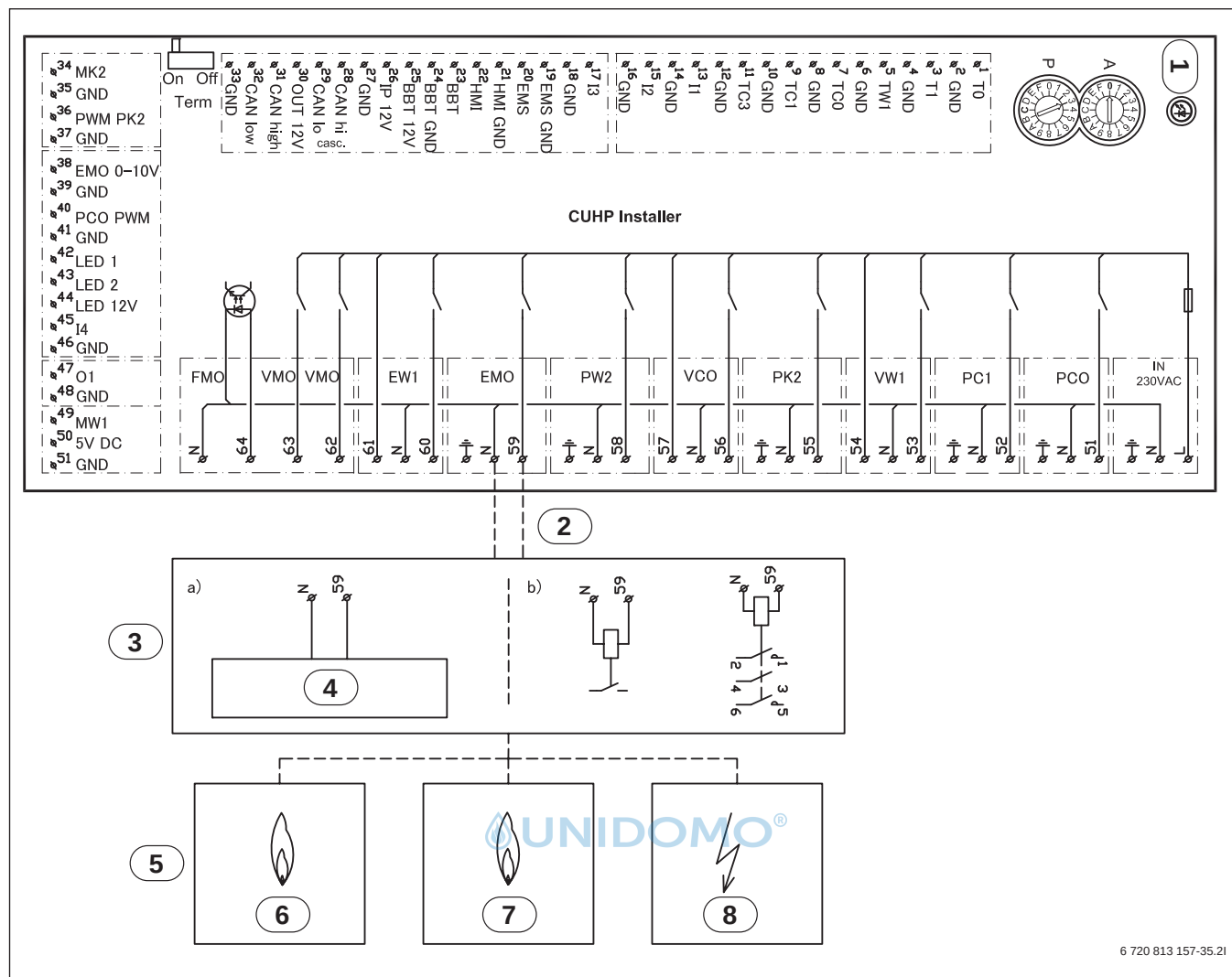
Bild 57 Schaltschema des Installationsmoduls, externen Zuheizer (z. B. Heizkessel) ein-/ausschalten
