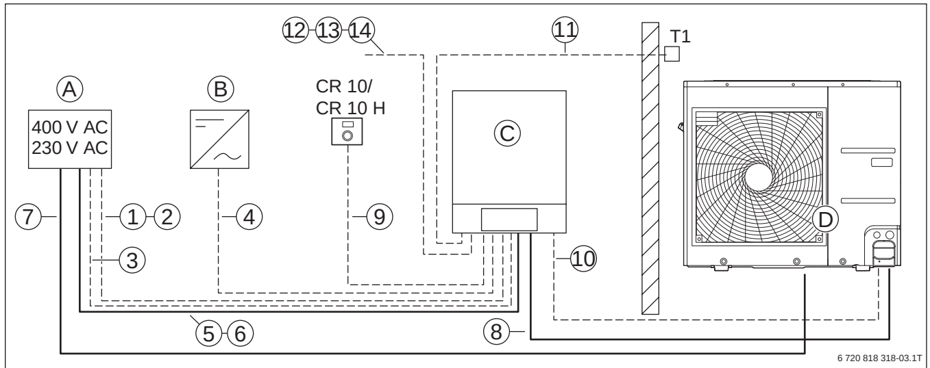
Bild 85 Elektrische Leitungen
