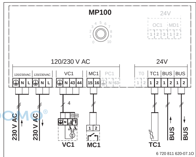
Bild 77 Elektrische Verdrahtung einer Schwimmbadanlage
