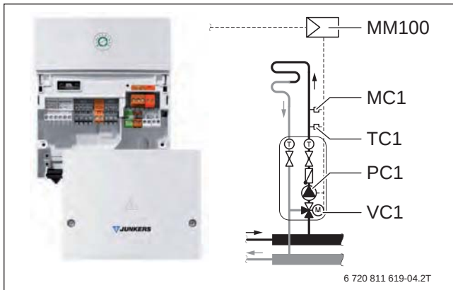
Bild 63 Mischermodul MM 100
