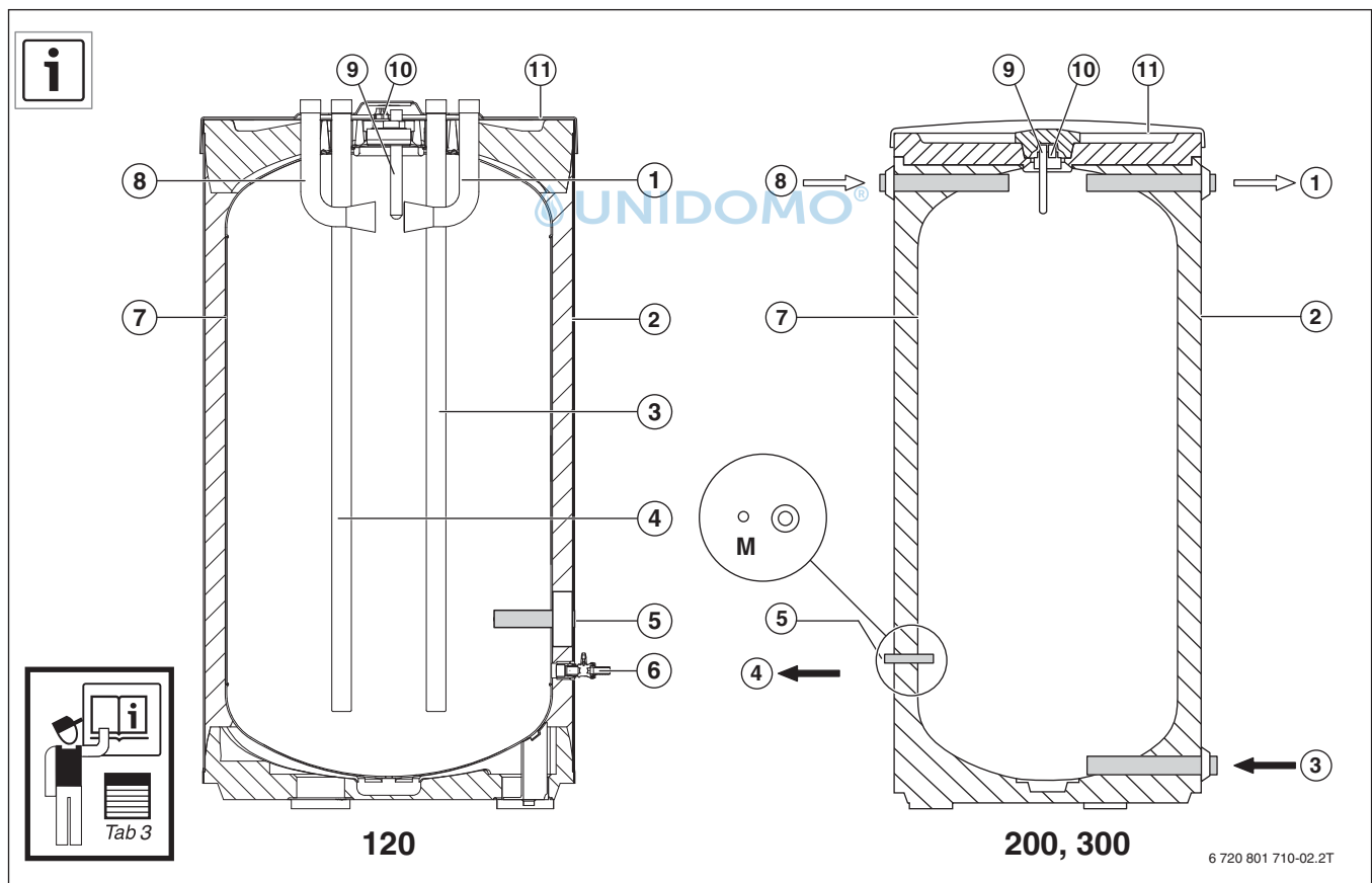
Bild 162 Übersicht PSW 120/200/300-5
