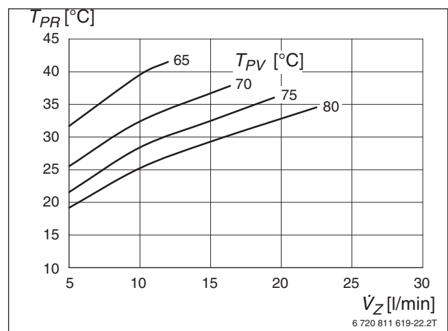
Bild 176 Volumenstrom vom Pufferspeicher (Rücklauf) bei 60 °C Zapftemperatur
