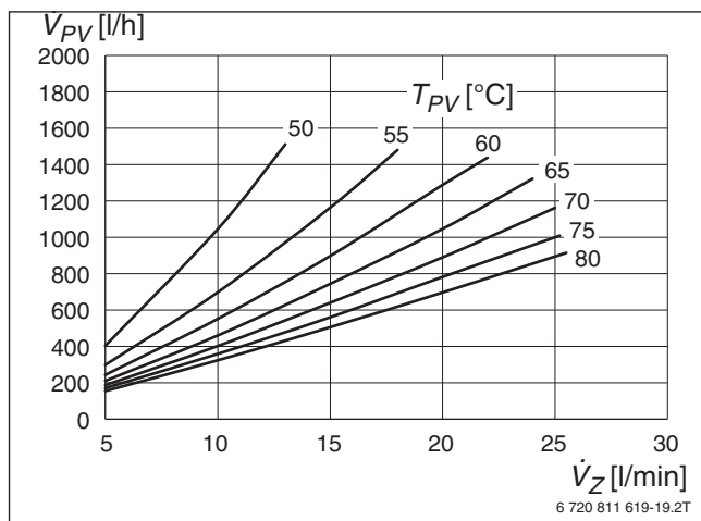
Bild 173 Volumenstrom vom Pufferspeicher (Vorlauf) bei 45 °C Zapftemperatur
