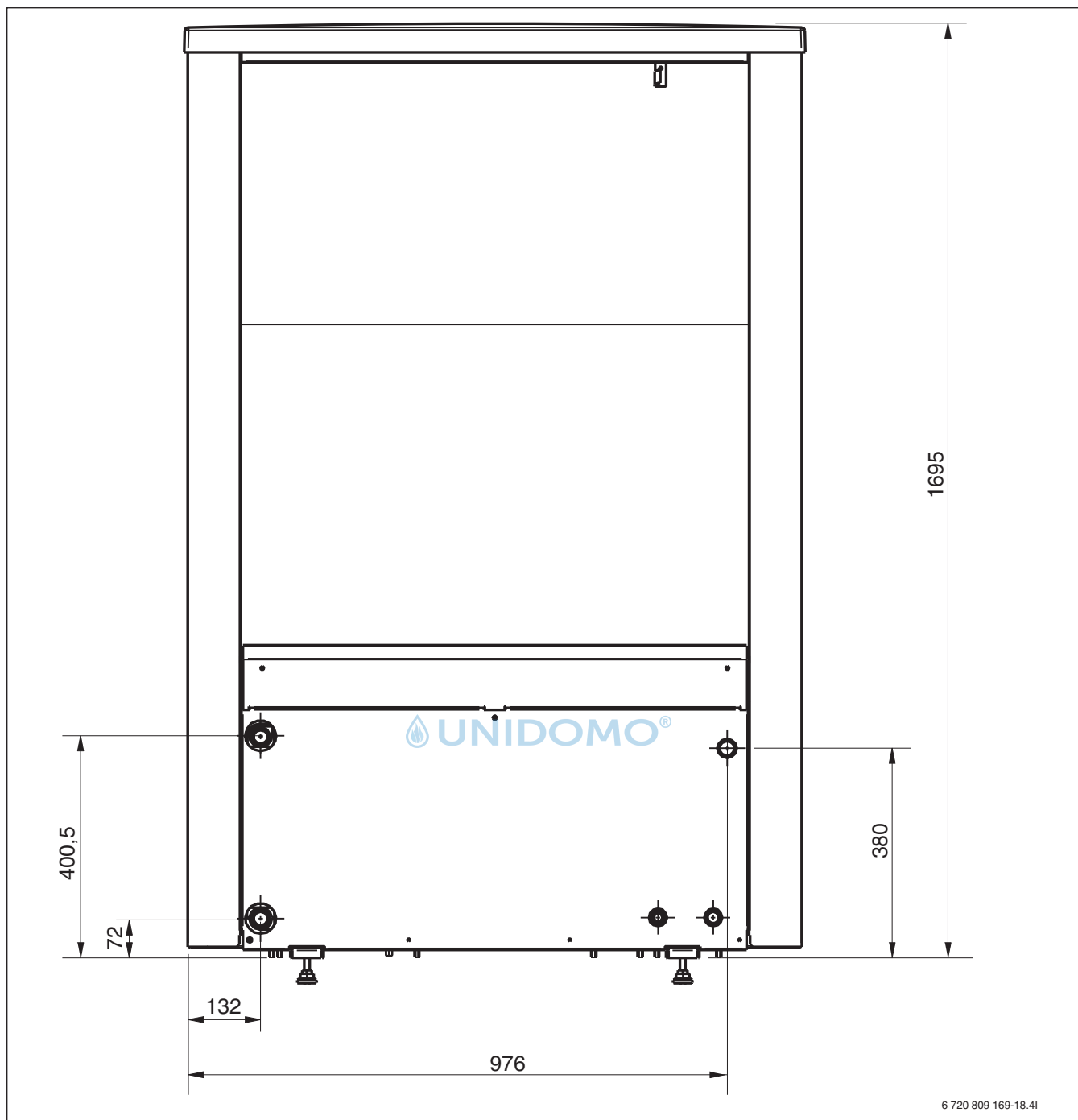
Bild 49 Abmessungen und Anschlüsse der SAO 110-2 / SAO 140-2, Rückseite Bezeichnung der Anschlüsse → Bild 51
