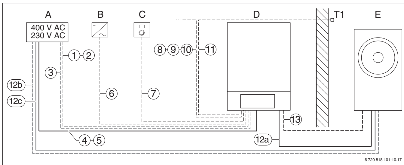
Bild 40 Übersicht über die elektrischen Leitungen
