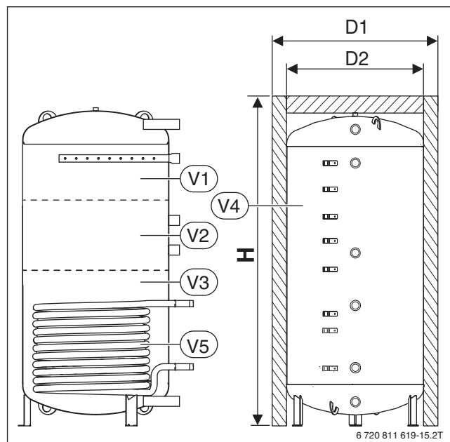
Bild 168 Maße und Volumina PSW 750/1000-5 S solar
