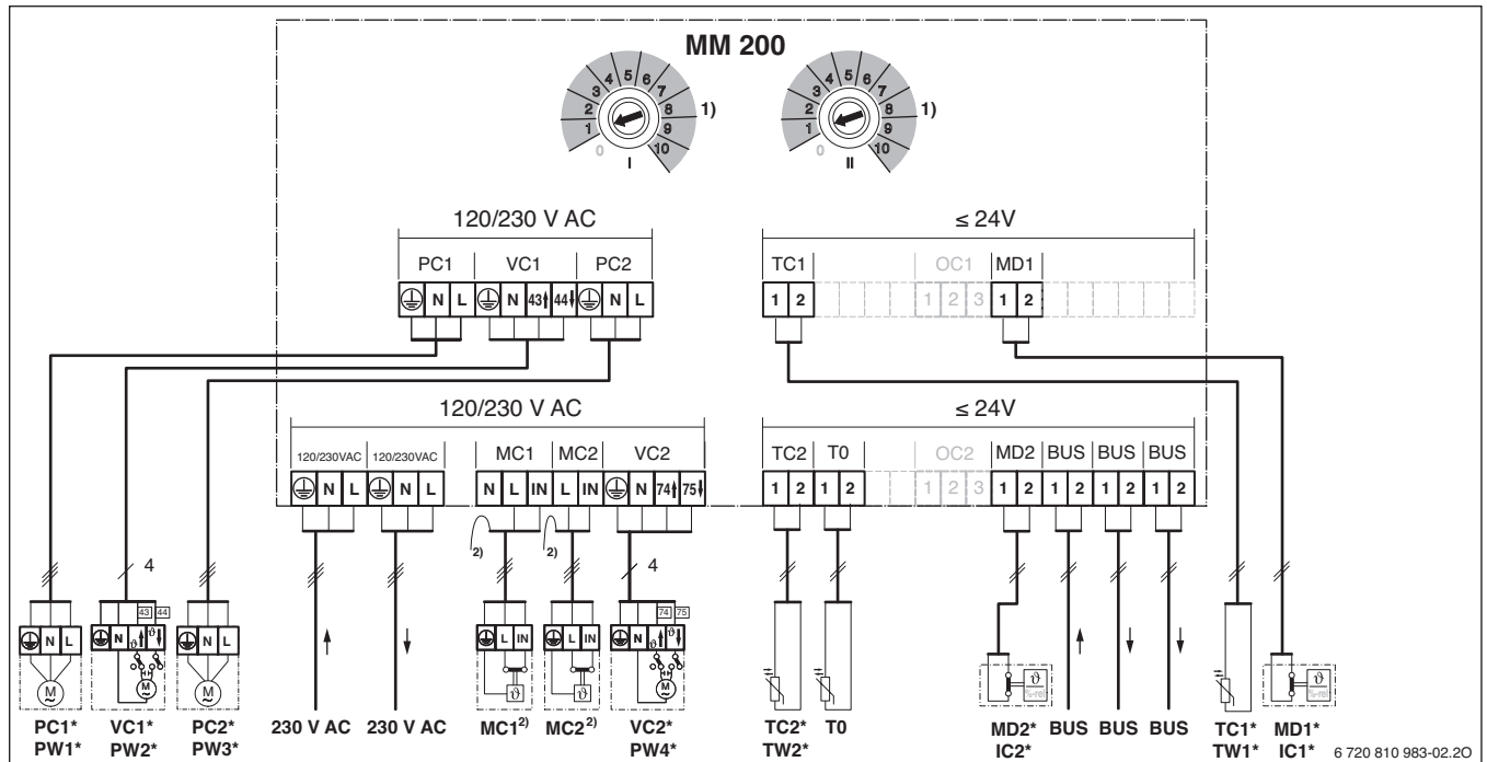
Bild 125 Anschlussplan des Heizkreismoduls MM200
