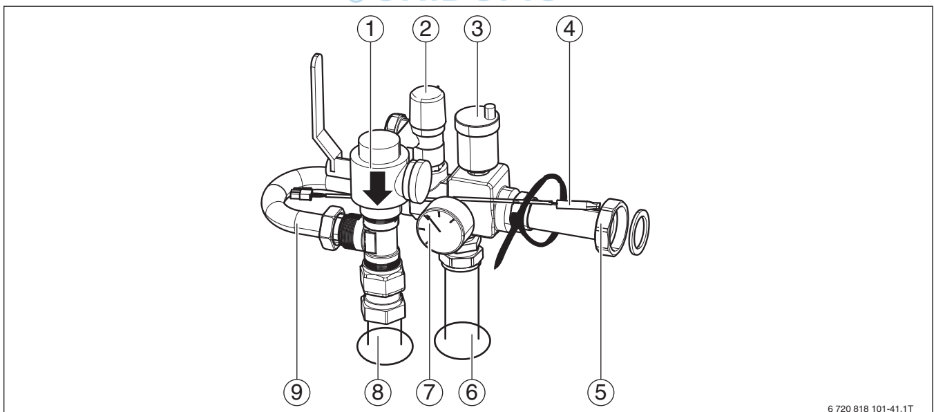
Bild 82 Montierte Sicherheitsgruppe
