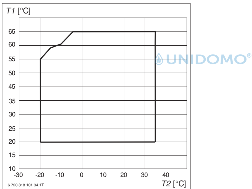
Bild 98 Wärmepumpe SAO ...-2 HT ohne Zuheizer
