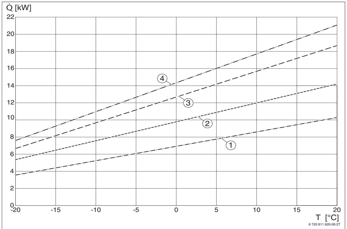
Bild 24 Bivalenztemperatur, Heizleistungskurve der Wärmepumpen SAO ...-2 bei 45 °C Vorlauftemperatur (schematische Darstellung)
