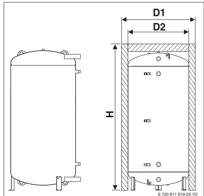
Bild 165 Maße PSW 500-5
