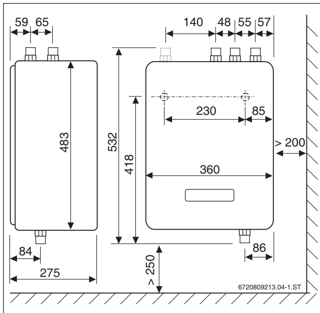
Bild 169 Abmessungen Frischwasserstation (in mm)
