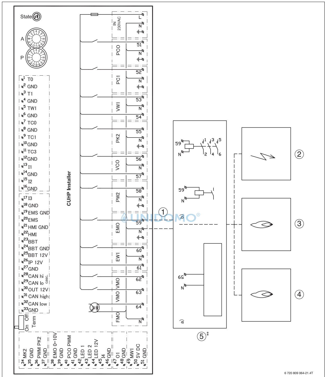
Bild 117 Schaltplan Installationsmodul, Start/Stopp
