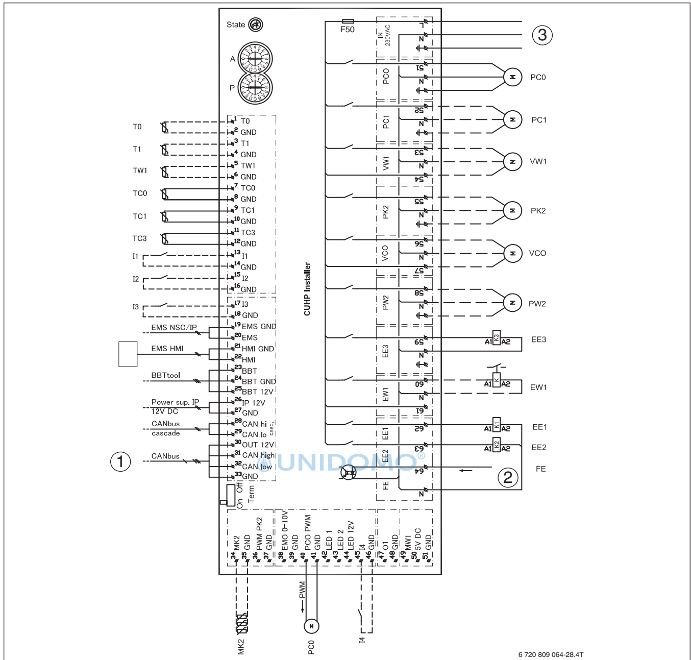
Bild 101 Schaltplan Installationsmodul
