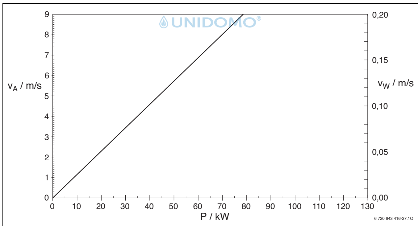
Bild 30 Diagramm Strömungsgeschwindigkeit HW 50, Anschluss 1½" bei \Delta T = 15 \text{ K } (T_V - T_R)
