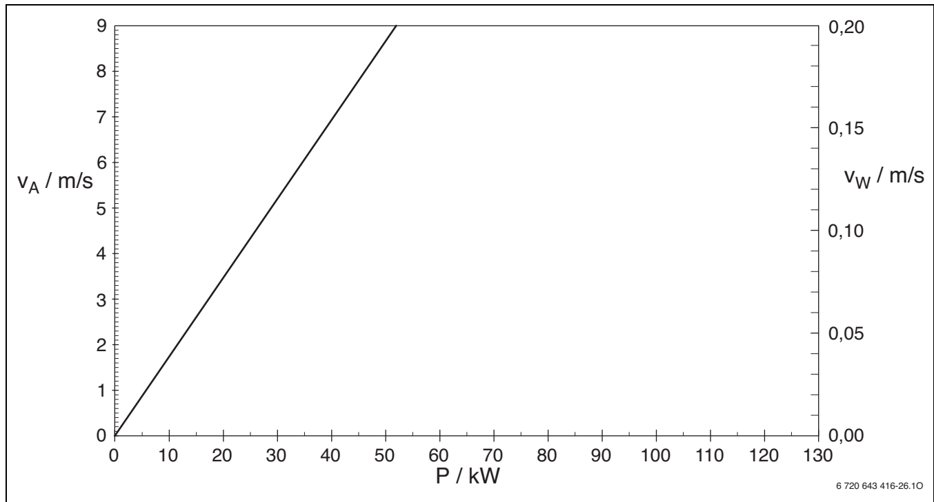
Bild 29 Diagramm Strömungsgeschwindigkeit HW 50, Anschluss 1½" bei \Delta T = 10 \text{ K } (T_V - T_R)
