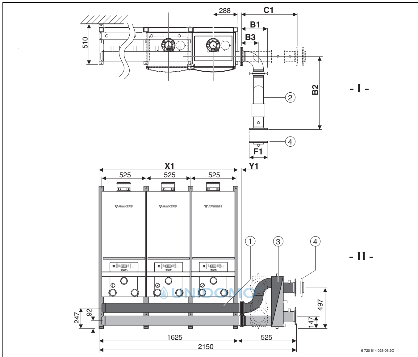
Bild 25 Maße Anschluss-Set
