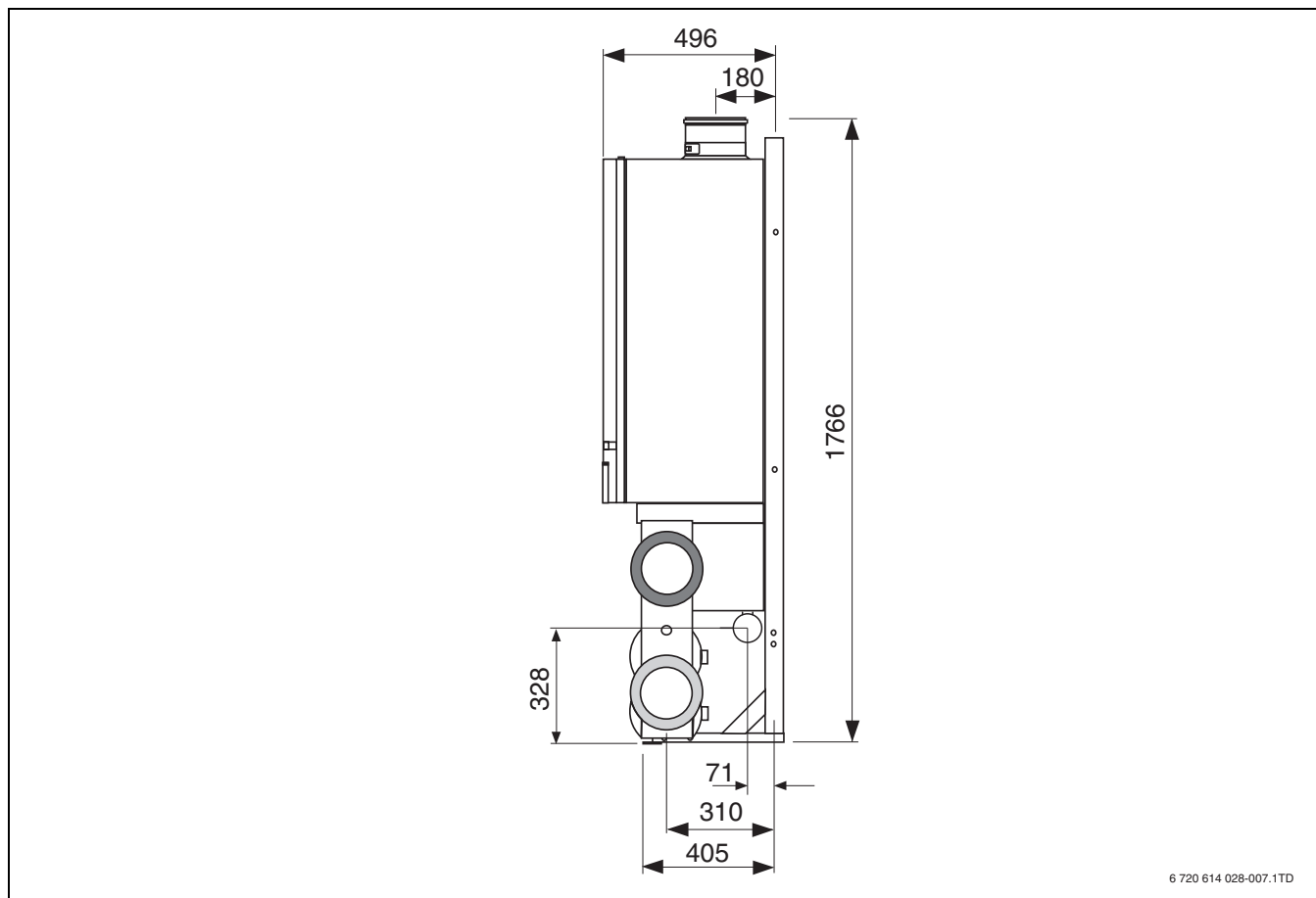
Bild 26 Maße Anschluss-Set (Seitenansicht)
