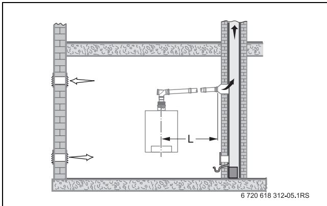
Bild 42 B 33 : Einzelführung an einem FU-Schornstein
