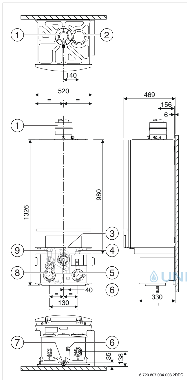
Bild 10 Abmessungen [mm]
