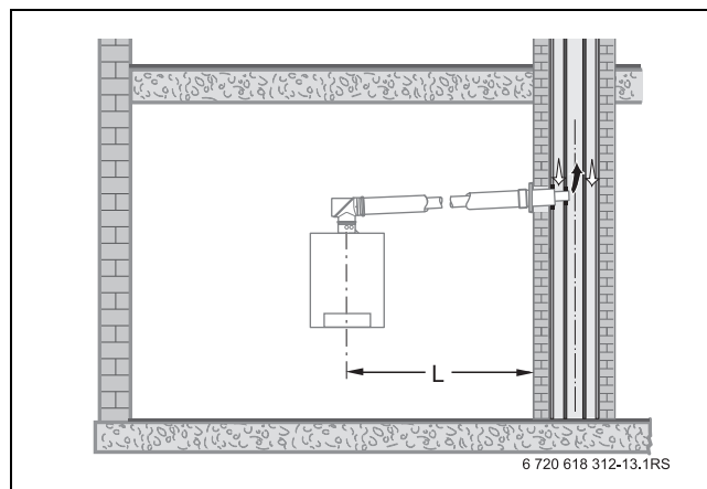
Bild 49 C 43x : Luft-/Abgasführung über mehrfach belegtes LAS in getrennten Schächten
