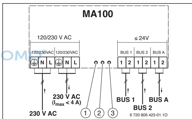
Bild 82 Anschlussplan BUS-Verstärkungsmodul MA 100
