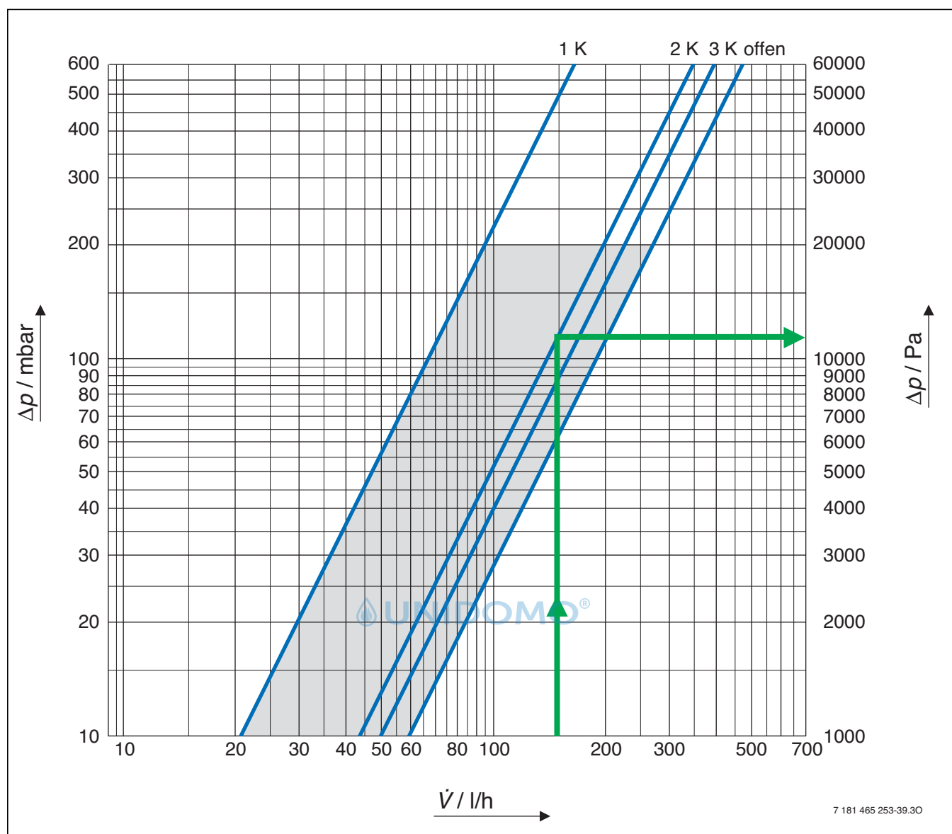
Bild 46 Durchflussdiagramm für Universalventile
