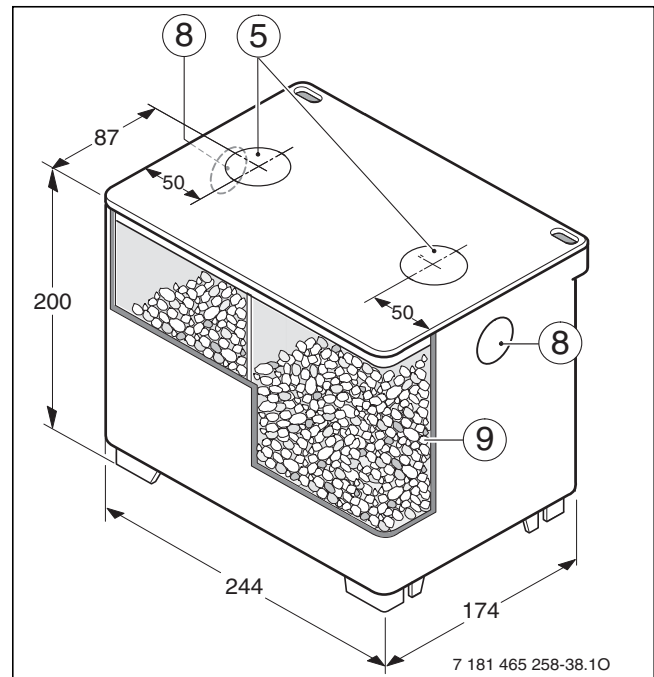
Bild 17 Neutralisationseinrichtung
