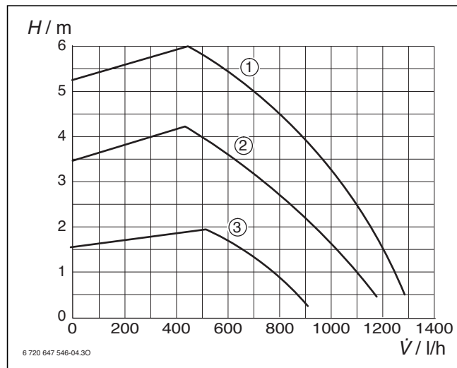
Bild 12 Konstantdruckbetrieb
