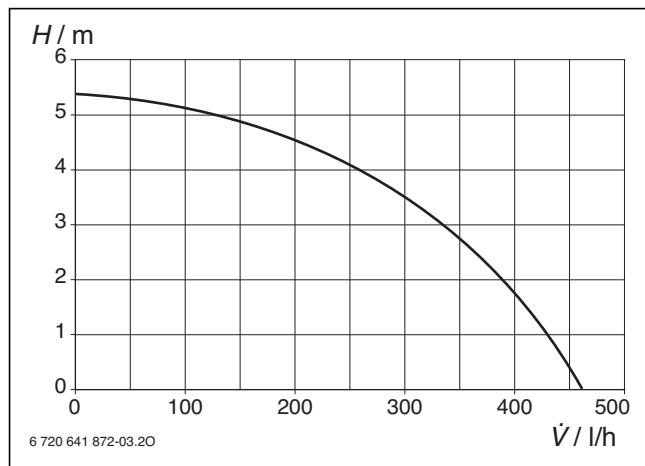
Bild 16 Kondensatpumpendiagramm: Förderhöhe über Volumenstrom
