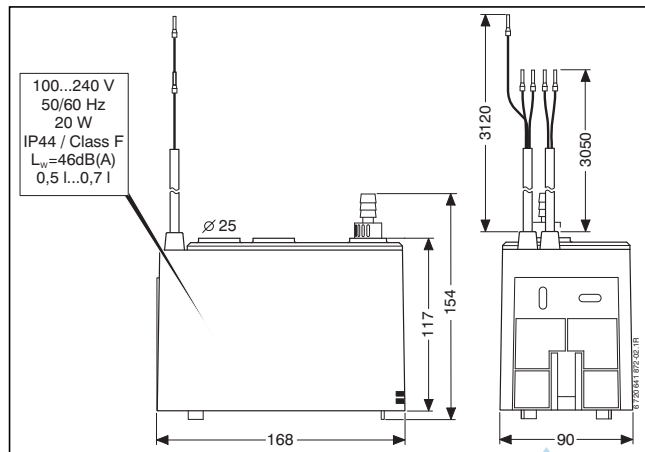
Bild 15 Kondensatpumpe
