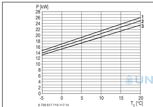
Bild 42 Leistungsdiagramm STE 170-1
