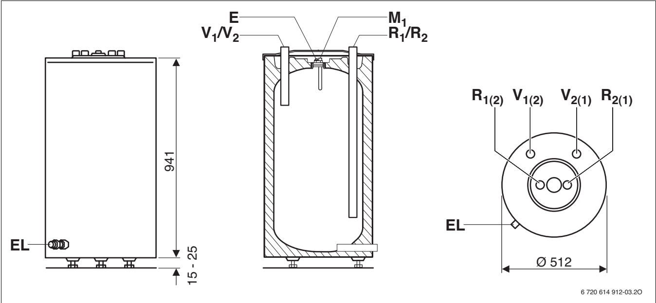
Bild 75 Bau- und Anschlussmaße Pufferspeicher PSW 120 (Maße in mm)
