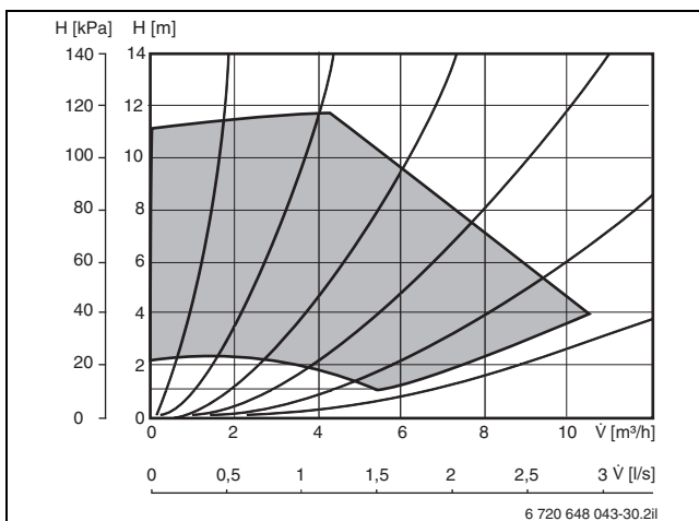
Bild 27 Pumpenkenlinie Solepumpe STM 100-1
