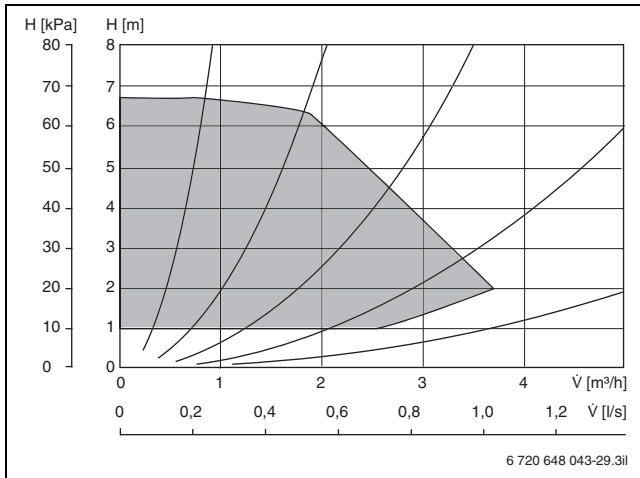
Bild 25 Pumpenkenlinie Solepumpe STM 60-1
