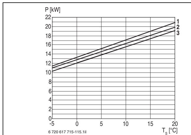
Bild 40 Leistungsdiagramm STE 130-1
