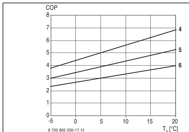
Bild 20 Leistungszahl STM 60-1
