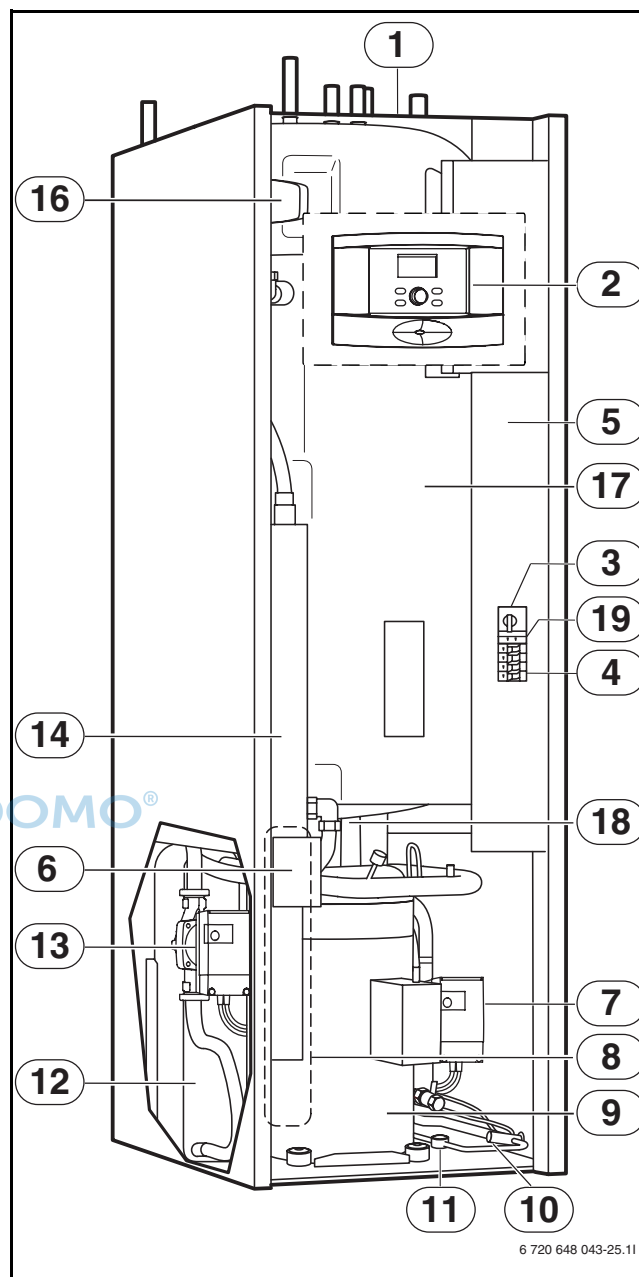
Bild 16 Ausgewählte Bauteile und Baugruppen STM 60-1 ... STM 100-1
