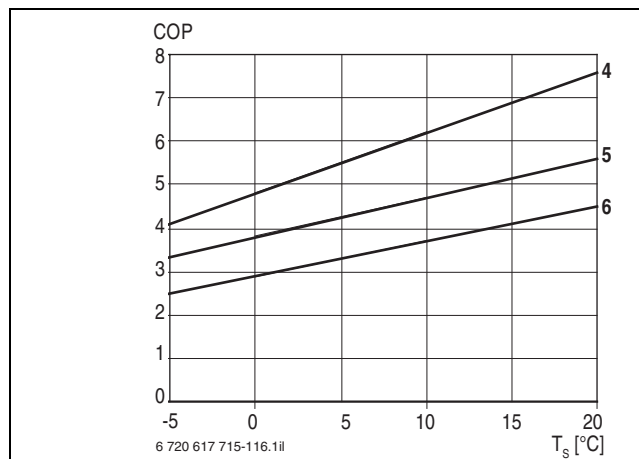
Bild 41 Leistungszahl STE 130-1
