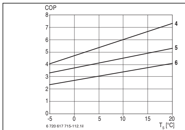
Bild 24 Leistungszahl STM 100-1
