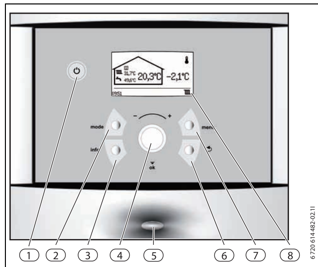
Bild 62 Bedienfeld
