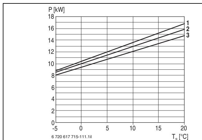
Bild 23 Leistungsdiagramm STM 100-1
