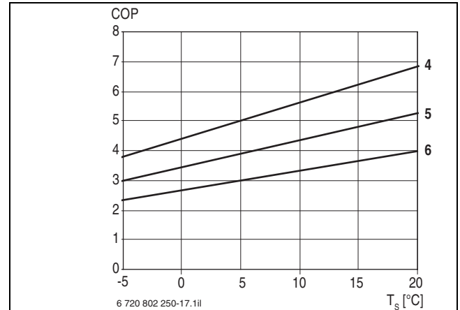
Bild 35 Leistungszahl STE 60-1
