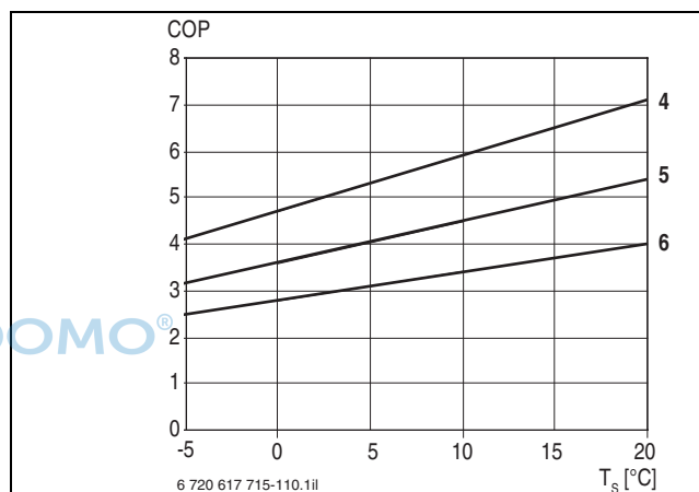
Bild 22 Leistungszahl STM 80-1
