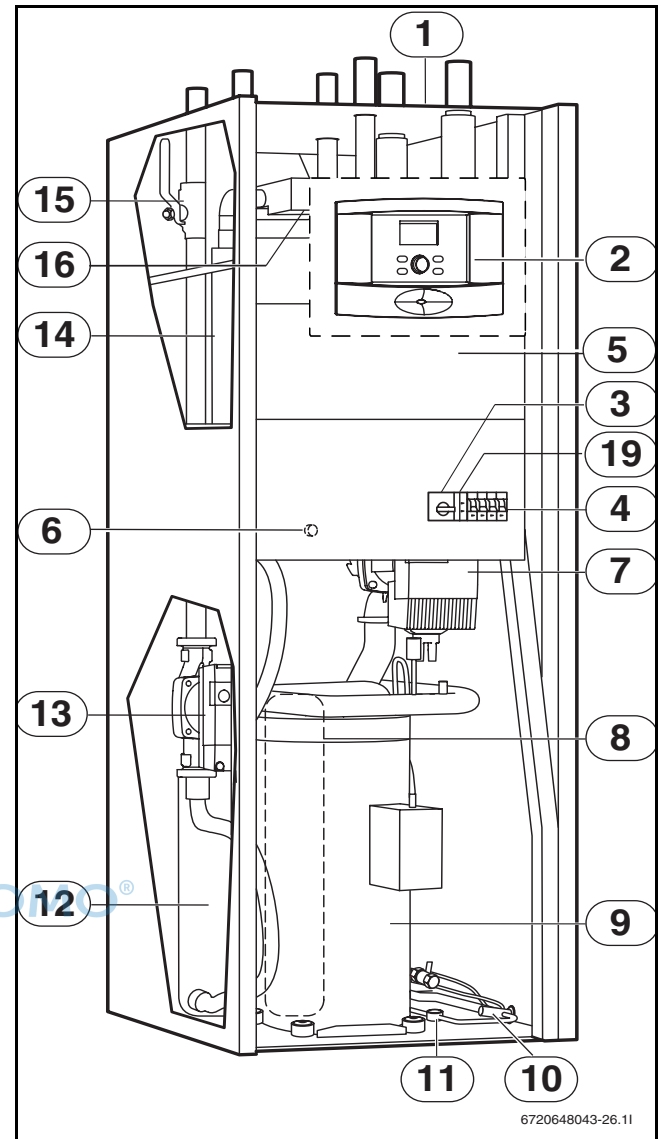
Bild 30 Ausgewählte Bauteile und Baugruppen STE 60-1 ... STE 170-1
