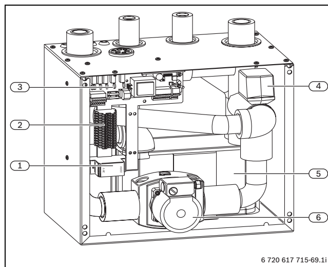
Bild 80 Aufbau natürliche Kühlstation NKS-1
