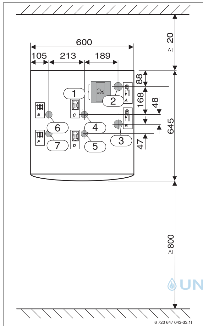
Bild 31 Abmessungen der Wärmepumpen STE 60-1 ... STE 80-1 (Maße in mm)
