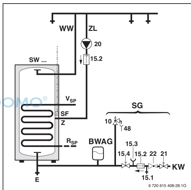
Bild 65 Trinkwasserseitiges Anschluss-Schema
