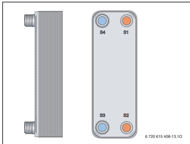
Bild 95 Plattenwärmeübertrager
