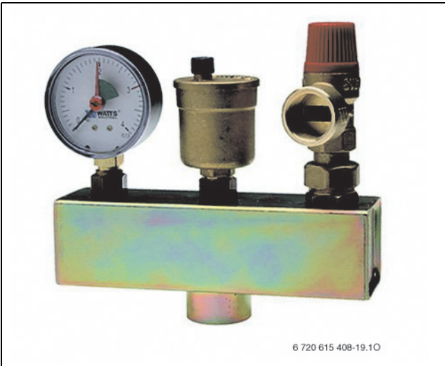
Bild 98 Sicherheitsgruppe KSG
