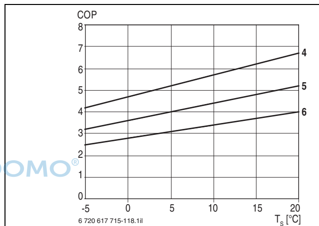
Bild 43 Leistungszahl STE 170-1
