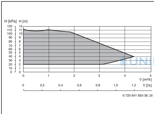
Bild 26 Pumpenkenlinie Solepumpe STM 80-1
