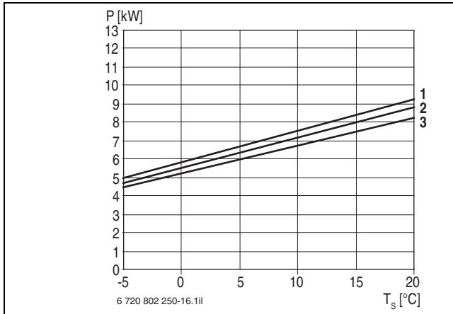
Bild 34 Leistungsdiagramm STE 60-1
