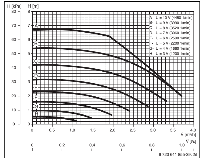
Bild 28 Pumpenkenlinie Heizungspumpe STM 60-1... STM 100-1
