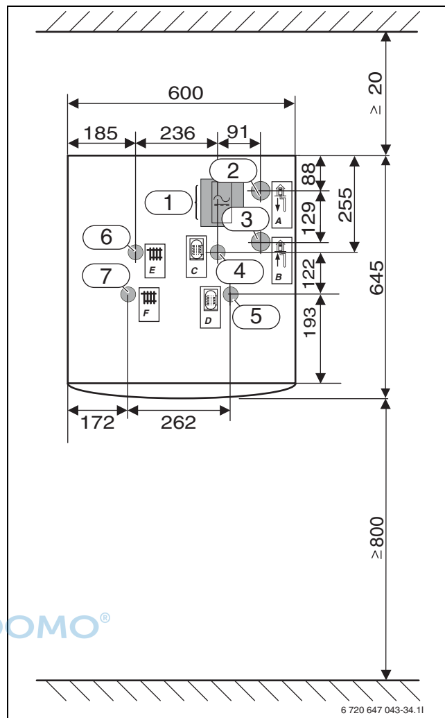
Bild 32 Abmessungen der Wärmepumpen STE 100-1 ... STE 170-1 (Maße in mm)
