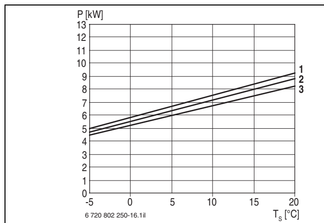
Bild 19 Leistungsdiagramm STM 60-1
