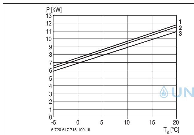
Bild 21 Leistungsdiagramm STM 80-1
