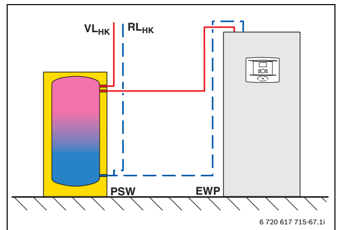
Bild 57 Gemeinsamer Anschluss mit T-Stück
