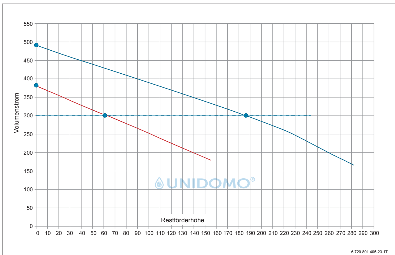
Bild 8 Kennlinie Luftvolumenstrom
