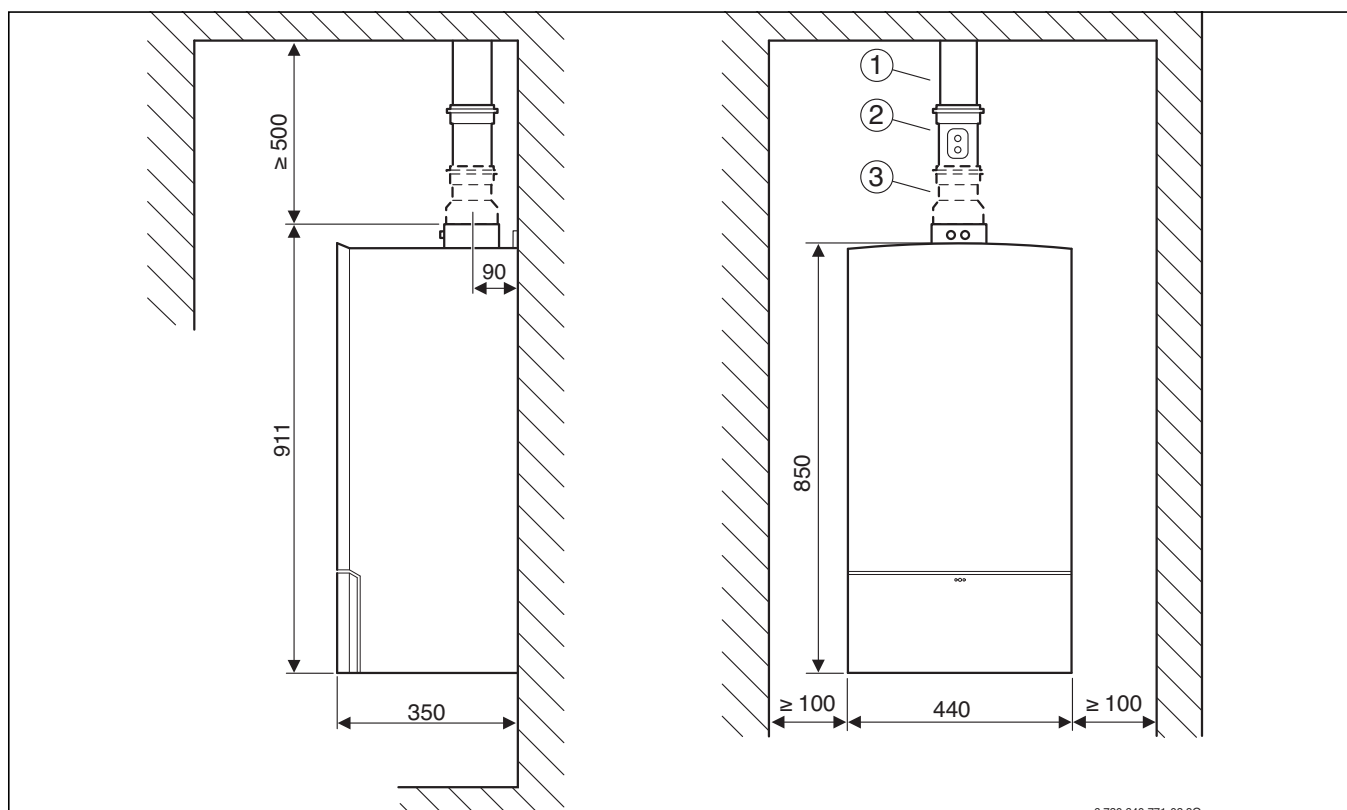
Bild 71 Flachdach
