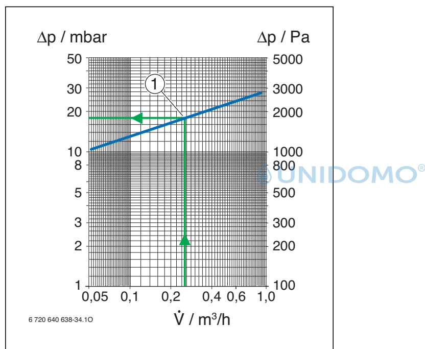
Bild 22 Druckverlust in der Heizschlange im Pufferspeicher P 400-5 SHU
