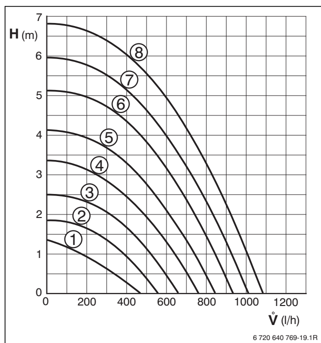
Bild 44 Pumpenkenlinien - Gerät mit Systempufferspeicher SP 400 SHU-2 und Anschluss-Set Zubehör Nr. 1463
