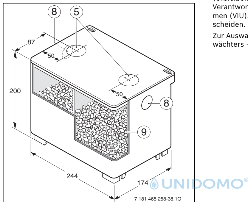
Bild 48 Neutralisationseinrichtung
