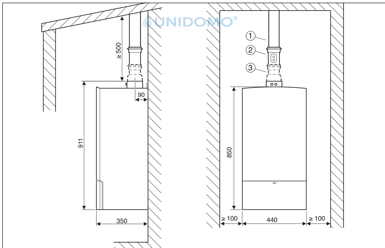
Bild 72 Schrägdach
