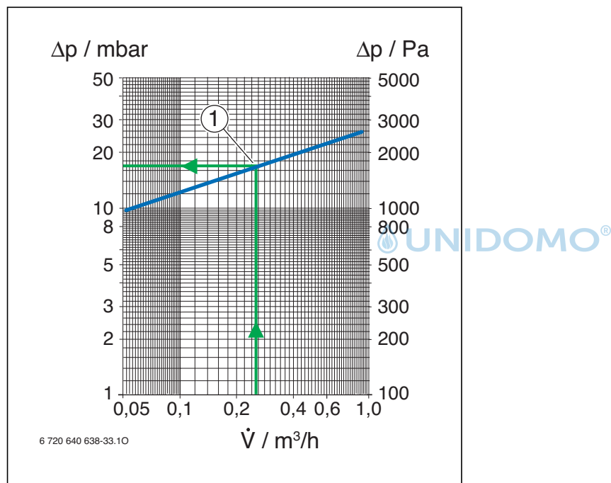
Bild 21 Druckverlust in der Heizschlange im Pufferspeicher P 290-5 SHU
