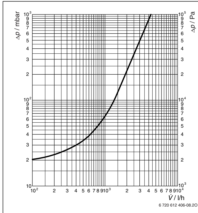
Bild 94 Druckverlust-Diagramm gemischter Heizkreise
