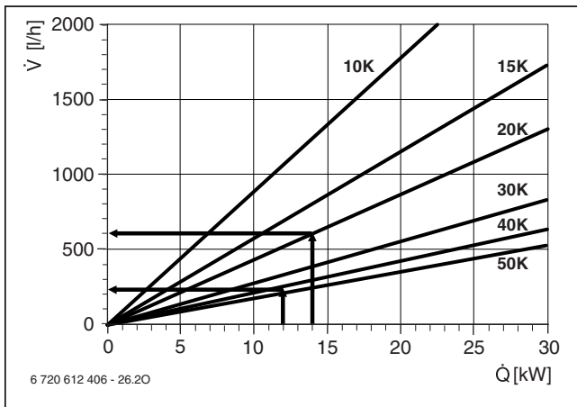
Bild 97 Volumenstrom Primärkreis
