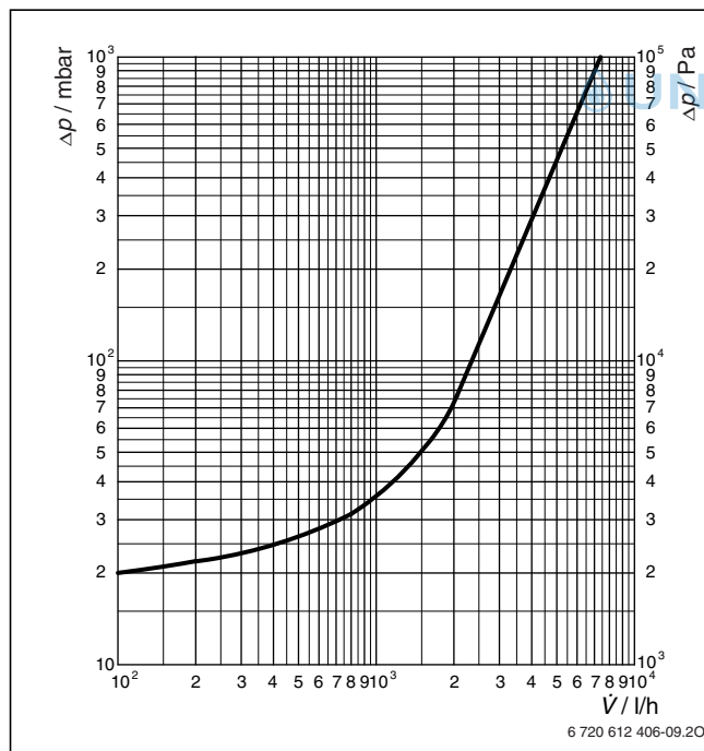
Bild 95 Druckverlust-Diagramm ungemischter Heizkreise
