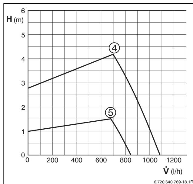
Bild 42 Proportionaldruck - Gerät mit Pufferspeicher SP 400 SHU-2 und Anschluss-Set Zubehör Nr. 1463
