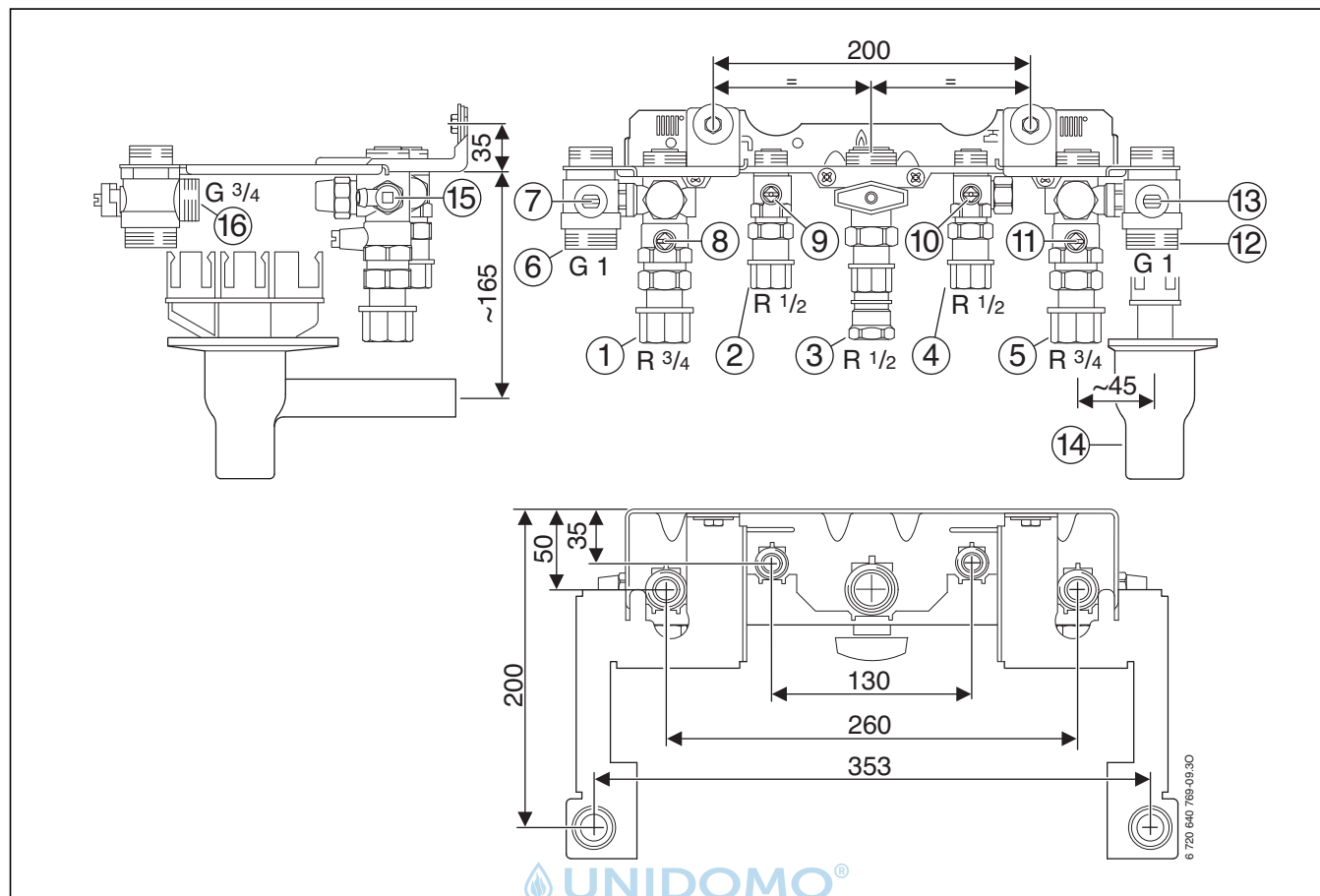
Bild 31 Montageanschlussplatte Nr. 1469
