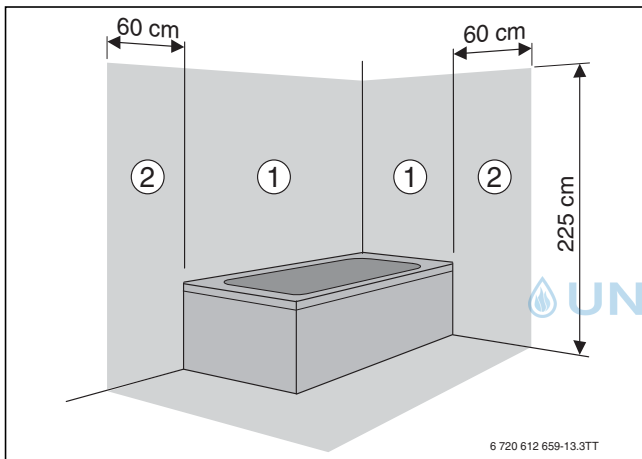
Bild 52 Schutzbereiche
