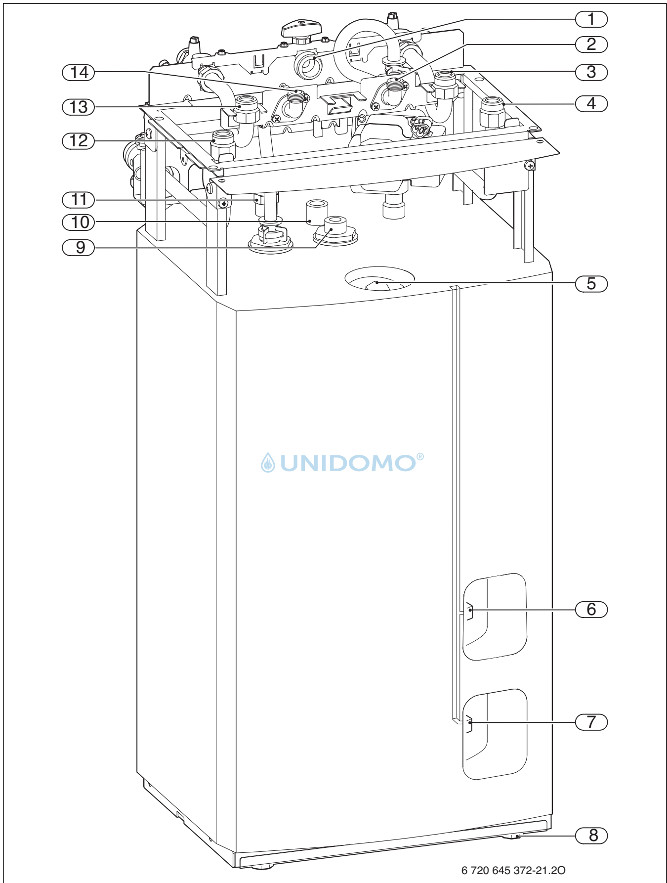
Bild 34 Schichtladespeicher
