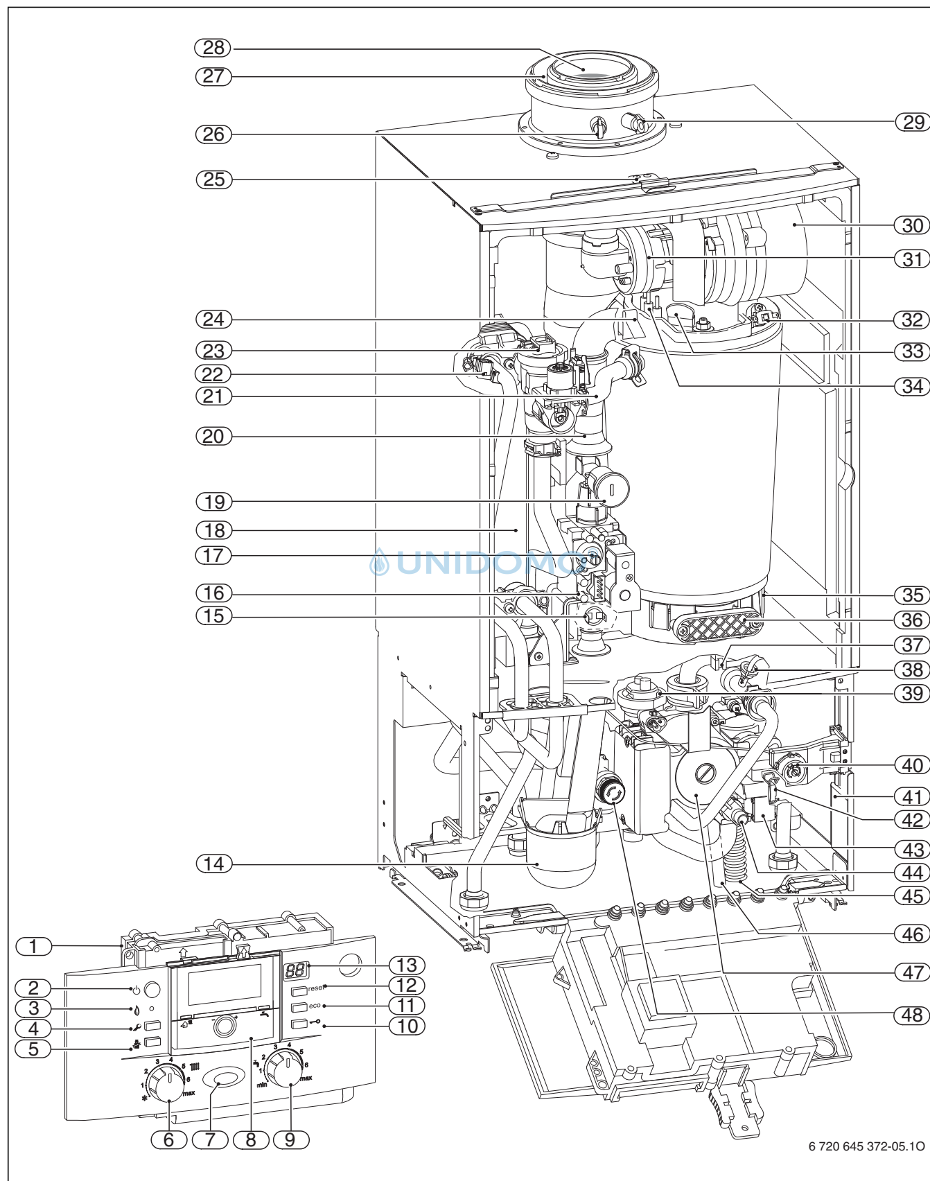
Bild 33 Gas-Brennwertgerät
