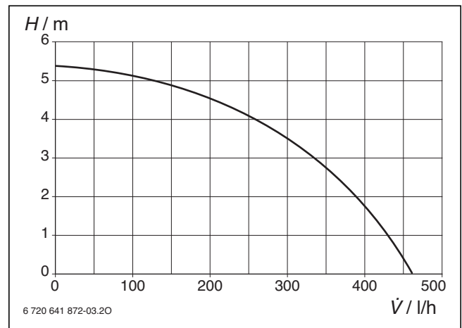
Bild 47 Kondensatpumpendiagramm: Förderhöhe über Volumenstrom
