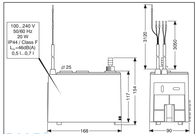
Bild 46 Kondensatpumpe
