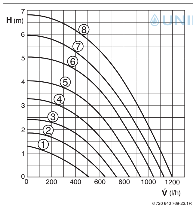
Bild 45 Pumpenkenlinien - Gerät ohne Systempufferspeicher und Verrohrung
