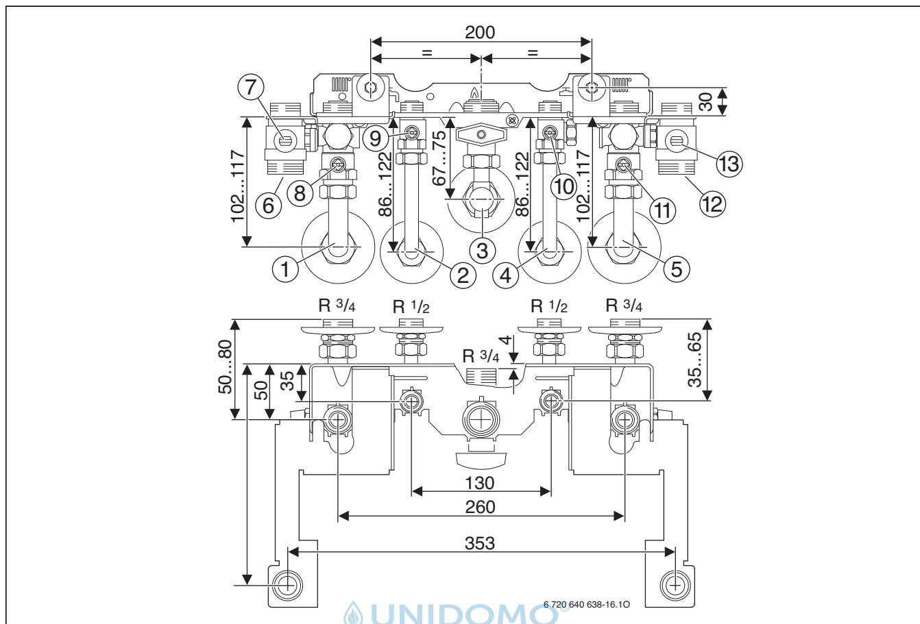
Bild 32 Montageanschlussplatte Nr. 1470
