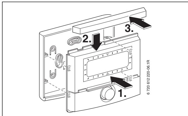
Bild 59 Wandinstallation
