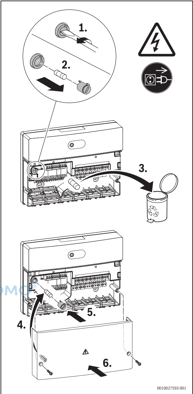
Bild 34 Sicherung tauschen
