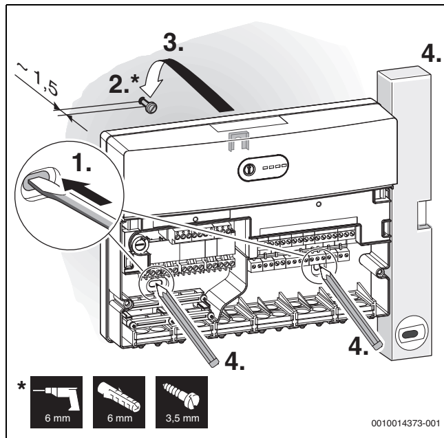
Bild 21 Wandbefestigung anzeichnen
