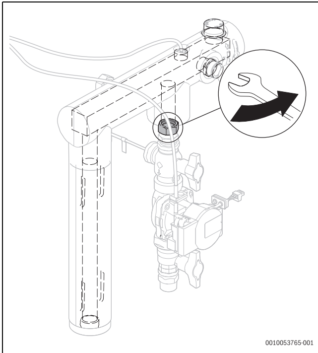
Bild 6 Lösen der Überwurfmutter
