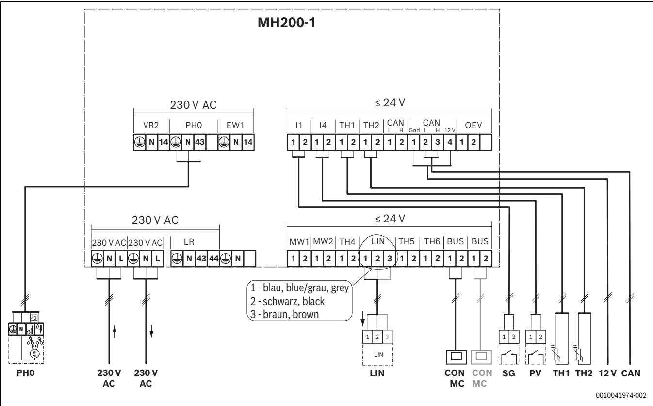
Bild 4 Überblick Anschlussklemmenbelegung
