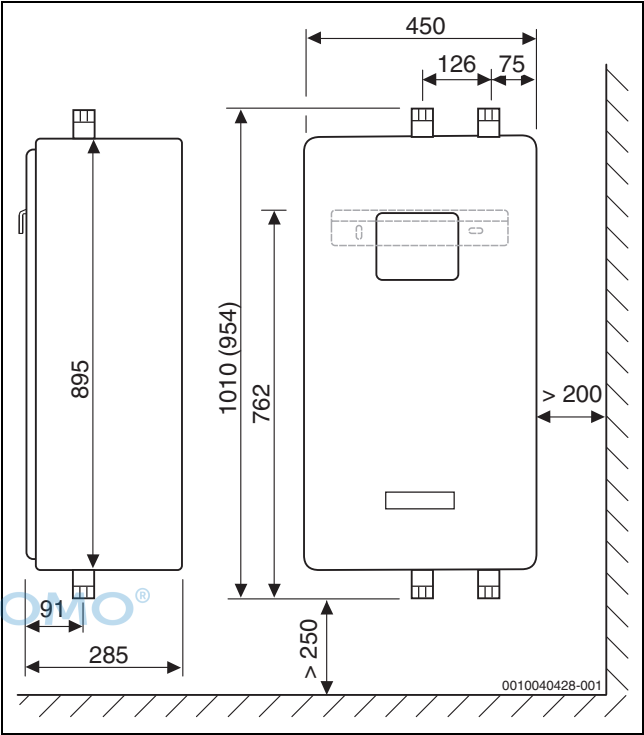
Bild 16 Abmessungen und Mindestabstände, Maße in mm (Wert in Klammern = TS 2-3 S)
