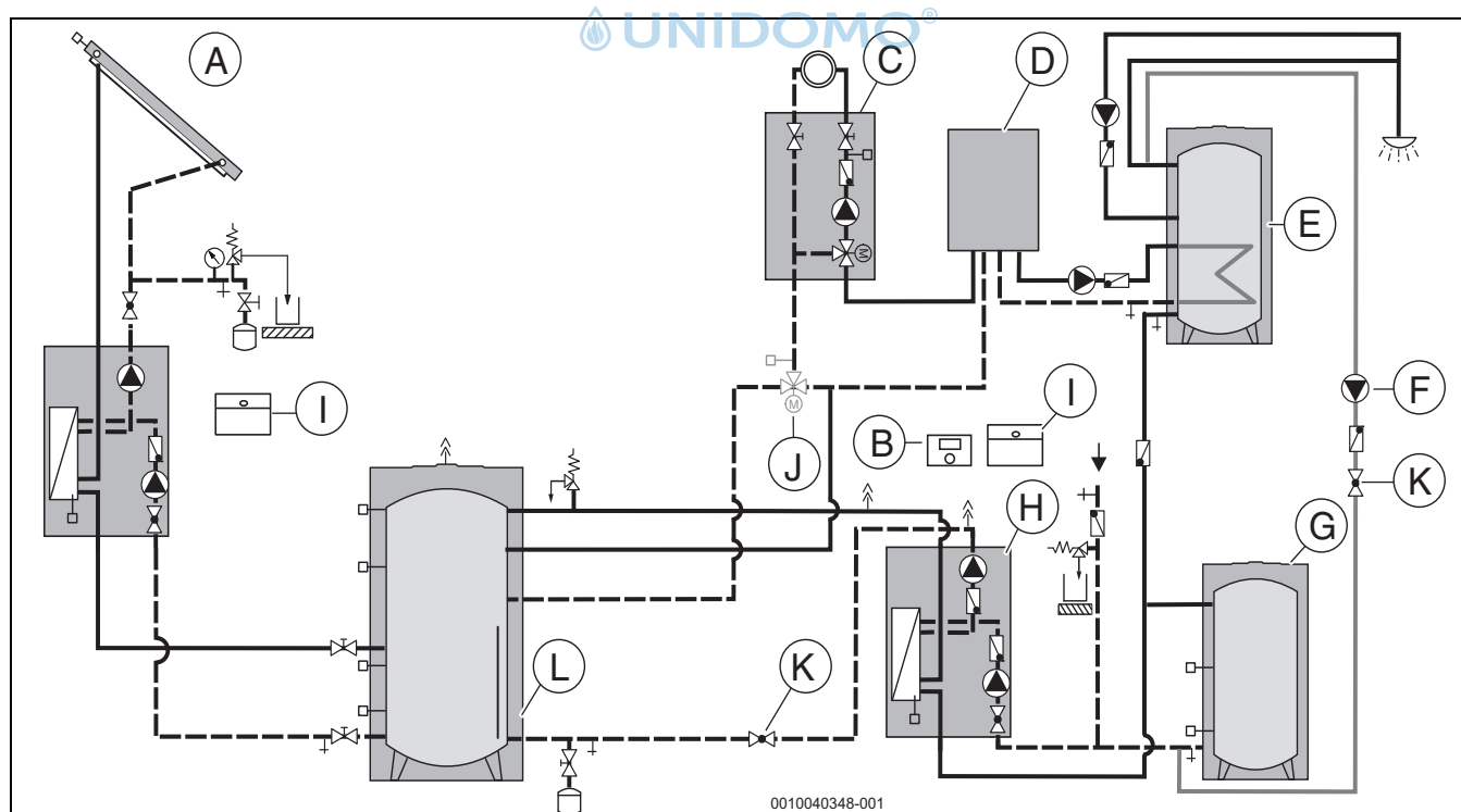
Bild 10 Anlagenbeispiel mit Optionen: Vorwärmstufe mit Umladebetrieb von Pufferspeicher auf Vorwärm Speicher (diese schematische Darstellung gibt keinen Hinweis auf eine mögliche Ausführung vor Ort)
