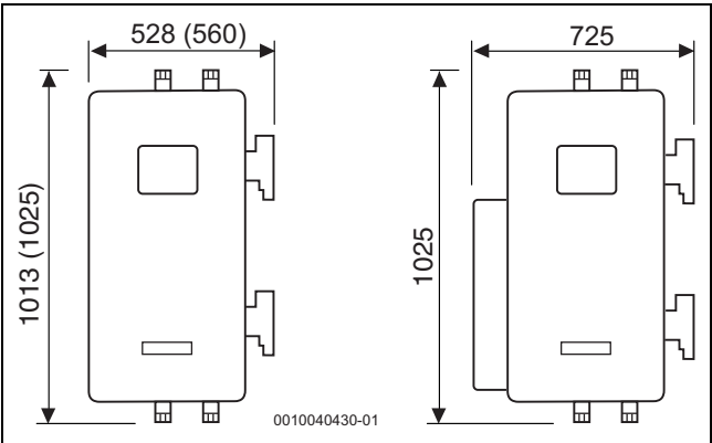
Bild 17 Links: TS 3-3 S und TS 4-3 S (Wert in Klammern = TS 4-3 S), rechts: TS 5-3 S
