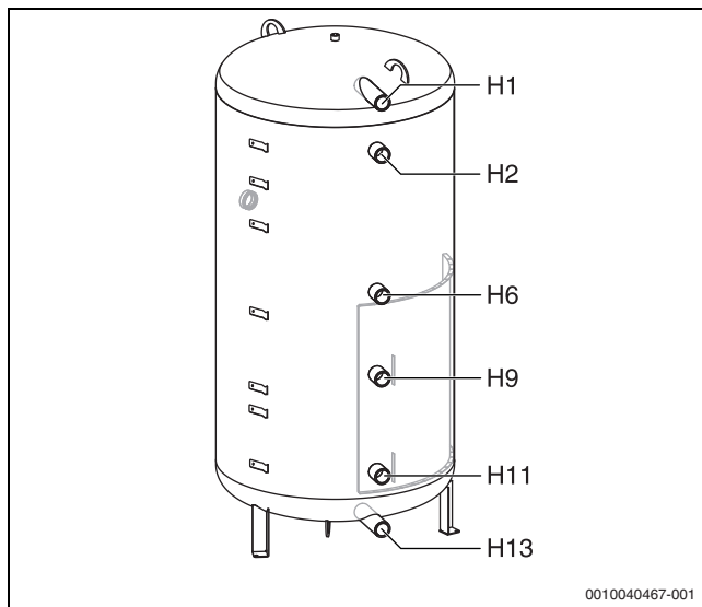
Bild 33 Pufferspeicher (→ Bild 10, Seite 6)
