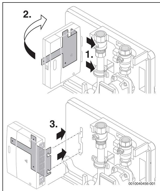
Bild 25 Modul in Arbeitsposition bringen
