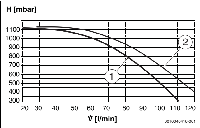
Bild 13 Restförderhöhe
