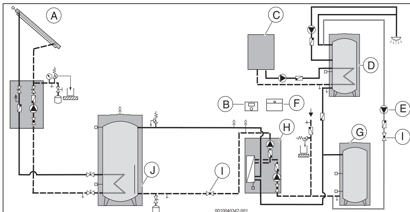
Bild 9 Anlagenbeispiel Standard: Vorwärmstufe mit Umladebetrieb von Pufferspeicher auf Vorwärm Speicher (diese schematische Darstellung gibt keinen Hinweis auf eine mögliche Ausführung vor Ort)
