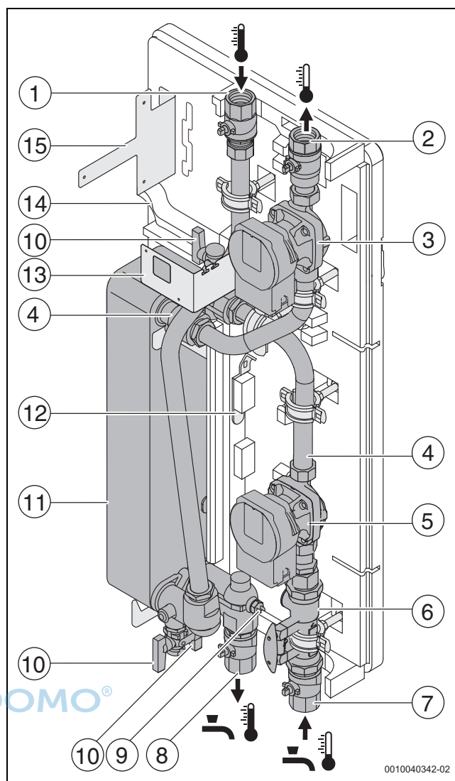
Bild 4 Station TS 1-3 S ohne vorderen Wärmeschutz
