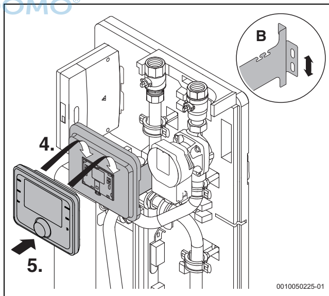
Bild 28 Bedieneinheit montieren
