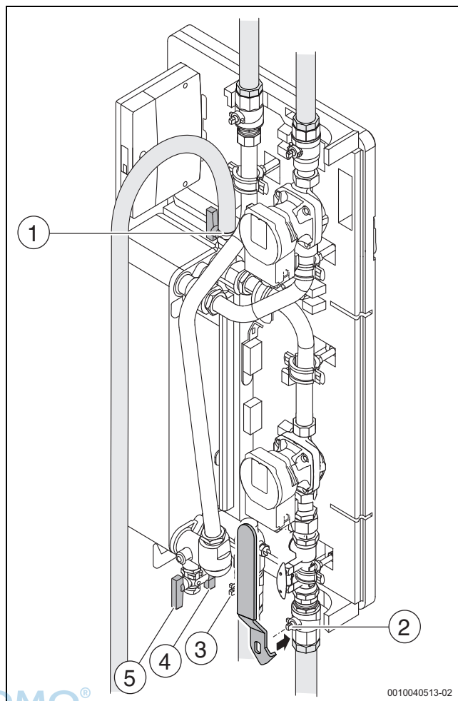
Bild 37 Wärmetauscher reinigen
