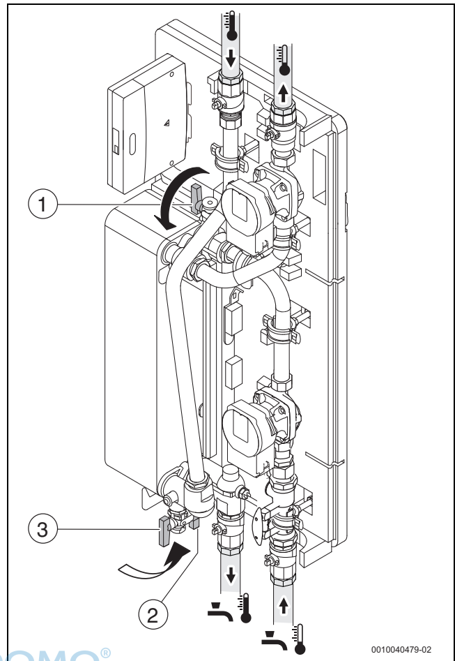
Bild 34 Anlage füllen
