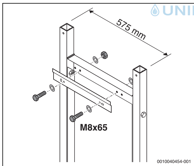
Bild 23 Wandhalter montieren
