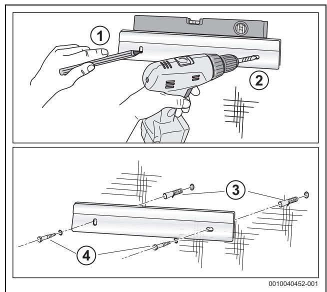
Bild 21 Wandhalter montieren
