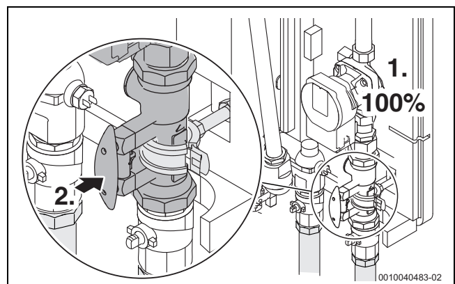
Bild 35 Durchflussbegrenzer Sekundärseite
